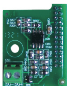
FCI-RS485
