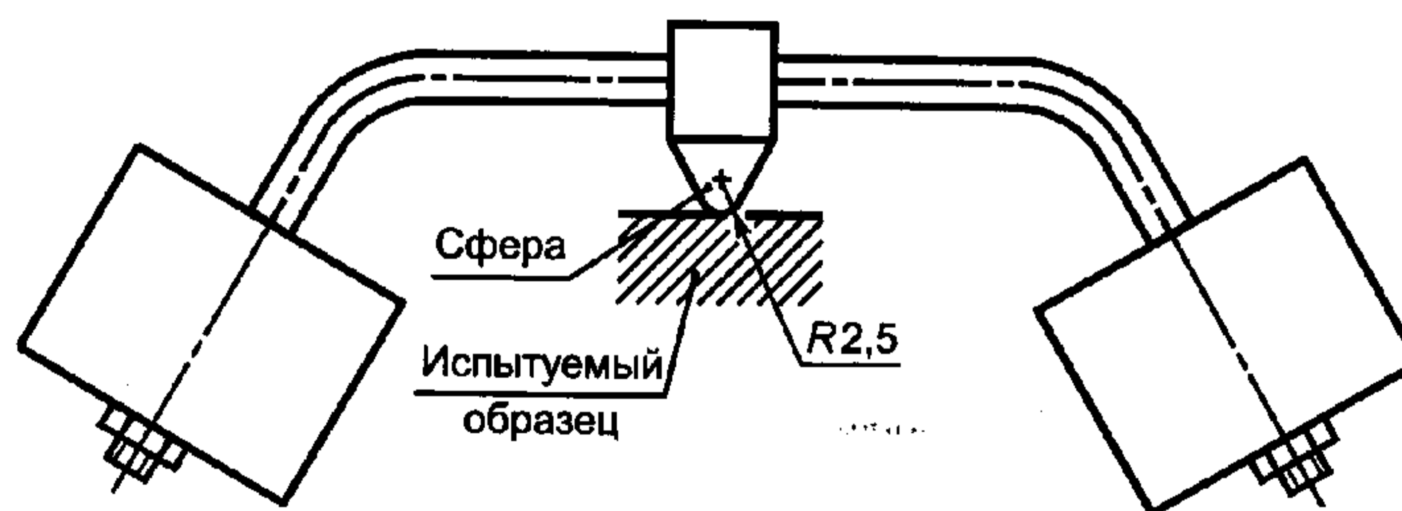
Рисунок 1 – Установка для испытания на теплостойкость
