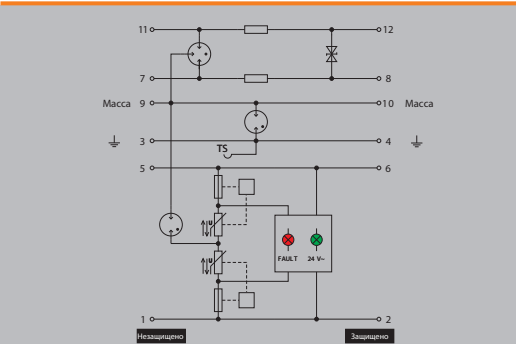
Комплектный модуль, не прямое заземления
