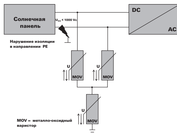
Рис. 4: Y-образная защитная схема с тремя варисторами
