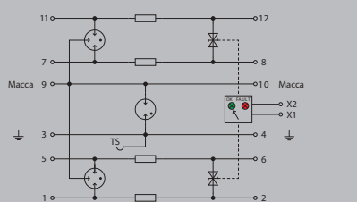
Комплектный модуль, не прямое заземление, с дистанц. оповещением
