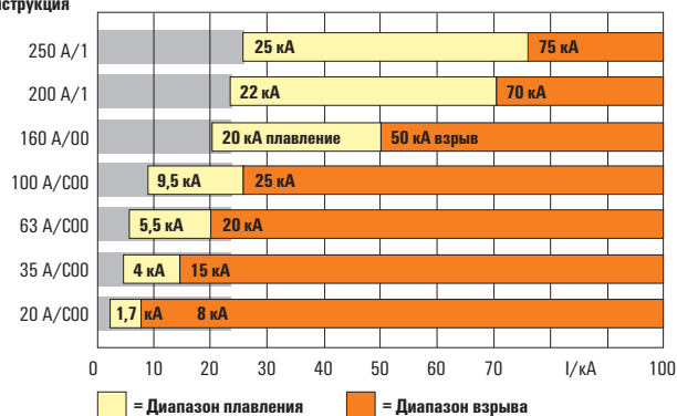
Номинальный ток и конструкция
