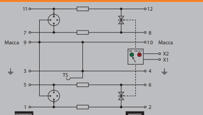
Комплектный модуль, прямое заземление, с дистанц. оповещением
