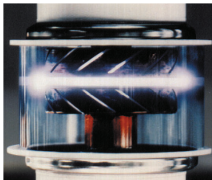
Дуговой разряд в выключателе 10 кВ при выключении
