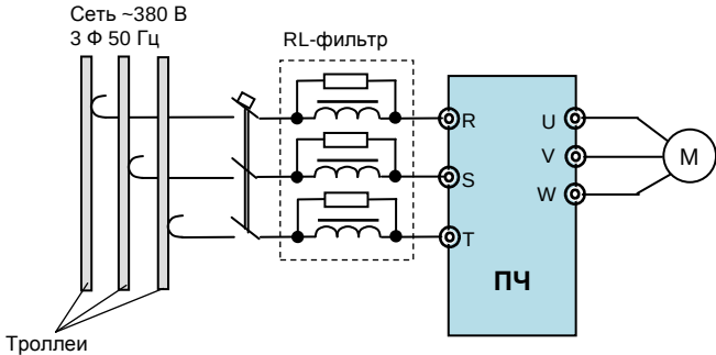
Схема подключения входного RL-фильтра при троллейном питании
