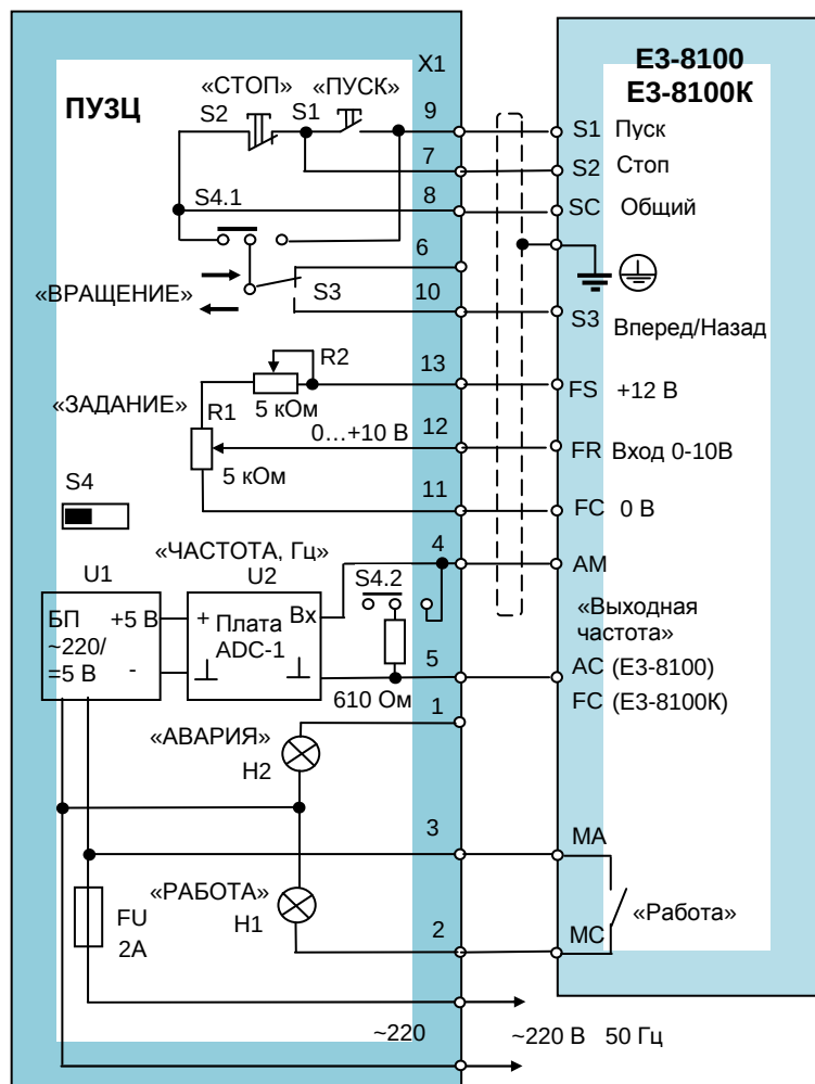
Подключение пульта ПУЗЦ к преобразователю ЕЗ-8100, (ЕЗ-8100К)
