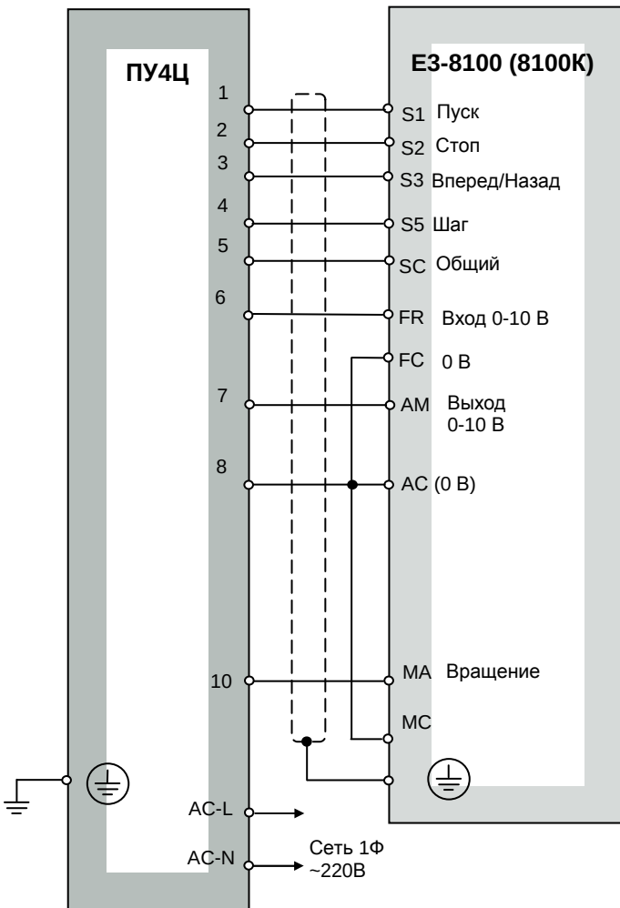
Подключение пульта ПУ4Ц к преобразователю ЕЗ-8100 (8100К)
