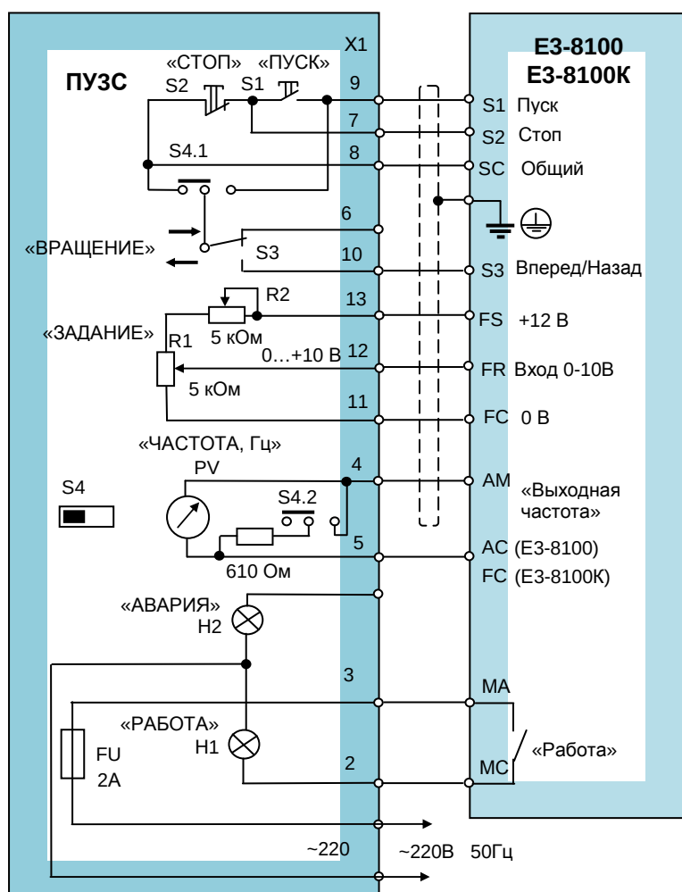
Подключение пульта ПУЗС к преобразователю ЕЗ-8100, (ЕЗ-8100К)
