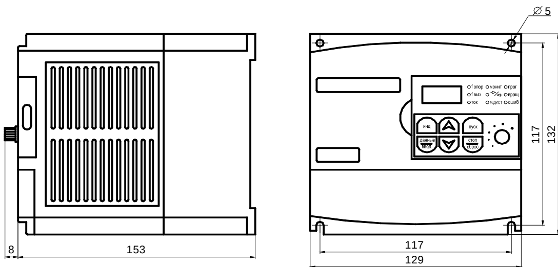
Преобразователь ЕЗ-8100-001Н
