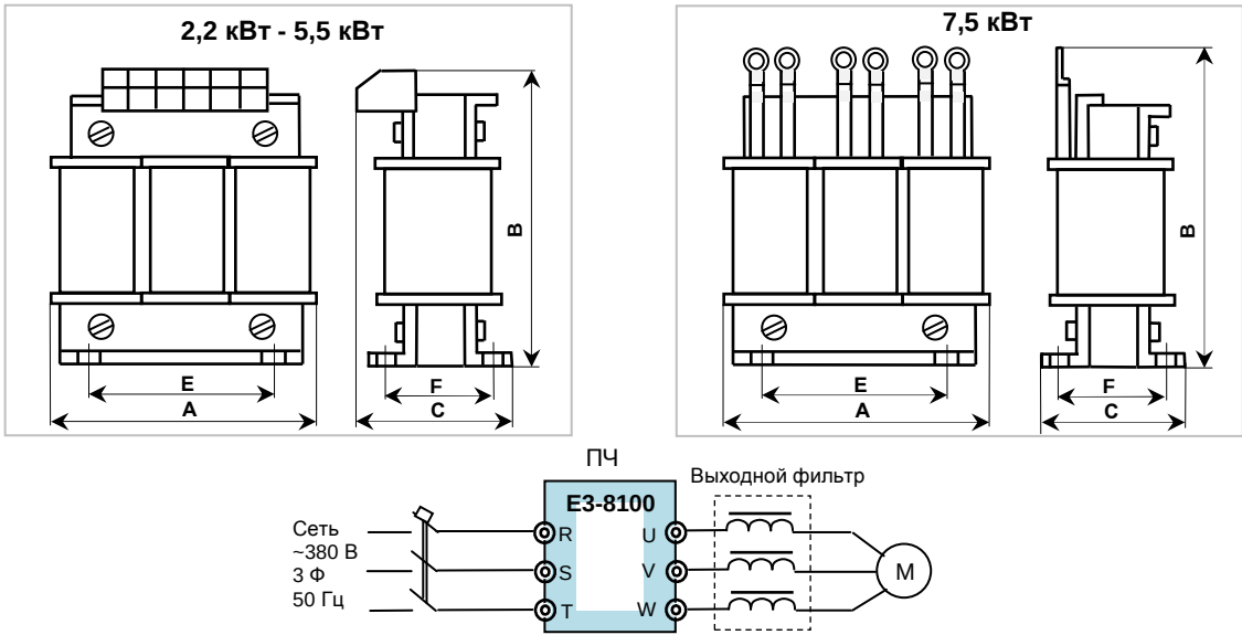
Схема включения выходного фильтра
