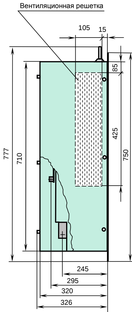
Вид справа
