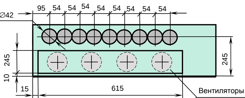
Вид снизу
