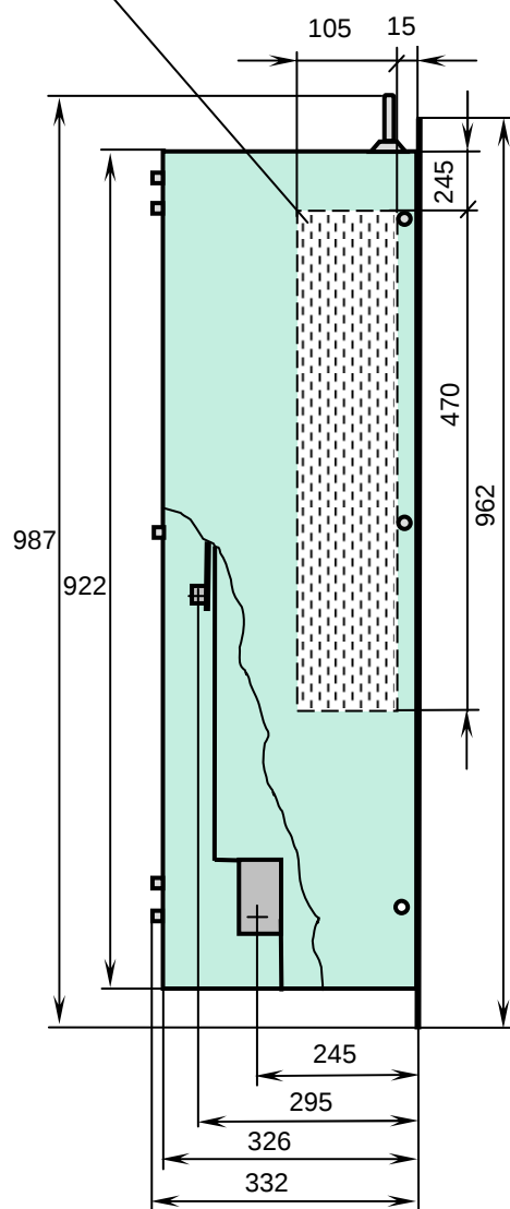
Вид справа
