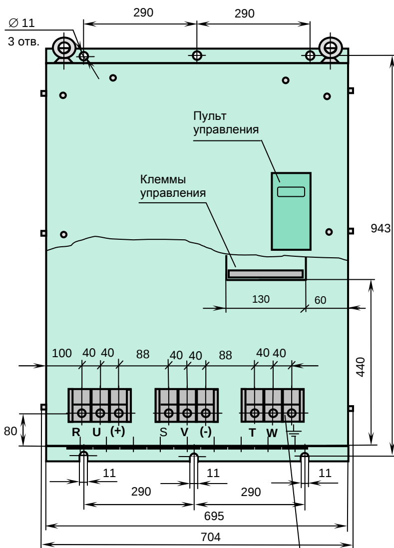
Силовые клеммы
