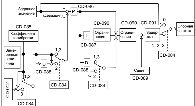
Схема ПИД-регулирования
