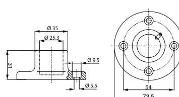
Цоколь для трубки, металл
