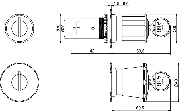
CE3K1/CE4K1
