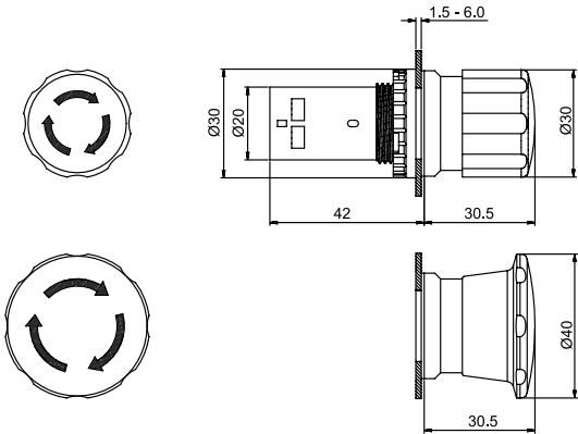
CE3T/CE4T (отпускание поворачиванием)
