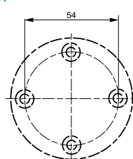
Схема сверления отверстий для сигнальных стоек K70
