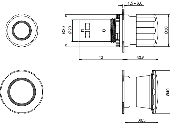
Кнопки аварийной остановки CE3P/CE4P (отпускание вытягиванием)
