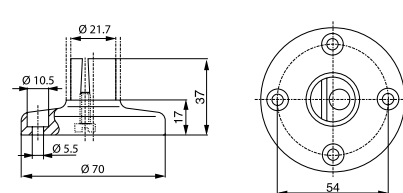
Цоколь для трубки, пластик
