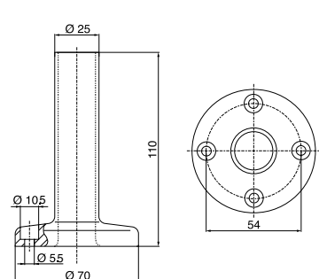
Цоколь для трубки, пластик
