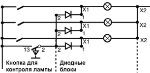
Схема контроля ламп с тремя диодными блоками (не предназначена для светодиодных блоков со встроенными светодиодами)
