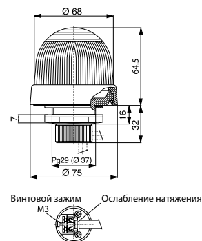
Сигнальные маяки KSB
