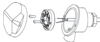
Установка НПТ-3 в датчик
