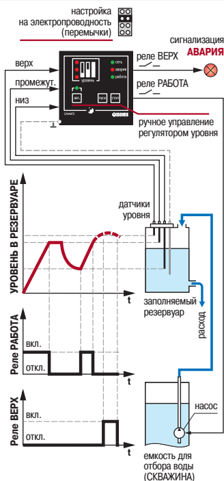
Режим заполнения резервуара
