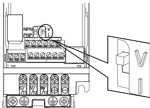
Рисунок 4.4.2. DIP-переключатель A1
