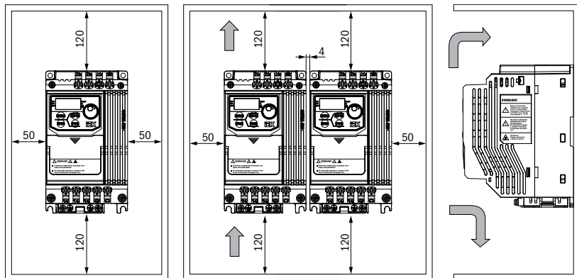
Рисунок 3.2. Установка преобразователей
