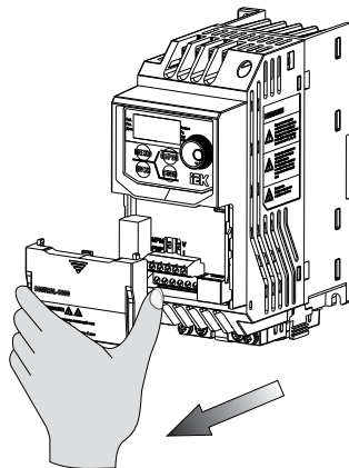
Шаг 2: снимите крышку клеммной колодки
