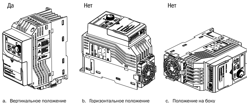
Рисунок 3.1. Установка преобразователя
