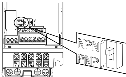
Рисунок 4.4.1. DIP-переключатель режимов NPN/PNP
