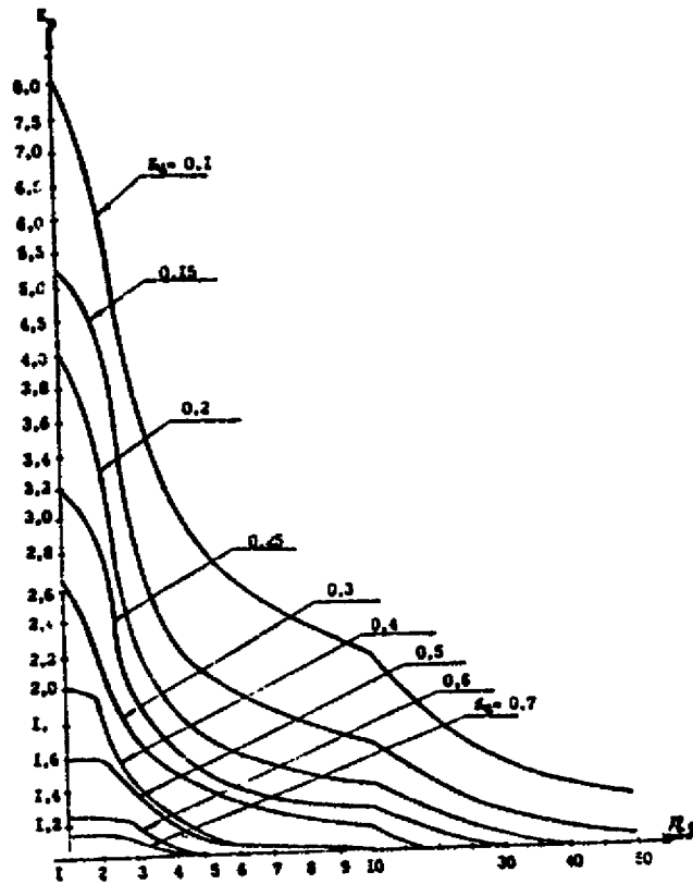
Кривые коэффициента расчетных нагрузок K_p для различных коэффициентов использования K_u в зависимости от n_3 (для постоянной времени нагрева T_o = 10 мин)
