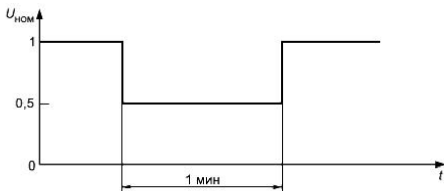
Рисунок В.3 - Провалы напряжения \Delta U = 50\%
