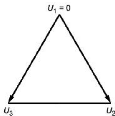
Состояние замыкания на землю
