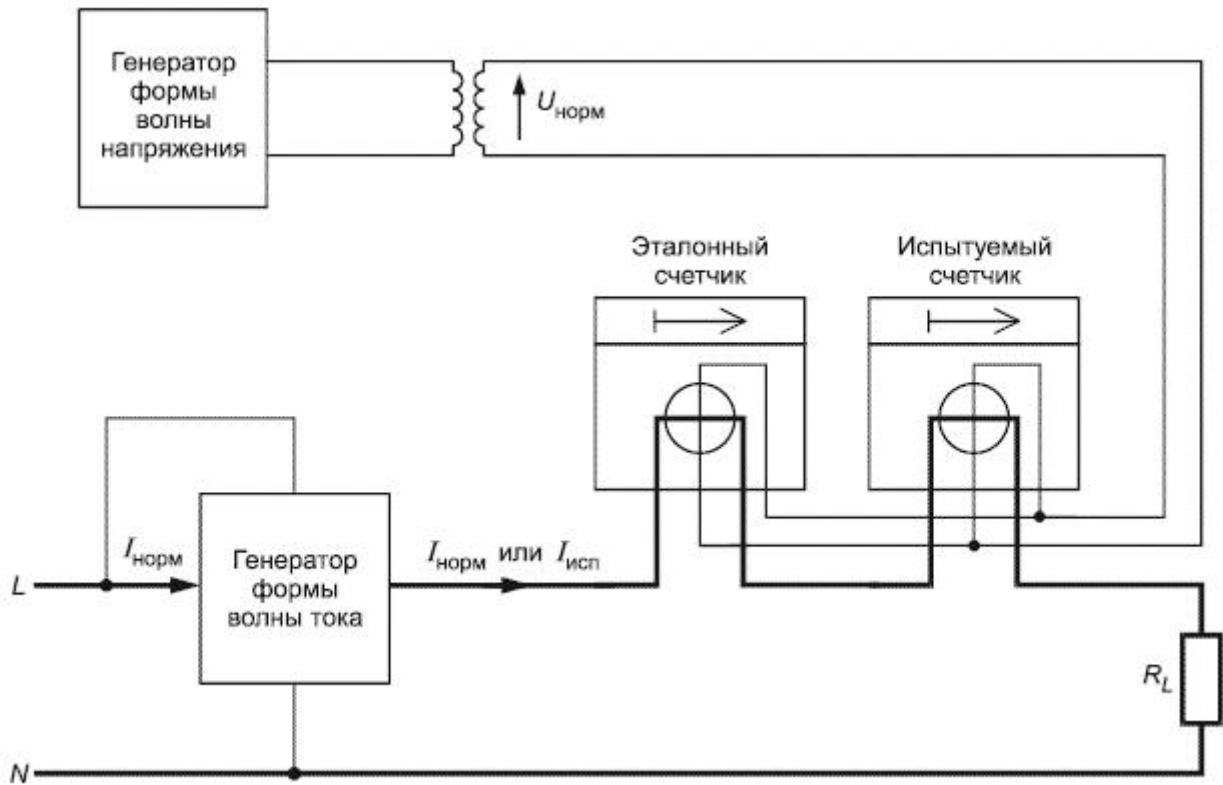
Рисунок А.4 - Схема испытательной цепи (справочная)
