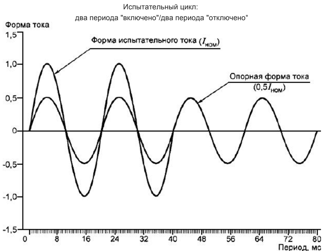
Рисунок А.2 - Форма тока при испытаниях на влияние субгармоник
