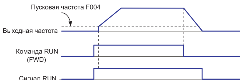
Рис. 10-7 Временная диаграмма сигнала RUN (Работа)
