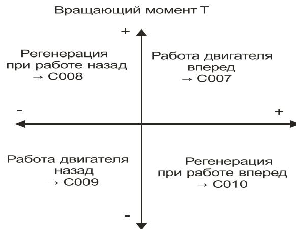
Рисунок 11-2 Предел вращающего момента (4секторный режим)
