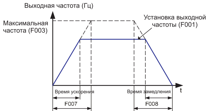
Рис. 7-12 Кривая установки ускорения и замедления ( A089=0 )
