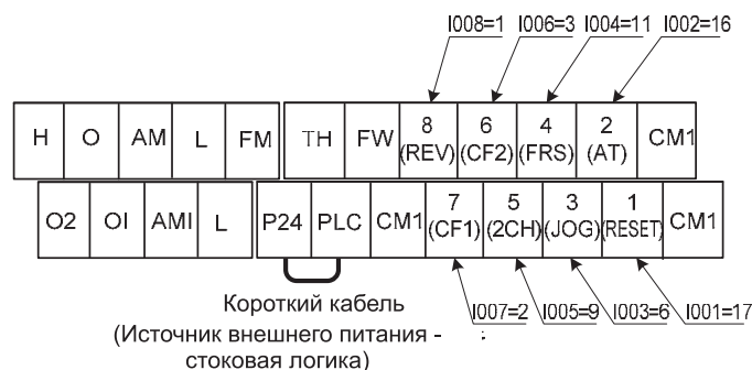
Рис. 9-6 Начальная установочная величина для (I001~I008)
