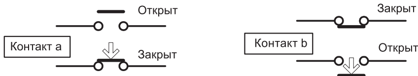
Рис. 9-7 Схема функционирования контакта а и контакта b
