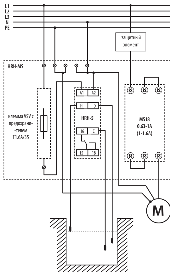
Комплекс контроля уровня жидкости HRH-MS-1A (HRH-MS-1.6A):
