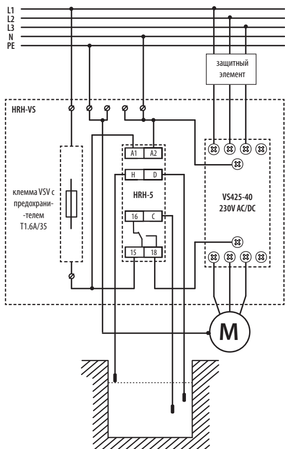
Комплекс контроля уровня жидкости HRH-VS:
