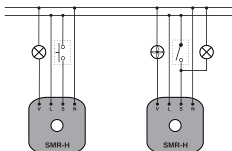
Типичное подключение SMR-H - таймер для светильника
