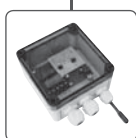
TEV-1 Термостат с „мертвой зоной”, настр. диапазон -20...+20 °C, защита от замерзания, исполнение водозащитное IP65.
