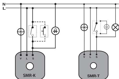
Пример подключения SMR-K - таймер для вентилятора
