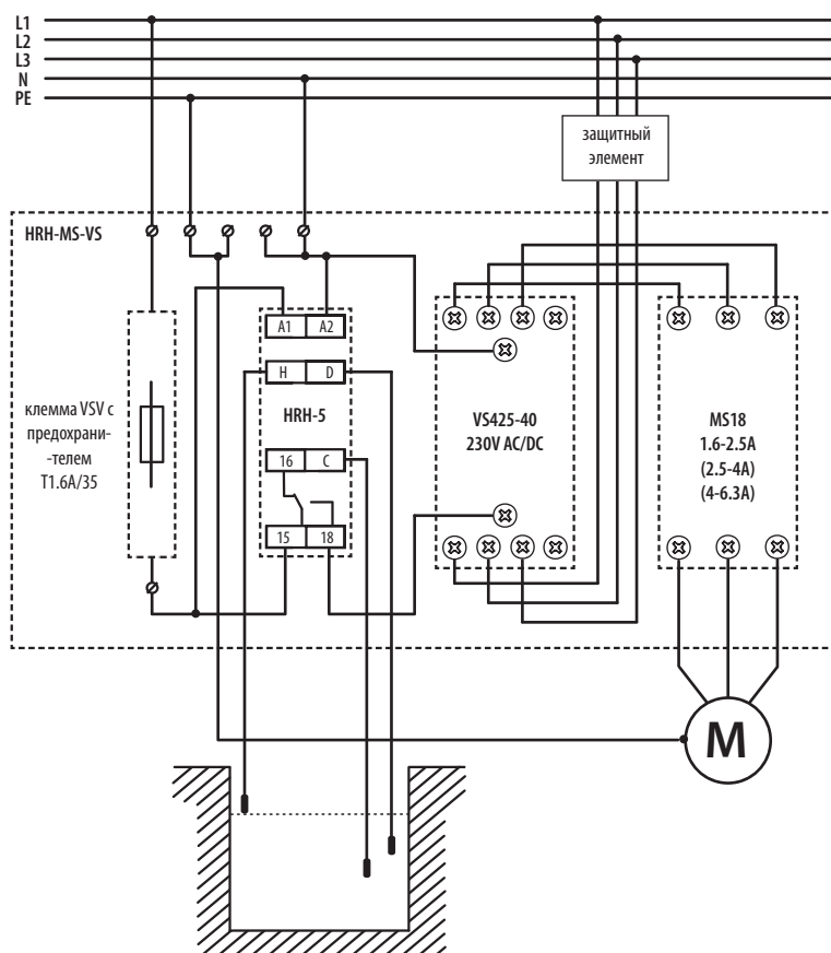
Комплекс контроля уровня жидкости HRH-MS-VS-2.5A (HRH-MS-VS-4A, HRH-MS-VS-6.3A):
