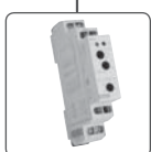
RHT-1 Гигро-термостат для контроля и регулирования температуры в диапазоне 0... +60 °C и относительной влажности в диапазоне 50... 90%.
