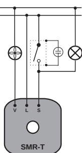
SMR-T: Управление вентилятором в зависимости от освещения
