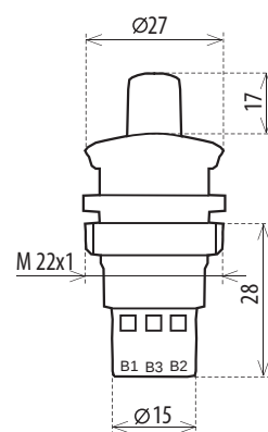
внешний потенциометр к CRM-2HE, CRM-91HE
