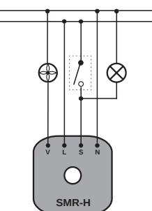
Управление вентилятором в зависимости от освещения
