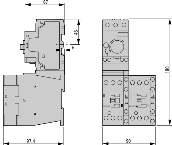
MSC-R-...-M17[...32]BBA...
