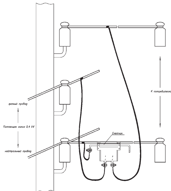
Установка счетчика на ответвлениях к вводу от ВЛН-0,4 кВ
