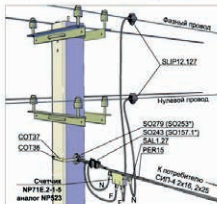
Установка счетчика на ответвлениях к вводу от ВЛН-0,4 кВ
