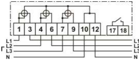
Трехфазные счетчики NP 73L.1-1-2, NP 73L.2-5-2 прямого включения
