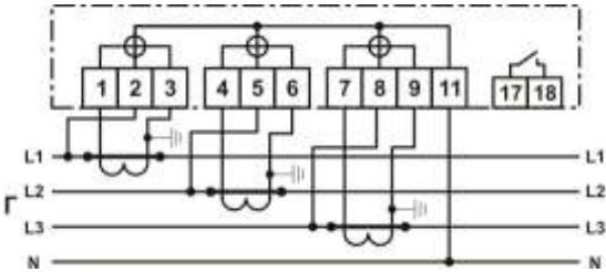
Трехфазный счетчик NP 73L.3-5-2 трансформаторного включения
