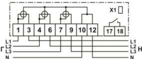
NP 73E.2-2-2– счетчик прямого включения
