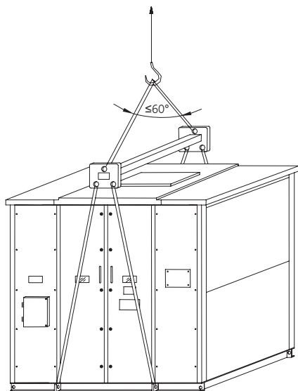
Погрузка и разгрузка трансформатора с оболочкой
