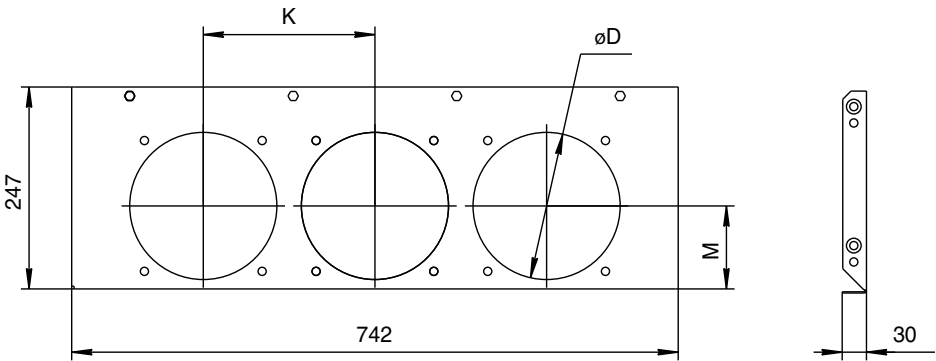
Вырезы для установки проходных изоляторов
