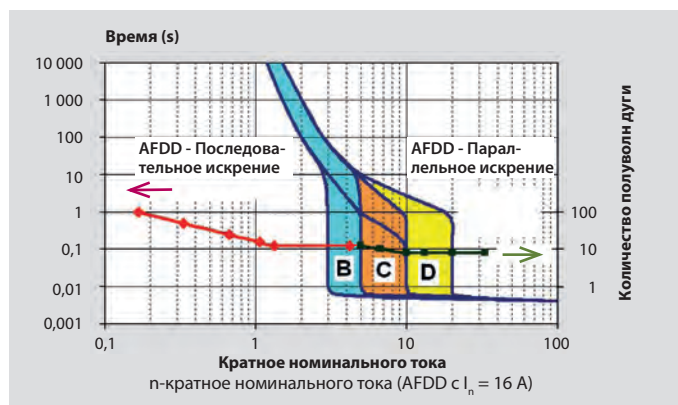
Защита автоматическим выключателем
