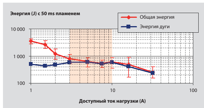
Энергия заметного пламени в зависимости от тока нагрузки
