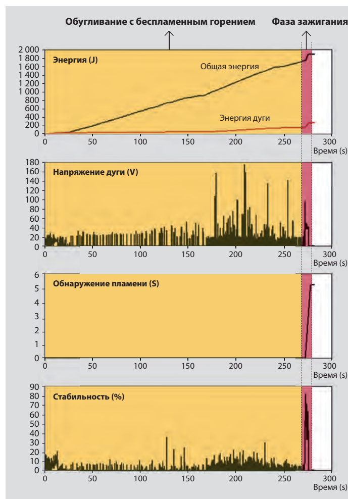
Развитие дуги на примере 2 А / 240 V
