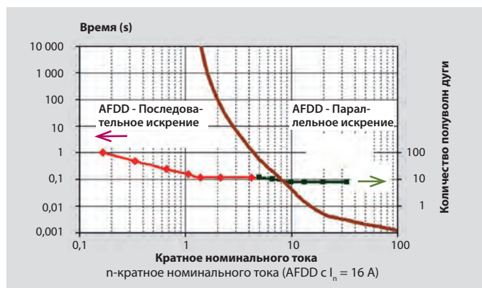
Защита предохранителем
