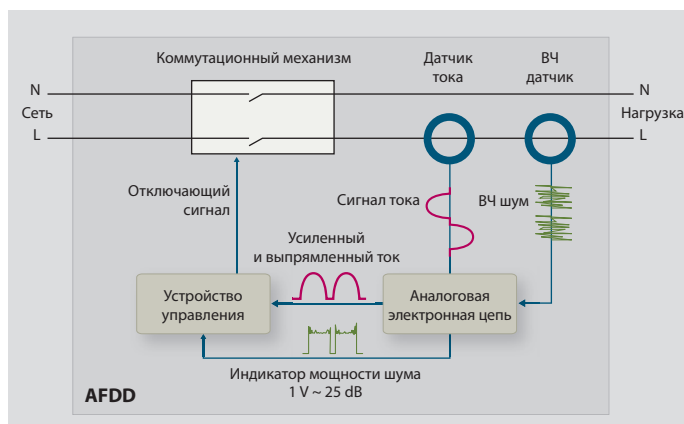
Базовая конструкция AFDD
