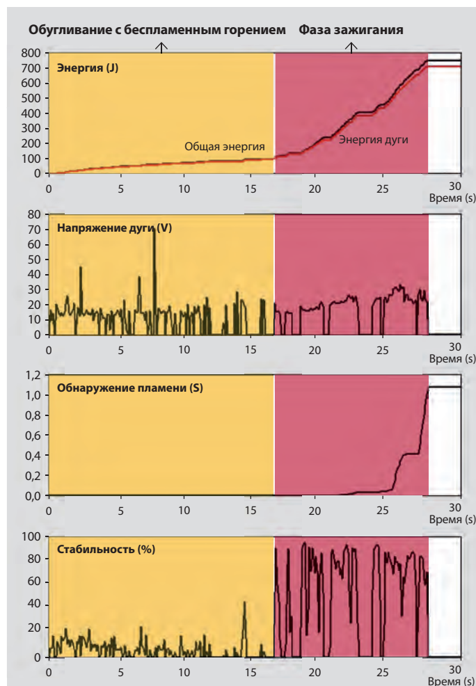
Развитие дуги на примере 5 А / 230 В
