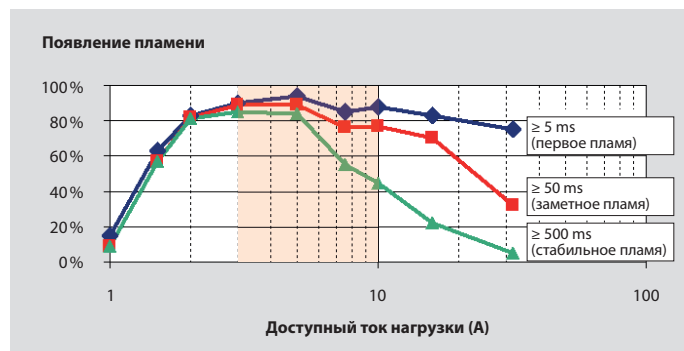
Вероятность появления пламени в зависимости от тока нагрузки
