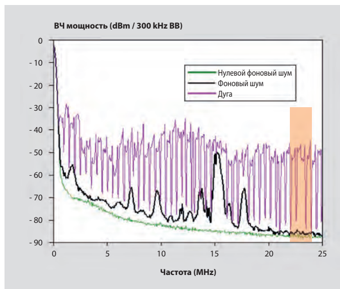
ВЧ шум (шум фона и дуг)
