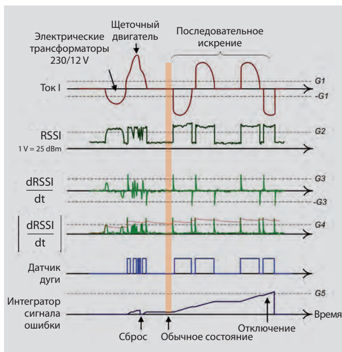
Оценка сигнала при обнаружении последовательного искрения
