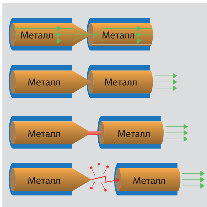
Дуга на контактах
