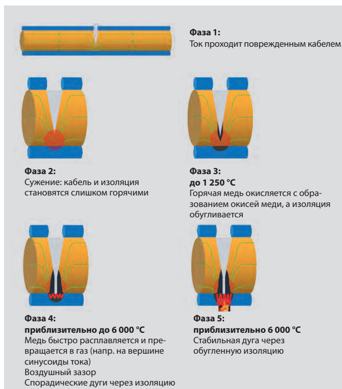
Вспыхивание пожара вследствие последовательного искрения
