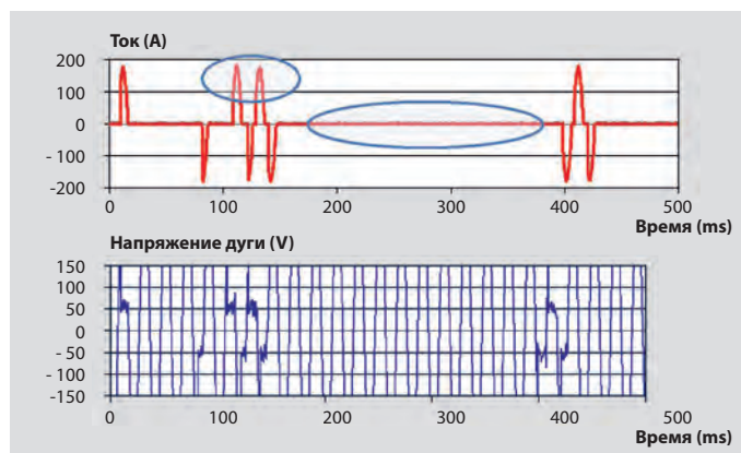
Характеристика тока и напряжения для параллельного искрения
