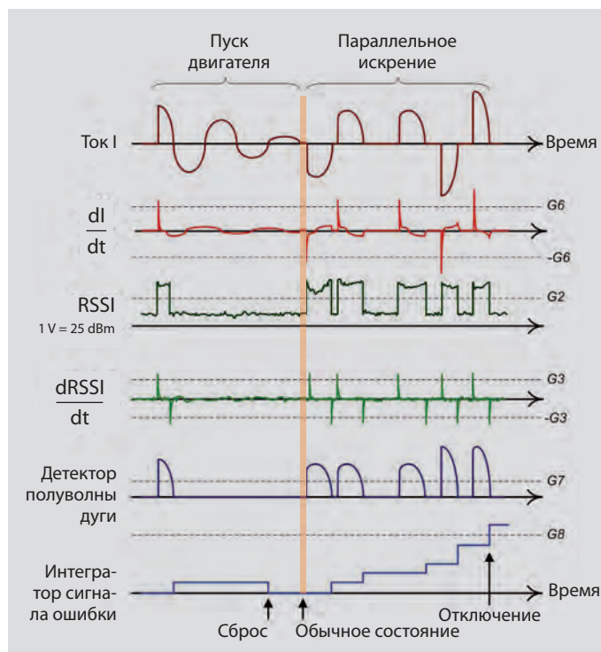
Оценка сигнала при обнаружении параллельного искрения
