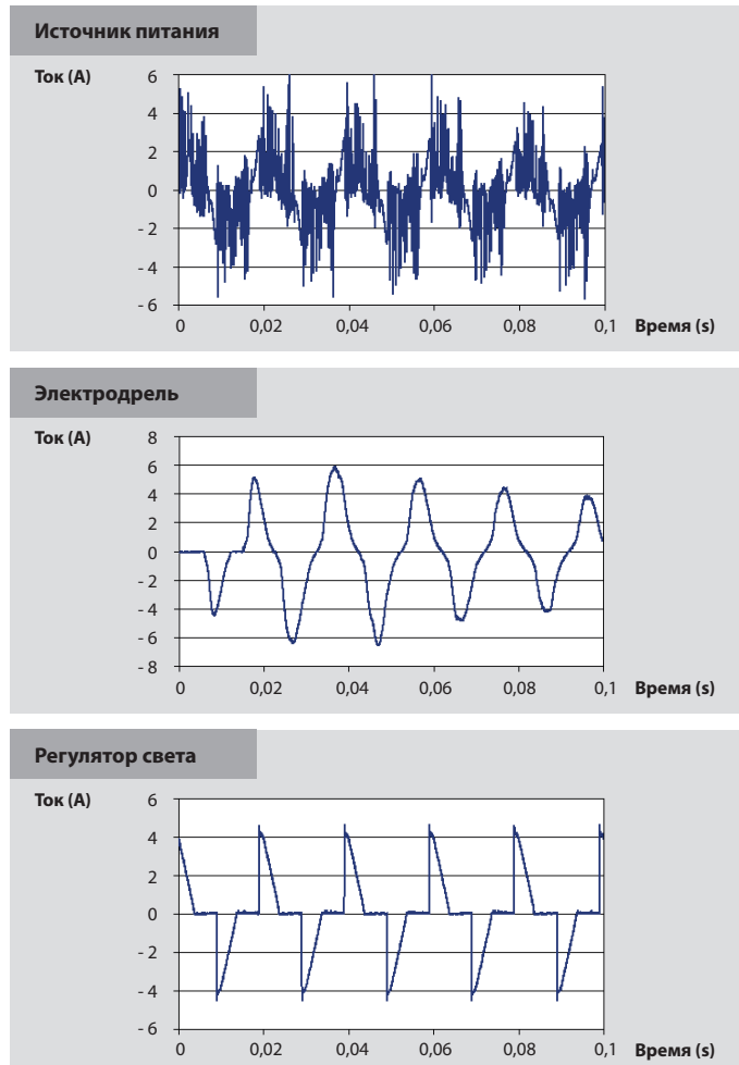
Примеры электрических нагрузок с ВЧ сигналами
