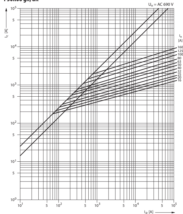
Характеристика токоограничения P50R06 gR, aR
