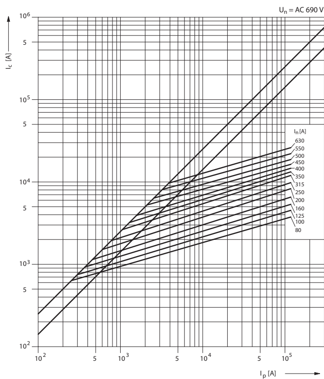
Характеристика токоограничения P50U06, P52U06 aR
