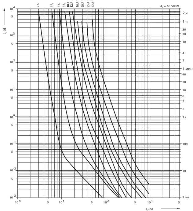
Времятоковая характеристика PVA10, PV10 1) gG
