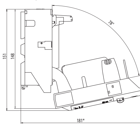
FH000-3A/T, FH000-1A/T и FH000-3L/T
