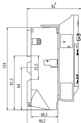
FH000-1A/T, FH000-3A/T и FH000-3L/T
