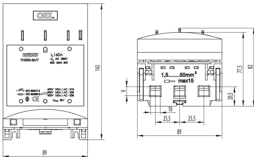
FH000-3A/T, FH000-1A/T и FH000-3L/T
