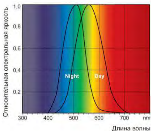
ВИДИМОЕ ИЗЛУЧЕНИЕ
