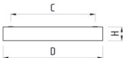
Разрез профиля оптической системы
