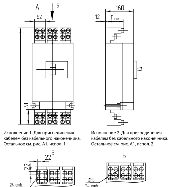
Рисунок А.2. Выключатели типов ВА52-41, ВА53-41, ВА55-41, ВА56-41 стационарного исполнения с ручным приводом для переднего присоединения
