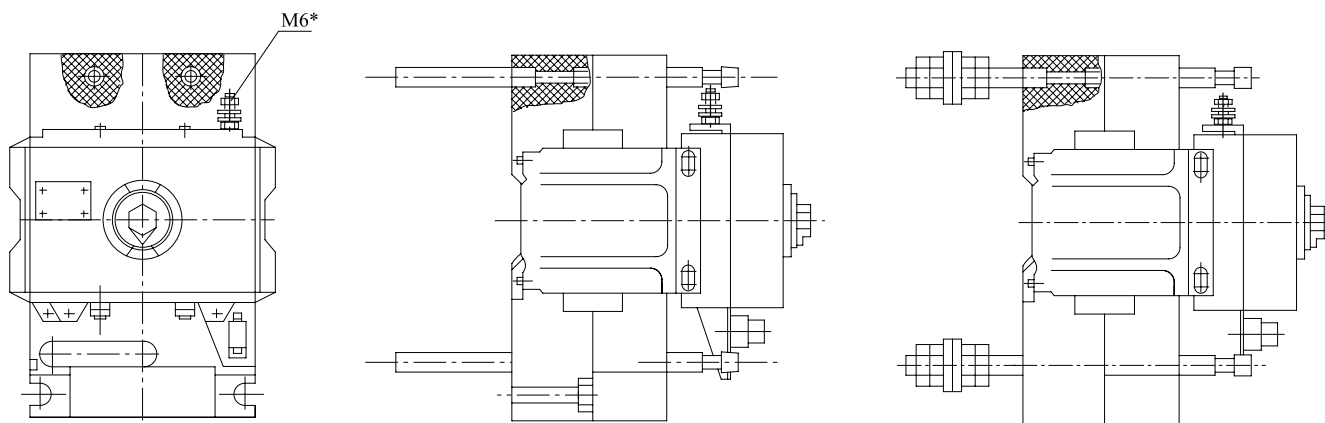
Рисунок А.6. Выключатели типов BA52-41, BA53-41, BA55-41, BA56-41 стационарного исполнения с электромагнитным приводом для заднего присоединения
