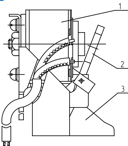
Рисунок 3. Расцепитель независимый
