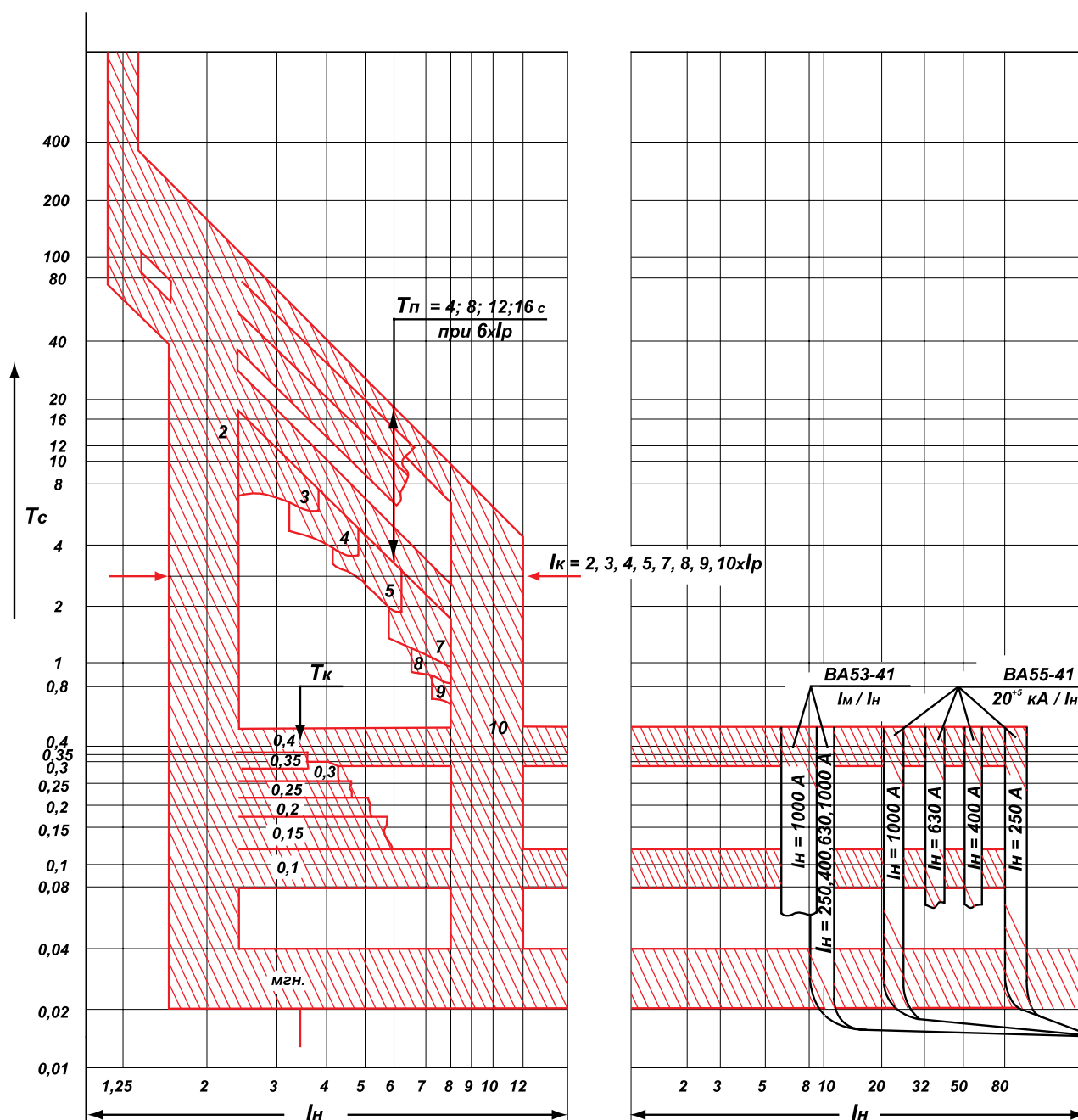
Рисунок В.1. Временотоксовая характеристика выключателей переменного тока ВА53-41 и ВА55-41 с блоками МРТ1-МП, МРТ2-МП
