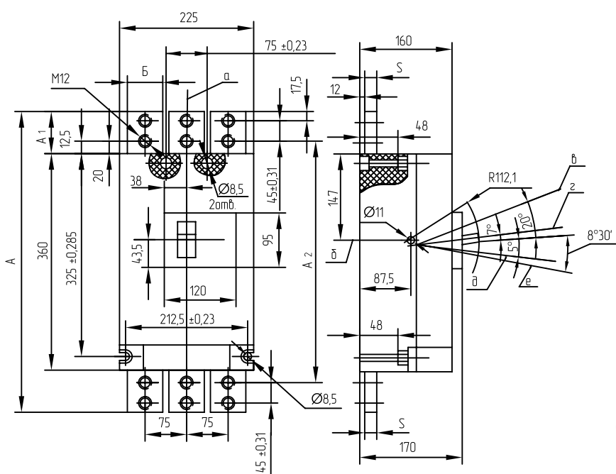
Исполнение 2 для присоединения шиной (остальное см. исполнение 1)
