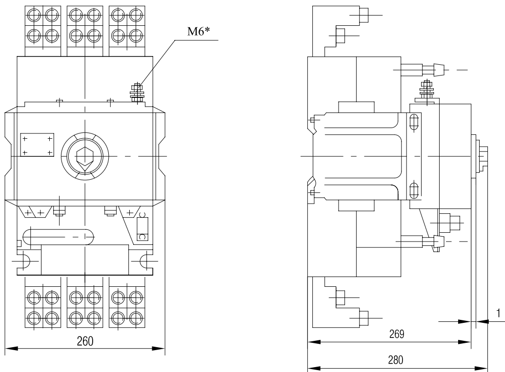
Рисунок А.5. Выключатели типов BA52-41, BA53-41, BA55-41, BA56-41 стационарного исполнения с электромагнитным приводом
