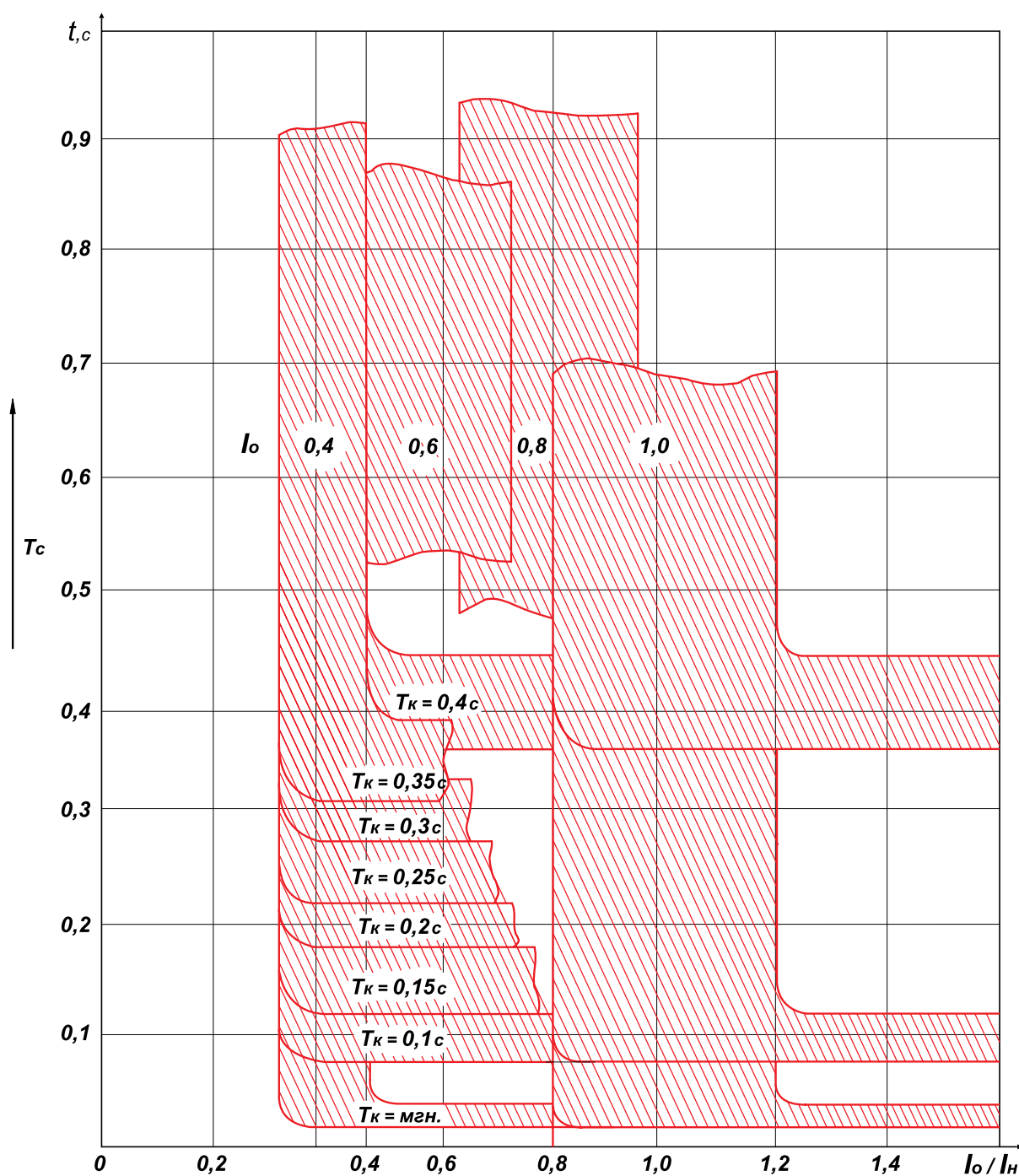
Рисунок В.5. Временная характеристика выключателей переменного тока ВА53-41 и ВА 55-41 с защитой от однофазных замыканий
