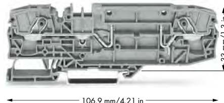
Оранжевый штекерный размыкатель (2006-8401) в рабочем положении
