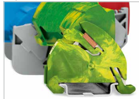
Держатель включает розетку с фиксирующим устройством для сборной шины 10 x 3 мм. Контакт между сборной шиной и рейкой устанавливается автоматически после установки ее на защелку на несущую рейку. Один конец шины устанавливается на держатель шины с заземлением, второй вставляется в среднюю часть изолированного держателя шины.
