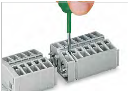
Извлечение клеммы.
