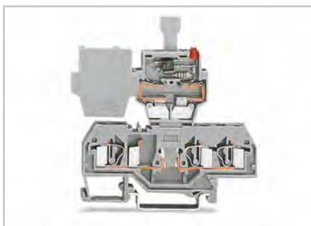
Вставка с предохранителем с индикацией перегорания на 3-проводной несущей клемме.
