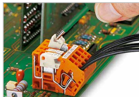
Открытие ножевого размыкателя.
