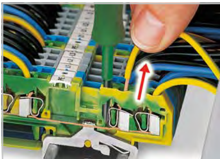
Извлечение проводника при помощи монтажного инструмента.
