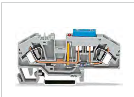
2-проводные клеммы для автомобильных предохранителей с ножевым контактом
