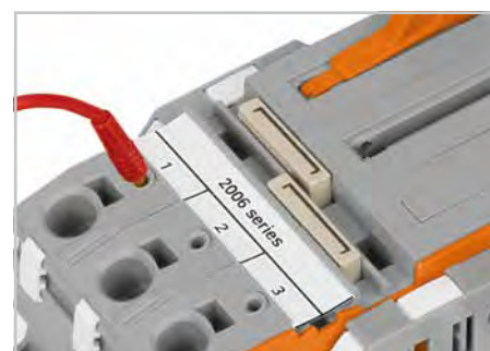
Объединение клемм шириной 15 мм с помощью гребешковых перемычек: от 1 до 3 (2006-433) и от 1 до 5 (2006-435). Тестовые разъемы на обеих сторонах клемм обеспечивают возможность прямого измерения.
