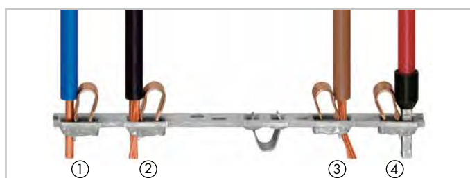
Клеммы Push-in CAGE CLAMP® для вставного присоединения обеспечивают подключение одного проводника на зажим.
