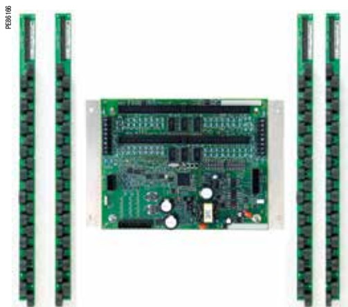
PowerLogic™ BCPM и платы с трансформаторами тока с неразъёмным сердечником
