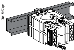
Монтаж на DIN-рейке
