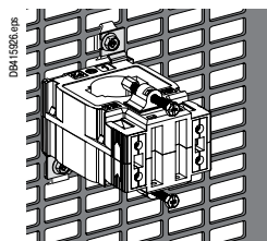
Установка на монтажной плате
