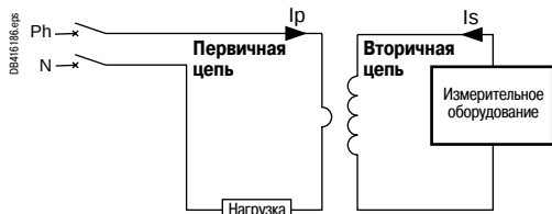
Схема применения ТТ
