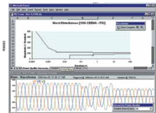
Оциллограмма переходного процесса и отчёт о качестве электроэнергии
