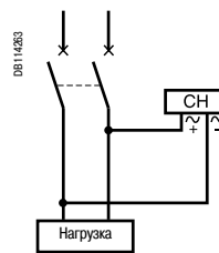
СН 48 x 48
