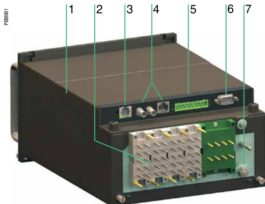
Интеллектуальный счётчик энергии PowerLogic™ ION8800
