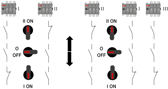
Реверсивная сблокировка
