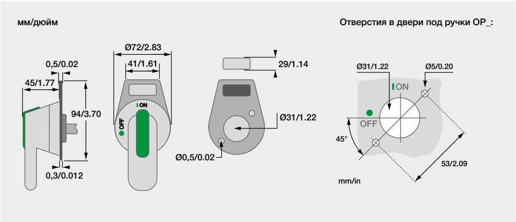
Размеры таблички с обозначениями для рукояток
