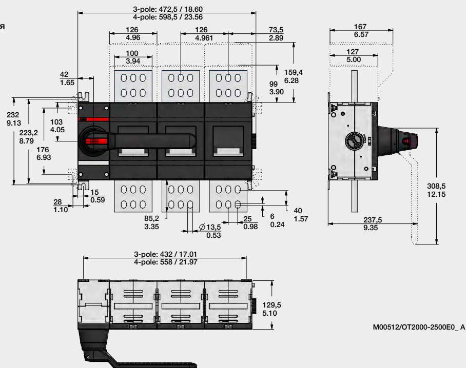
OT2500_K Механизм переключения сбоку выключателя мм/дюйм
