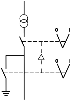
Механическая блокировка
