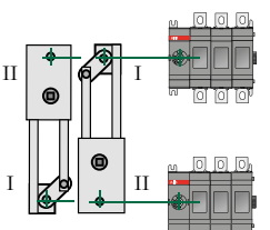
Реверсивная сблокировка
