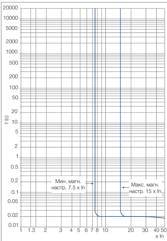
DWB400_M (Двигатель)
