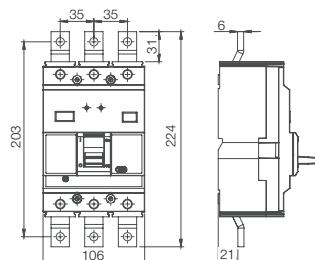
Габарит 250 3P + BE DWB250 3P
