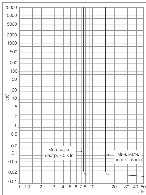
DWB800 (Двигатель)
