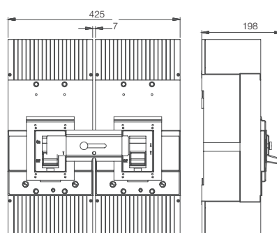
Габарит 1600 3P + BLIM DWB1600
