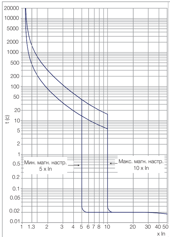
DWB400_M (Двигатель)
