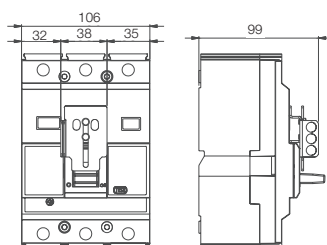
Габарит 250 3P + PLW DWB250
