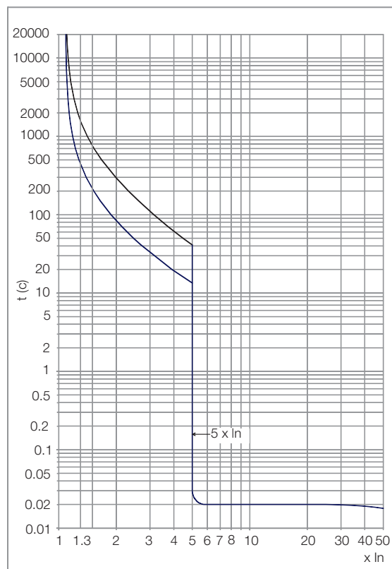
DWB250_G (Генератор)
