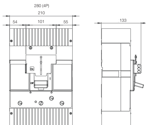
Габарит 800-1000 + PLW800-1000
