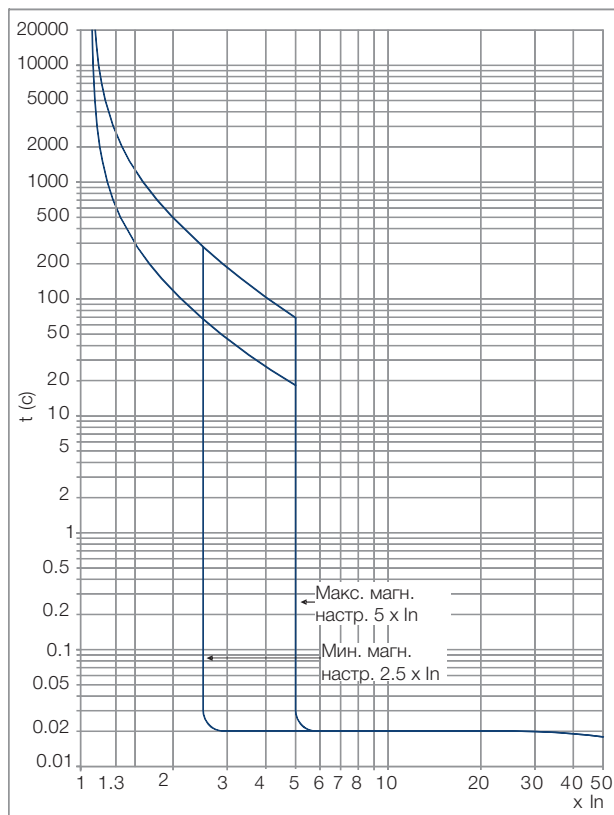
DWB800 (Генератор)
