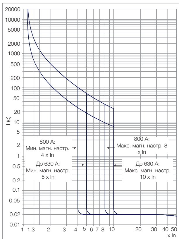
DWB800 (Распределительная цепь)
