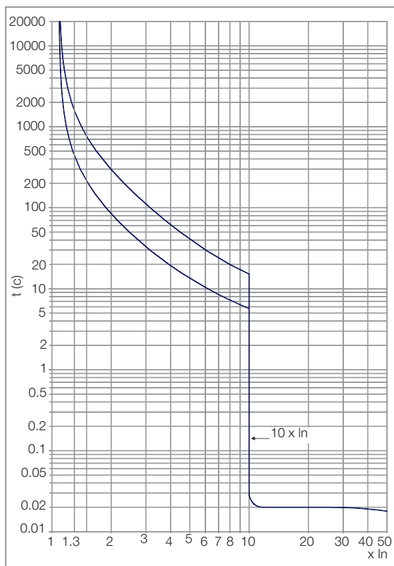
DWB250_M (Двигатель)
