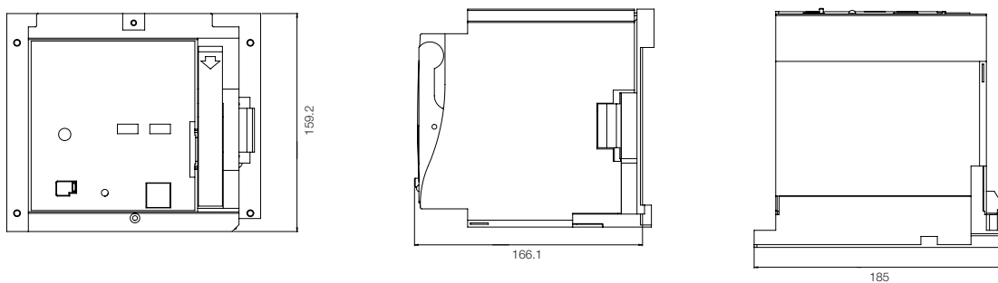
AM DWB400
