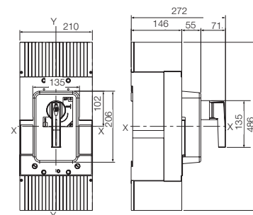
Габарит 1600 3P + MRI DWB1600
