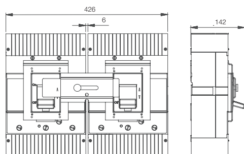
Габарит 800 3P + BLIM DWB800 / DWB1000
