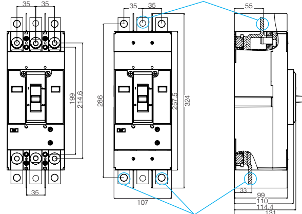
Габарит 400 3P + BE DWB400 3P
