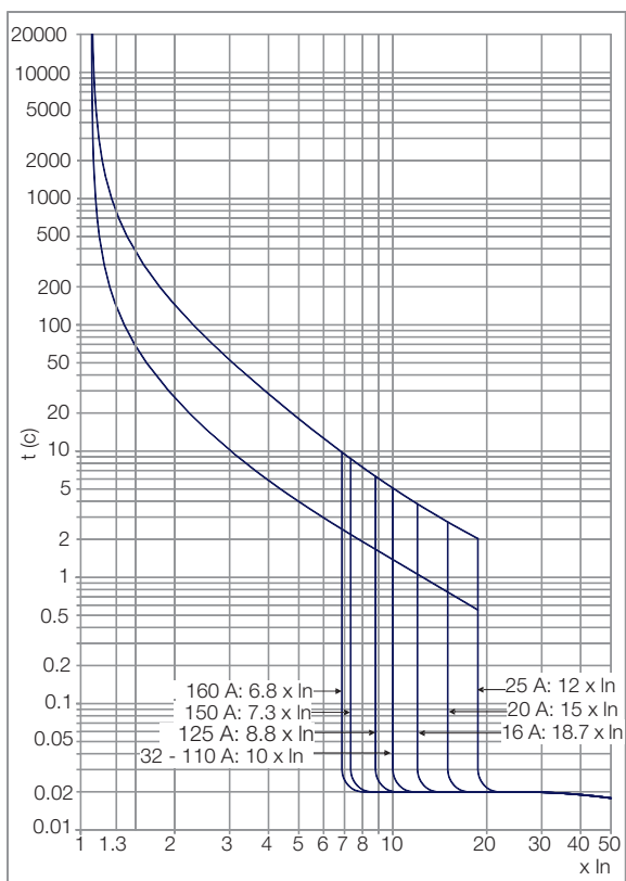
DWB160_M (Двигатель)
