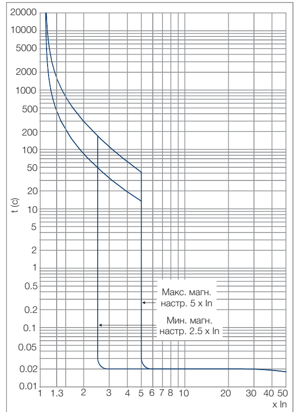
DWB400_G (Генератор)
