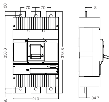
Габарит DWB800-1000 3P + BE DWB800-1000
