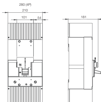
Габарит 1600 + PLW1600
