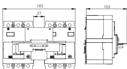
Габарит 160 3P + BLIM DWB160 3P
