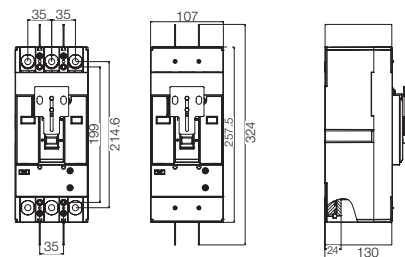
Габарит 400 3P + PLW DWB400
