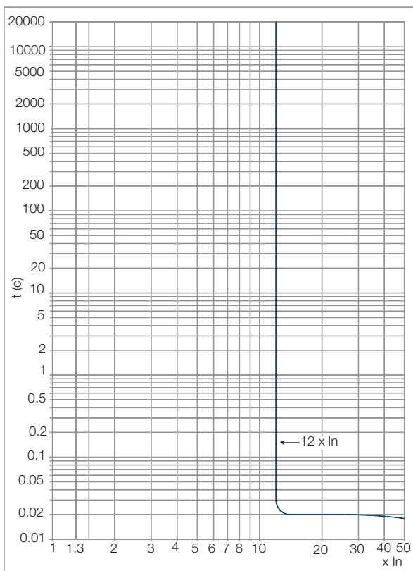
DWB160_M (Двигатель)
