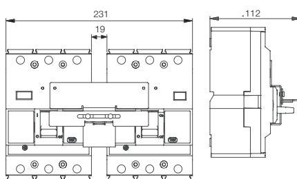
Габарит 250 3P + BLIM DWB250 3P
