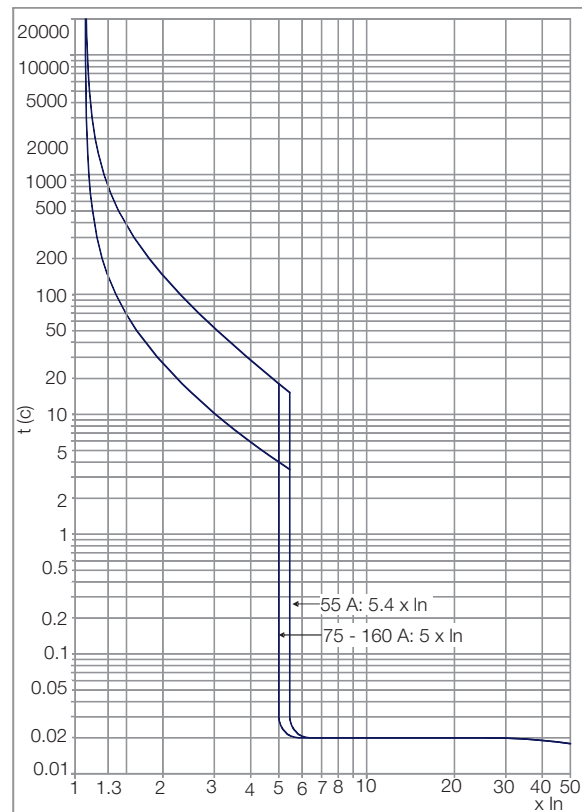
DWB160_G (Генератор)
