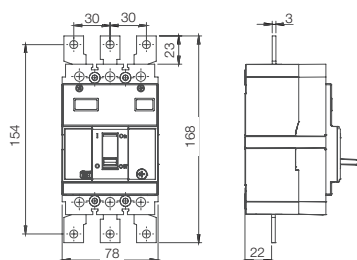
Габарит 160 3P + BE DWB160 3P
