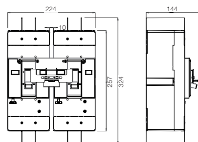
Габарит 400 3P + BLIM DWB400 3P
