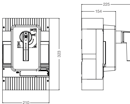
Габарит 800-1000 3P + MRI DWB800-1000
