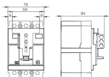
Габарит 800-1000 + PLW800-1000
