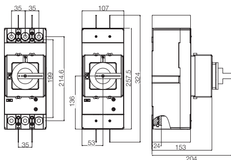
Габарит 400 3P + MRI DWB400
