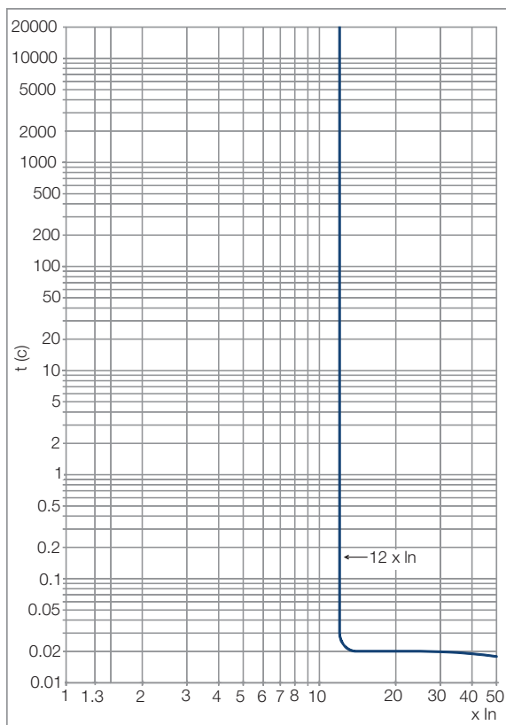
DWB250_M (Двигатель)
