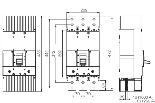
Габарит 1600 3P + BE DWB1600
