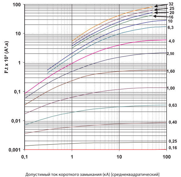
Кривая зависимости I^2t при 415В - MPW25/25i
