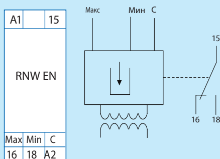
Схема соединений
