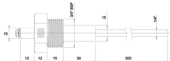
Размеры (мм)
