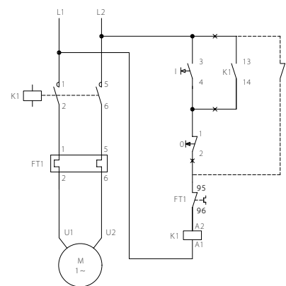
Однофазный пускатель для прямого пуска от сети
