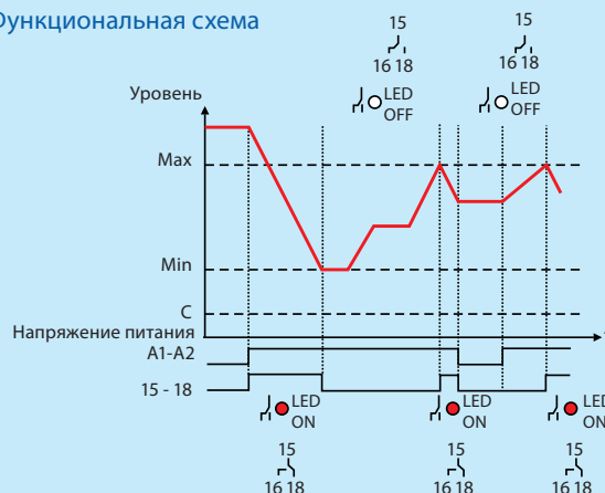
Функциональная схема
