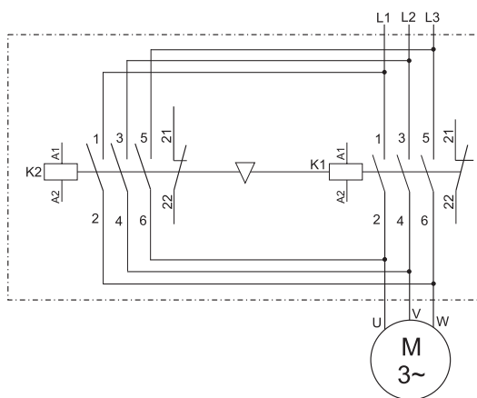
Реверсивные пускатели
