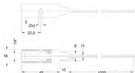
Размеры (мм)
