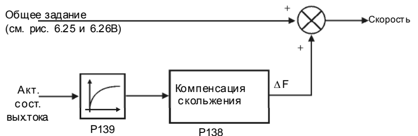
Рис. 6.8 - Блок-схема P138
