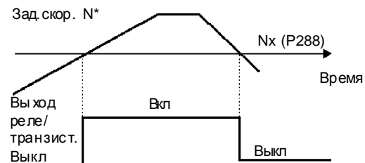
e) N^* > N_x
