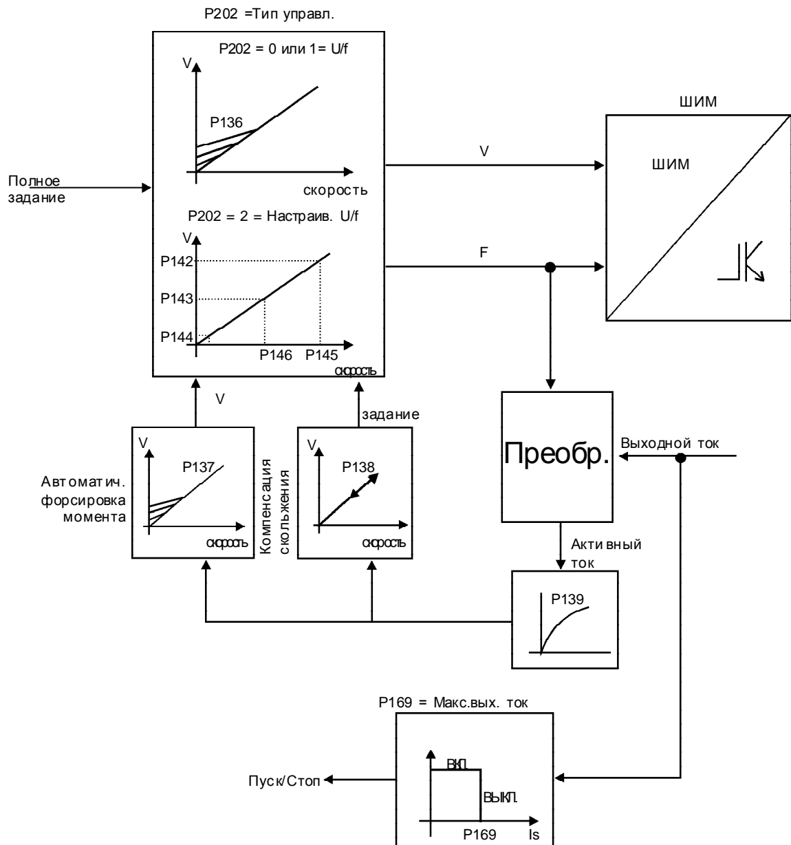
Рис. 6.26В - Блок-схема управления U/f = \text{const}
