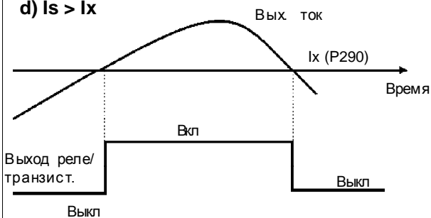
d) I_s > I_x
