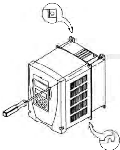
а) Размеры 1 и 2
