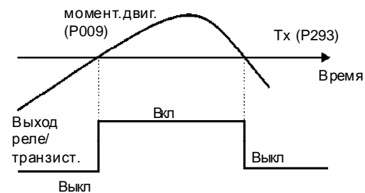
g) Момент > Tx
