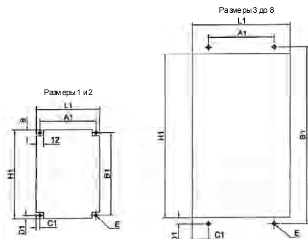
с) Габаритные размеры (см.таблицу 3.4)
