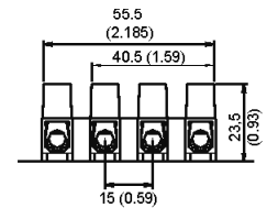
Тип/47 - Размеры в мм. Клеммные зажимы для негибкого кабеля 16 мм 2 и гибкого кабеля 10 мм 2 .
