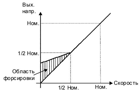
Рис. 6.7 - U/f управление с автоматической форсировкой по моменту
