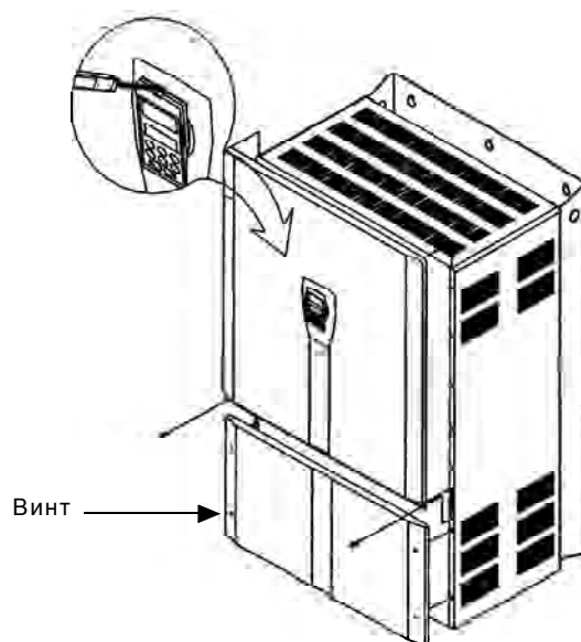
с) Размеры 9, 10 и 10E
