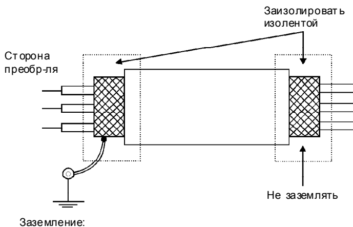
Рисунок 3.14 – Подключение экрана
