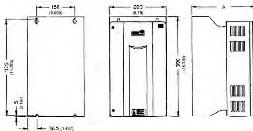
Рис. 8.25 - Размеры DBW-01 и DBW-02 (в мм)
