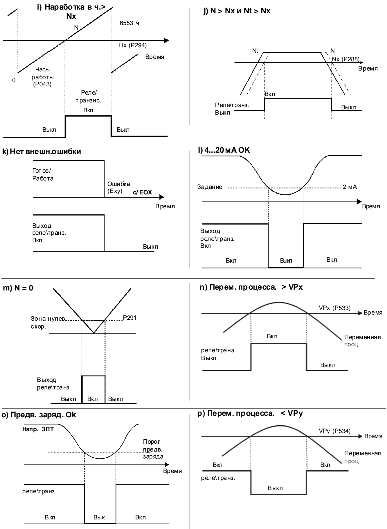
Рис. 6.34 i) р) - Работа цифровых выходов (продолжение)
