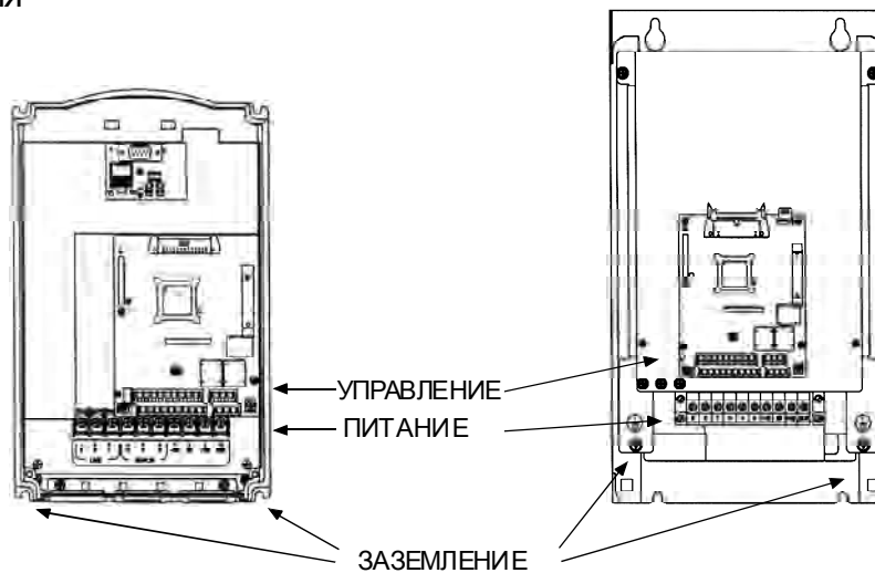
a) Размеры 1 и 2
