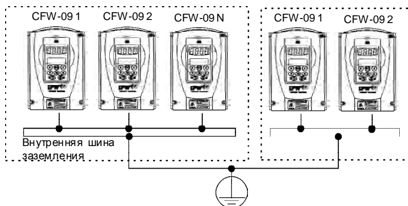
Рисунок 3.7 – Заземление нескольких преобразователей
