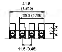
Тип/45 - Размеры в мм. Клеммные зажимы для негибкого кабеля 6 мм 2 и гибкого кабеля 4 мм 2 .
