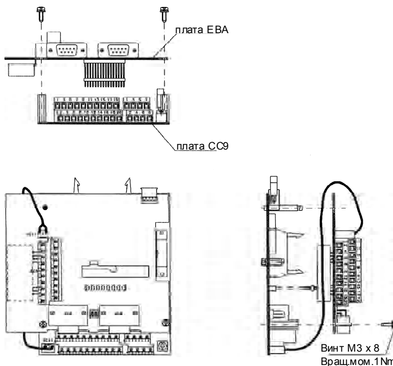
Рис. 8.6 - Установка платы EBB
