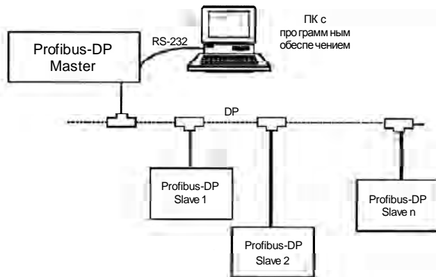
Рис. 8.39 - Сеть Profibus-DP
