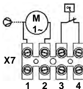
Рис. 8.31 - Клеммник X7
