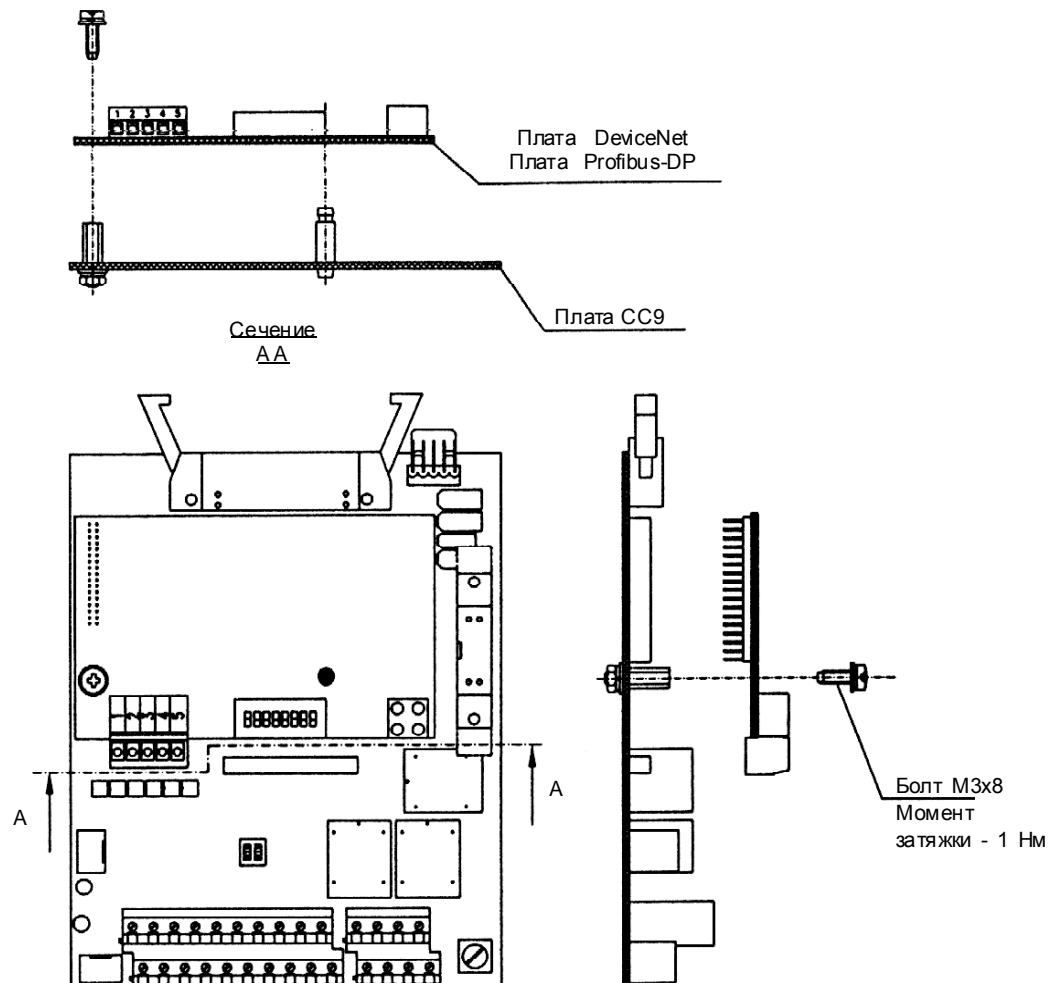
Рис. 8.35 - Установка платы Fieldbus
