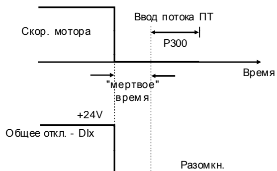
Рис. 6.36 - Торможение при общем отключении
