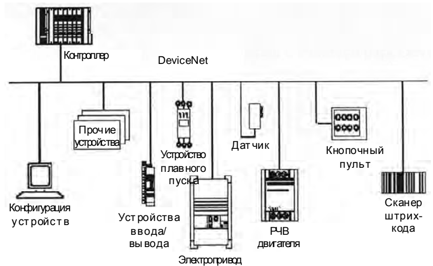
Рис. 8.41 - Сеть DeviceNet
