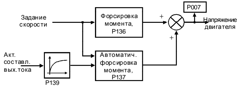
Рис. 6.6 - Блок-схема P137
