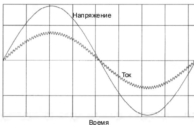
Рис. 8.54А - Работа электропривода в двигательном режиме
