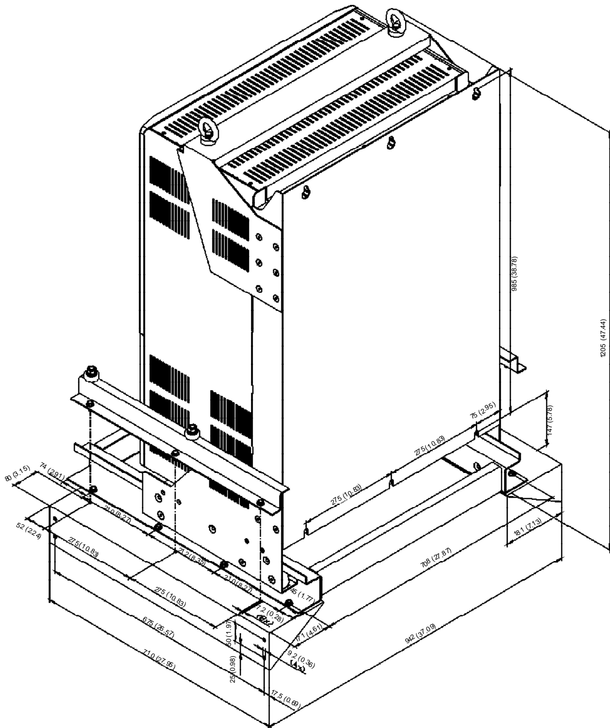
Размеры в мм.(дюймы)
