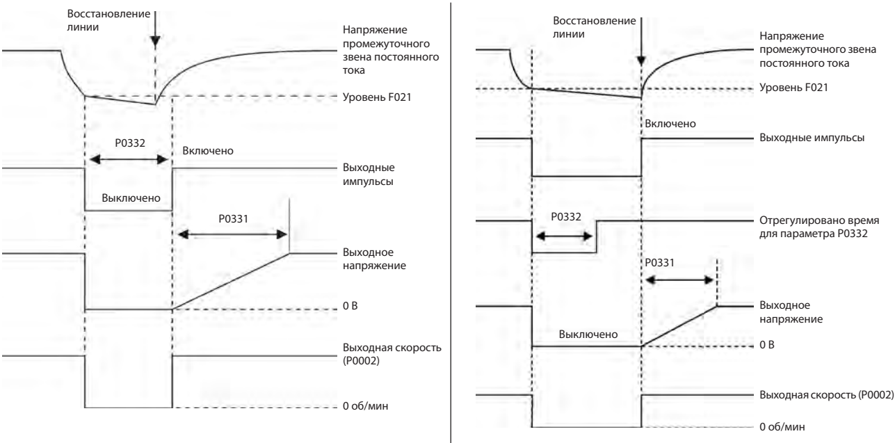
(a) при восстановлении линии до истечения времени, заданного параметром P0332 (b) при восстановлении линии после истечения времени, заданного параметром P0332, но до истечения 2 с (для P0332 \leq 1 с) или до 2 \times P0332 (для P0332 > 1 с)
