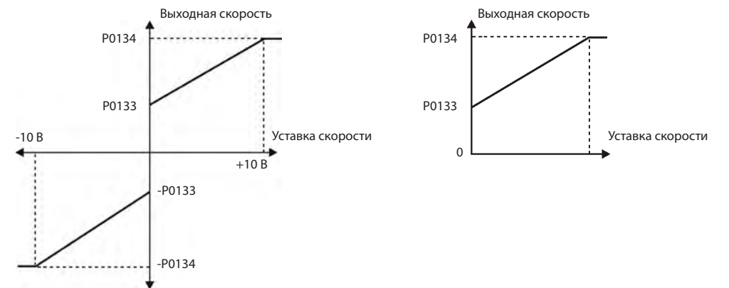
Рис. 12.3 (а). Ограничение скорости при отключенной «зоне нечувствительности» (P0230 = 0)
