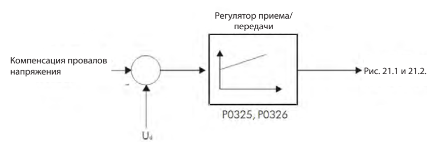
Рис. 21.3. ПИ-регулятор компенсации провалов
