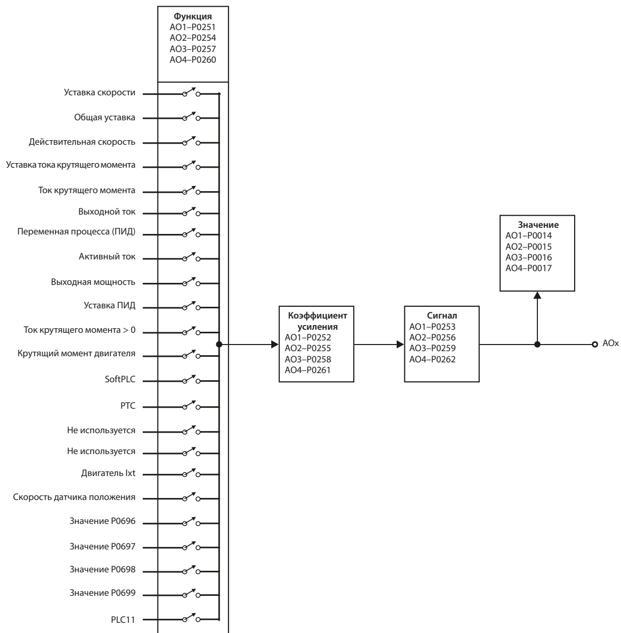
Рис. 13.3. Блок-схема аналогового выхода
