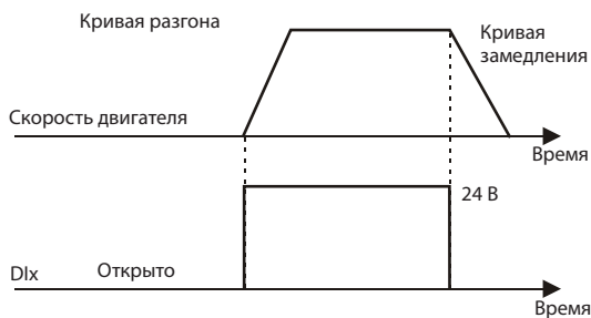
(a) ПУСК/ОСТАНОВ
