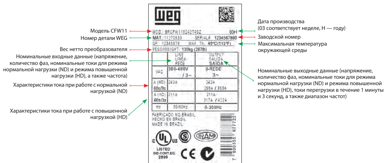
(a) Идентификационная табличка на боковой грани преобразователя для моделей в шкафу (CFW-11)
