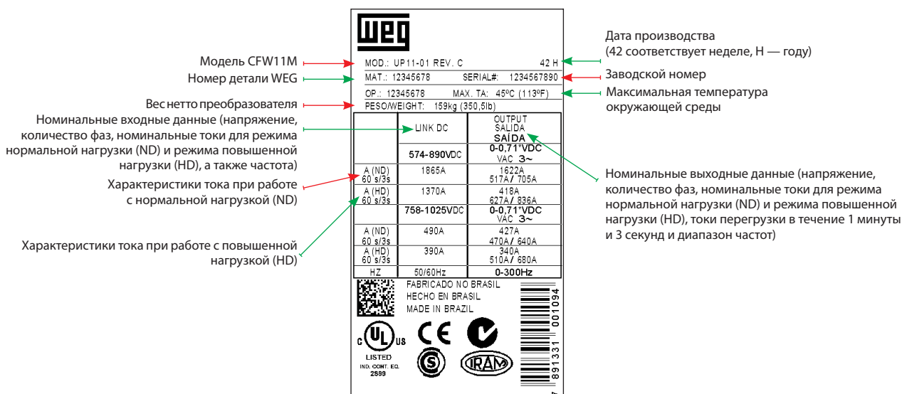
(b) Идентификационная табличка CFW-11M, закрепленная внутри панели, на которую установлен преобразователь
