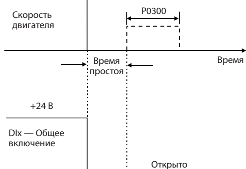
Рис. 12.12. Использование торможения постоянным током посредством общего отключения: режим V/f
