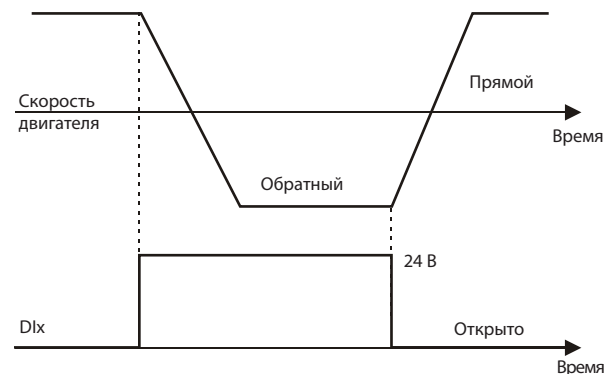
(d) ПРЯМОЙ/ОБРАТНЫЙ
