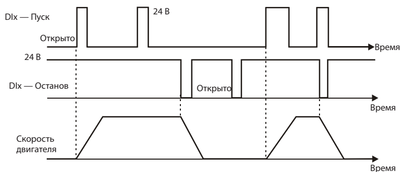
(к) ПУСК/ОСТАНОВ ТРЕХПРОВОДНОЙ ЛИНИИ
