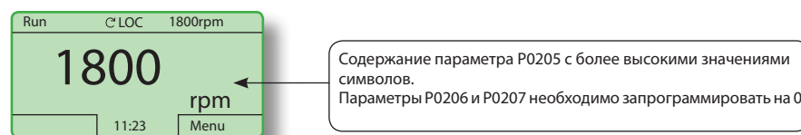
Рис. 5.6. Пример экрана в режиме контроля с P0205, запрограммированным на более высокие значения символов
