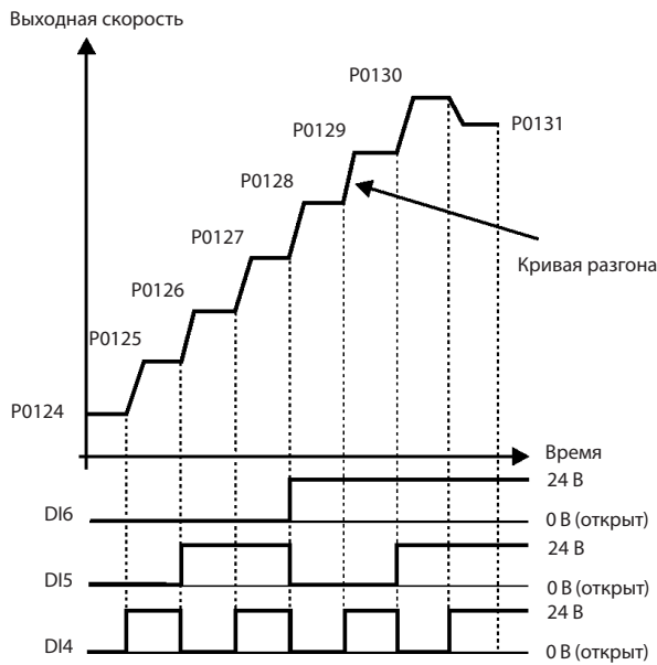
Рис. 12.4. Многоскоростной режим
