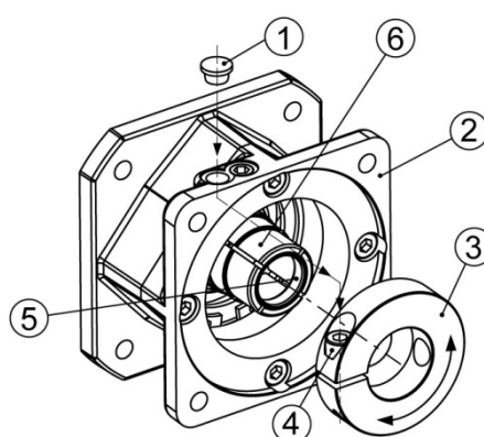
Рис. 14: Вид серво адаптера с гладким сплошным валом
