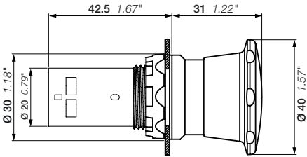
CPM3 Габаритные размеры (мм, дюймы)
