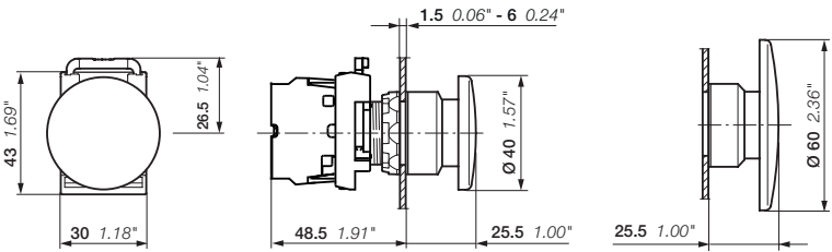
MPM1, MPM2 Габаритные размеры (мм, дюймы)
