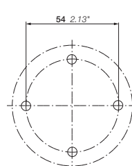
Схема сверления отверстий для сигнальных стоек K70
