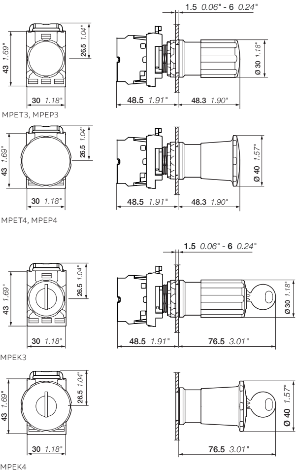
Габаритные размеры (мм, дюймы)
