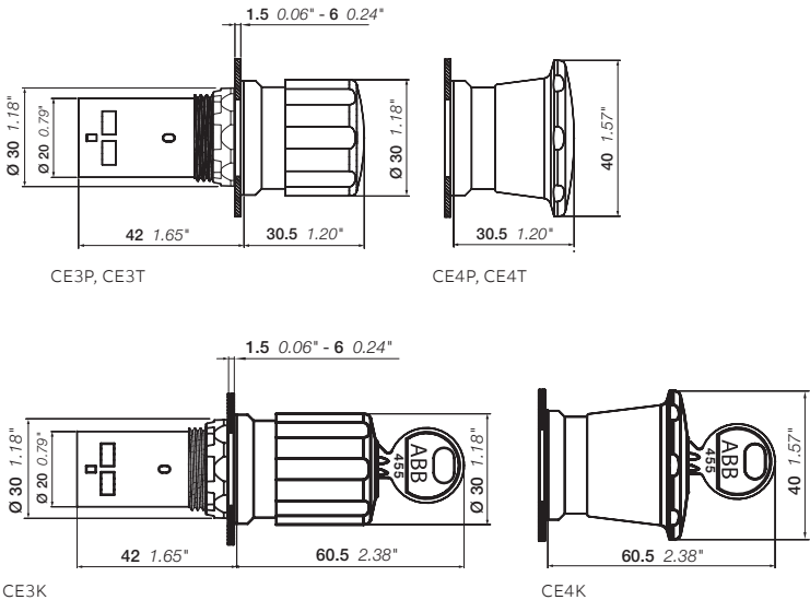
Габаритные размеры (мм, дюймы)
