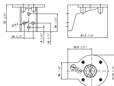
Кронштейн для монтажа на поверхности
