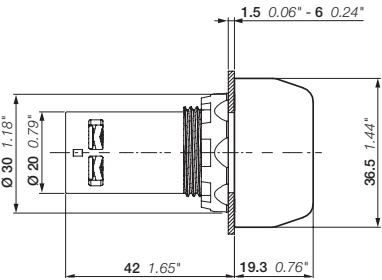
CP6 Габаритные размеры (мм, дюймы)
