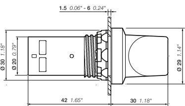
C3SS, короткая ручка Габаритные размеры (мм, дюймы)
