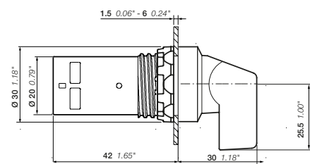
C2SS, длинная ручка
