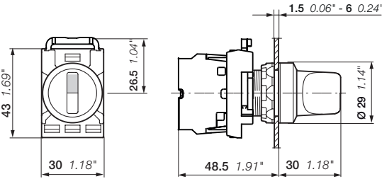
M2SSV, M3SSV Габаритные размеры (мм, дюймы)
