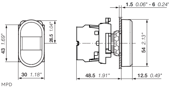
Габаритные размеры (мм, дюймы)
