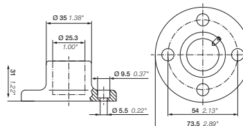
Схема сверления отверстий для сигнальных стоек K70
