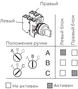
Рабочие положения контактных блоков
