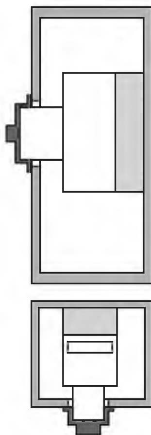
Рисунок R 1 — Механизм управления снаружи оболочки
