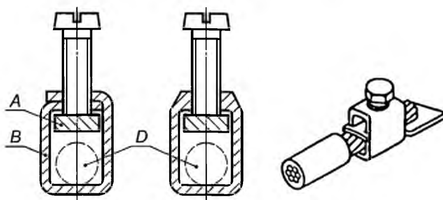
Выходы с непрямой передачей давления
