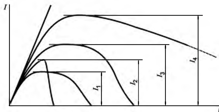
Рисунок 15 — Определение ожидаемого тока отключения после проведения первой калибровки при токе, меньшем номинальной отключающей способности [см. 8.3.4.1.8, перечисление b)]
