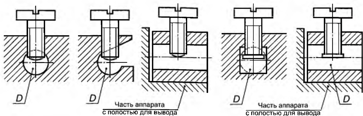
Выходы без прокладок
