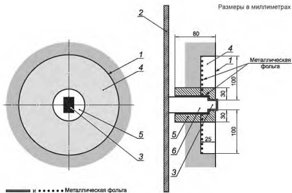
Рисунок R 1 — Механизм управления снаружи оболочки
