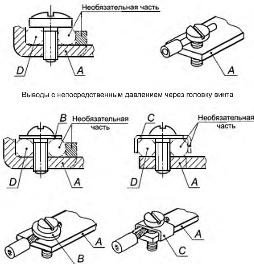
Выводы с косвенным давлением через прокладку
