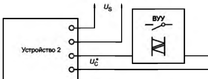
Рисунок U.3 — Раздельные входы для источника питания и цепи управления
