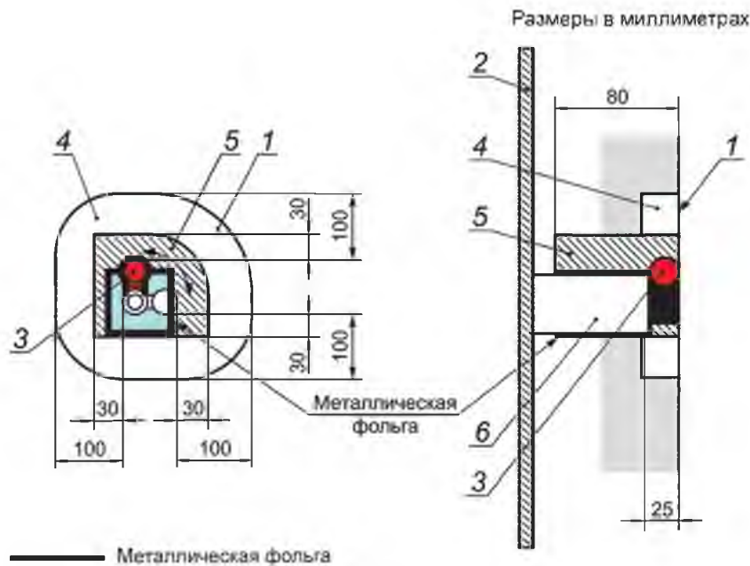
1 — область основания; 2 — монтажная панель; 3 — рычаг; 4 — область с задней поверхностью для защиты руки; 5 — область для защиты пальца; 6 — гнездо выключателя
