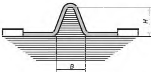
Рисунок G.1 — Размеры ребер
