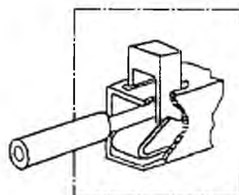
Рисунок D.7 — Безрезьбовые зажимы
