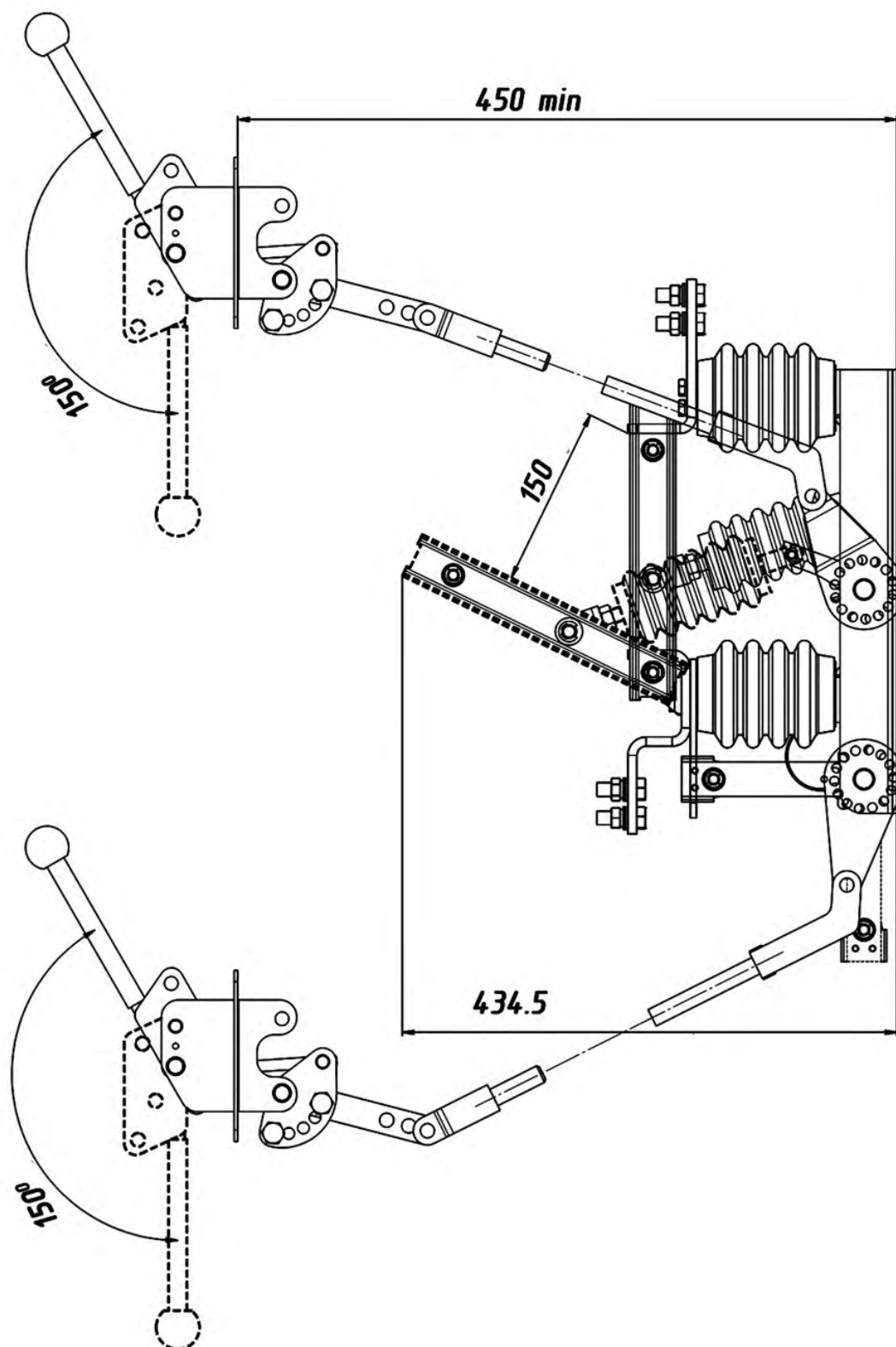
Рис. 13. Монтаж трехполюсных разъединителей типа PB, PB3, PBФ3 с приводом ПР-10, промежуточные тяги (показаны штрихпунктиром) в комплект поставки привода не входят
