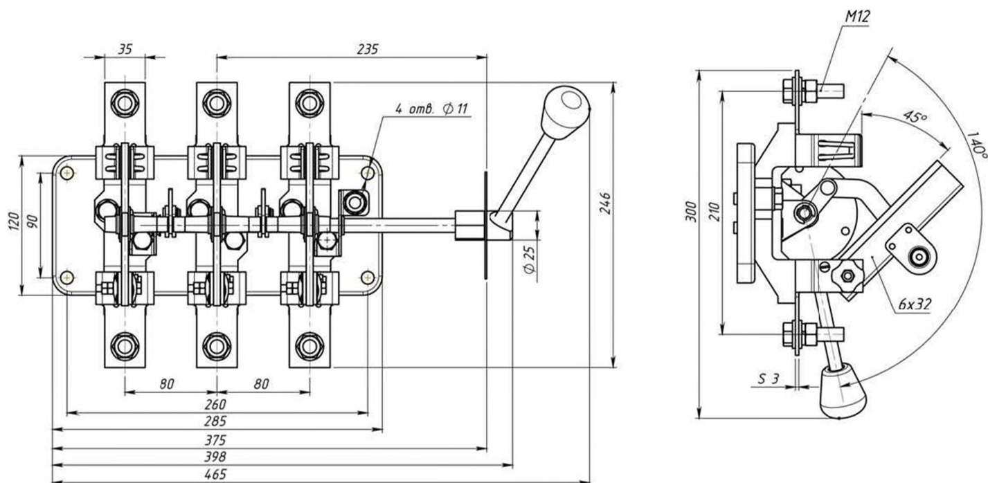
Рис. 5. Разъединитель серии Р с боковой рукояткой РБ-6, на номинальный ток 630 А
