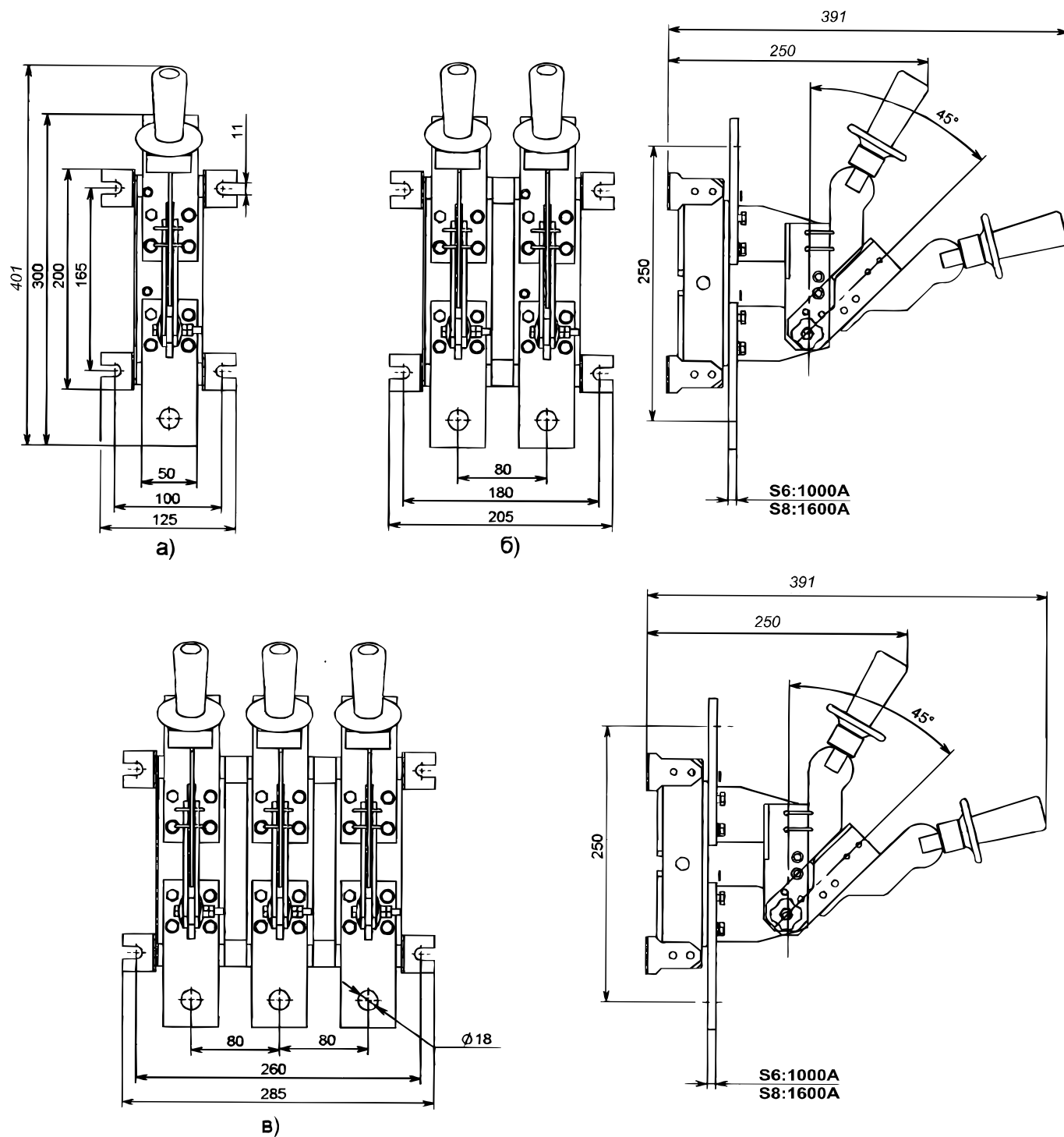
Рис. 27. Разъединитель PE19 с рукояткой для полюсного оперирования а) PE19-41(43)-11170-00 УХЛЗ; б) PE19-41(43)-21170-00 УХЛЗ; в) PE19-41(43)-31170-00 УХЛЗ
