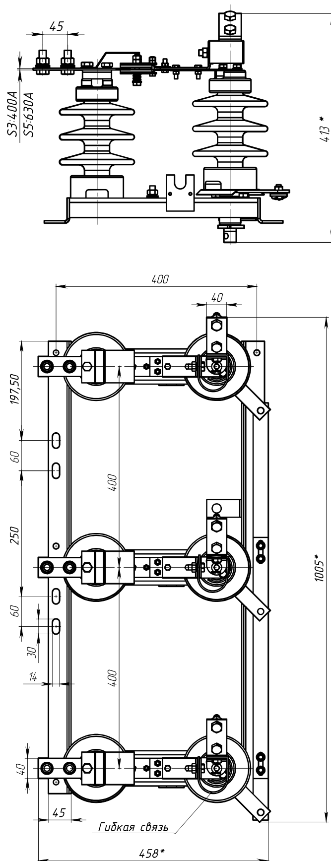
Рис. 4. РЛНД1.0-10II/400(630)-УХЛ1, масса не более 36 кг
