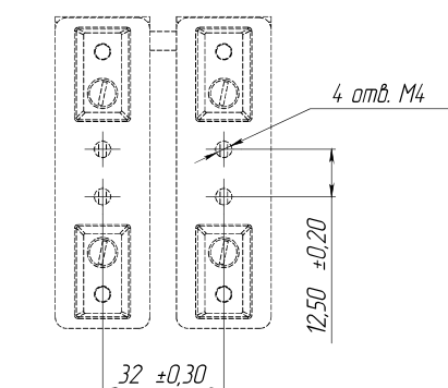
Разметка панели под установку комплекта из двух Р-25-1111
