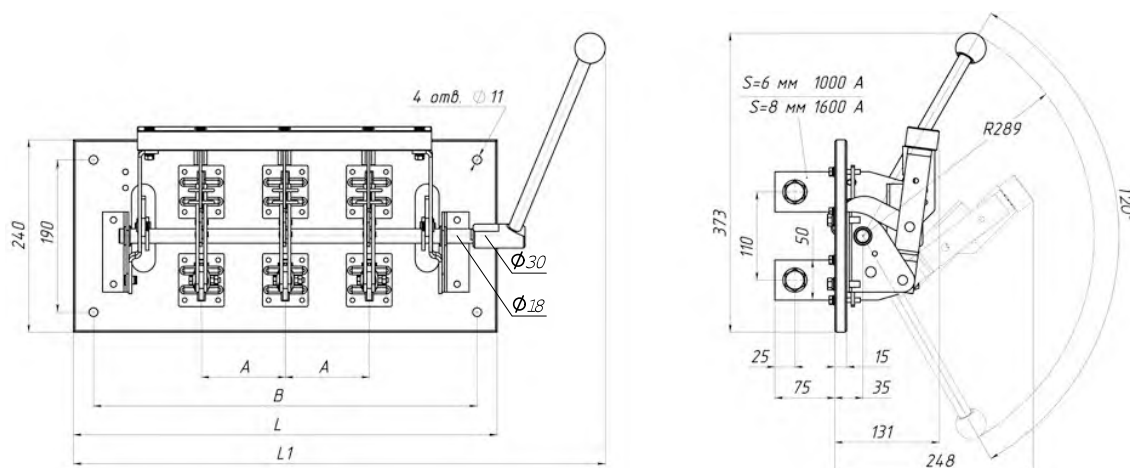
Рис. 21. Разъединитель РЕ19-41(43) -31120-00 УХЛЗ с боковой рукояткой, на изоляционной плите с м/п расстоянием 105, 120 и 130 мм
