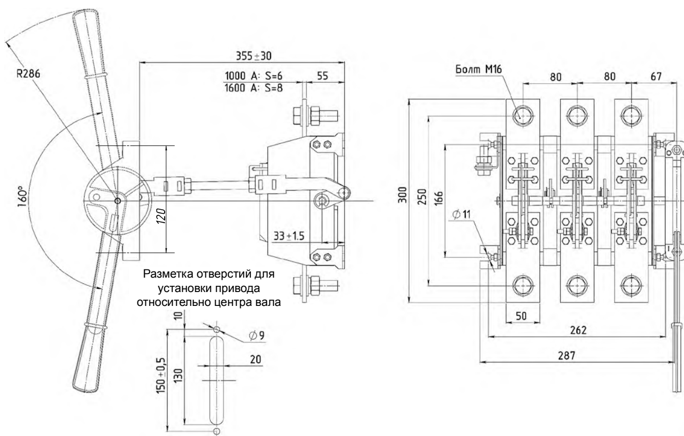
Рис. 16. Разъединитель PE19-41(43)-31140-00 УХЛЗ с передней смещенной рукояткой
