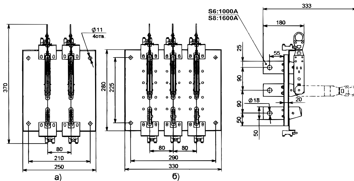
Рис. 41. Разъединитель PE19 на два направления с рукояткой для пополюсного оперирования, на изоляционной плите
