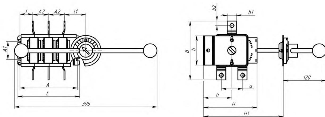
Рис. 17. Выключатель-разъединитель на два направления трехполюсный с передней поворотной рукояткой
