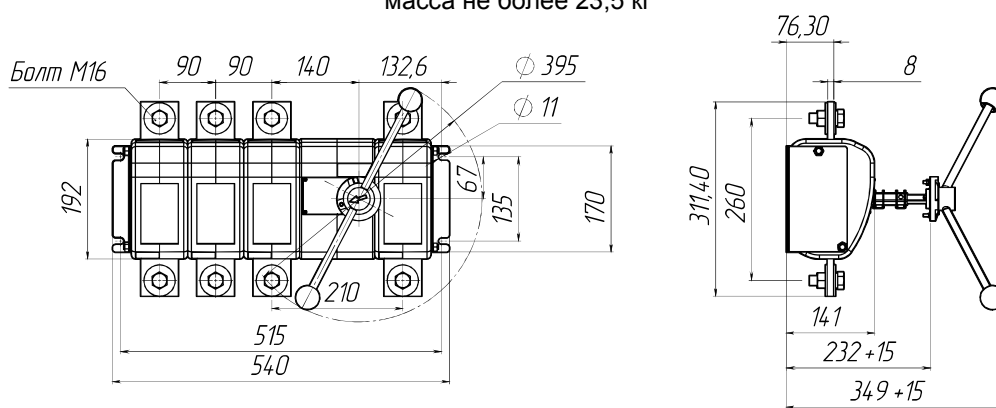
Рис. 8. ВНК-41-41130-32 УХЛЗ, масса не более 21,8 кг
