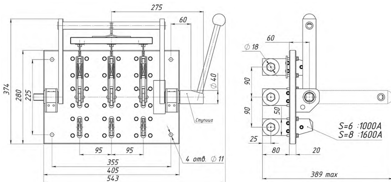
Рис.43. Разъединитель PE19 на два направления с боковой рукояткой, на изоляционной плите PE19-41(43)-72220-00 УХЛЗ, и/п
