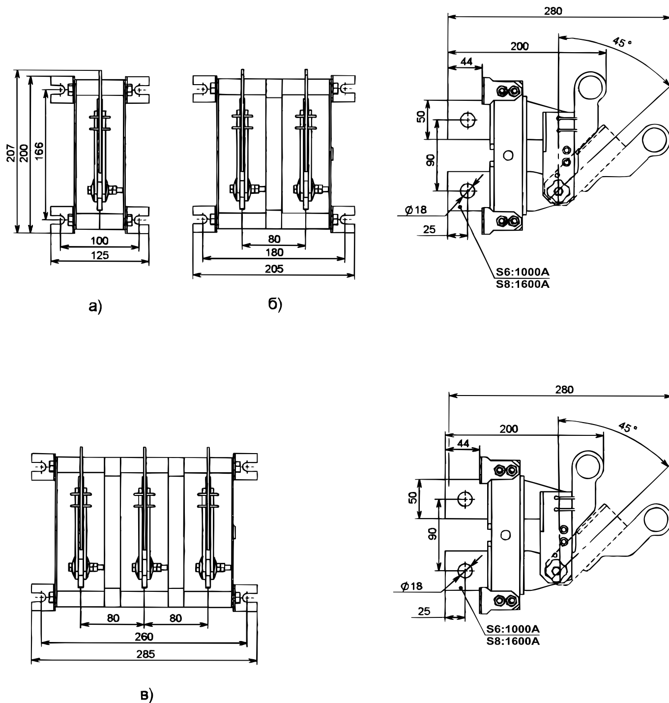
Рис. 24. Разъединитель PE19 с рычагом для пополюсного оперирования штангой, заднего присоединения шин а) PE19-41(43)-12260-00 УХЛЗ; б) PE19-41(43)-22260-00 УХЛЗ; в) PE19-41(43)-32260-00 УХЛЗ
