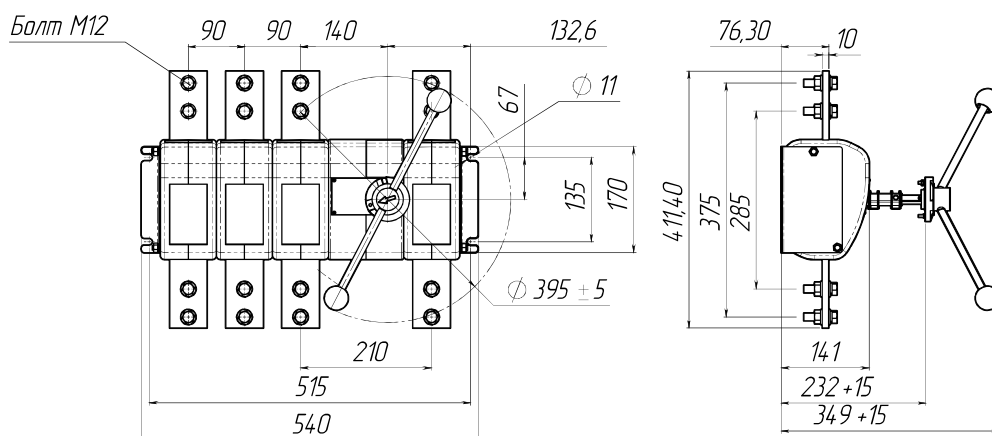
Рис. 7. ВНК-43-41130-32 УХЛЗ, масса не более 23,5 кг
