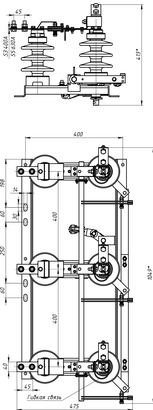
Рис. 2. Разъединитель РЛНД1.1-10II/400(630) – УХЛ1, масса не более 40,1 кг
