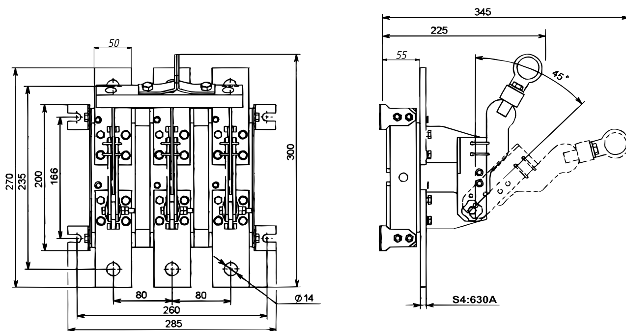
Рис. 10. Разъединитель РЕ19-39-31190-00 УХЛ3 с центральным рычагом для управления штангой
