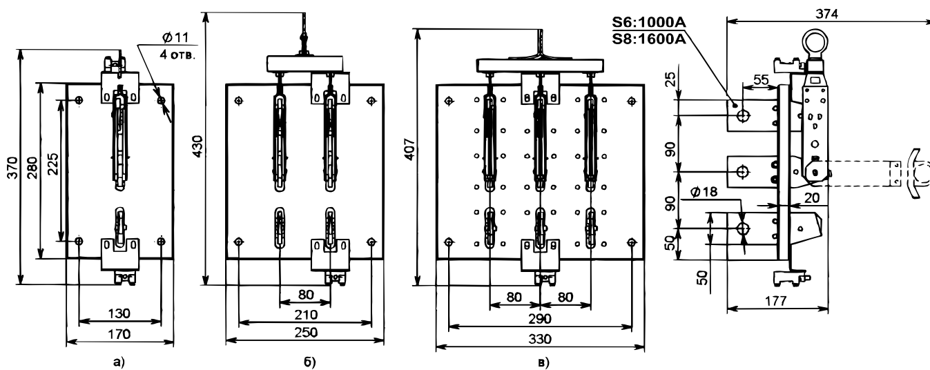
Рис. 39. Разъединитель PE19 на два направления с центральной рукояткой, на изоляционной плите а) PE19-41(43)-52211-00 УХЛЗ, и/п; б) PE19-41(43)-62211-00 УХЛЗ, и/п; в) PE19-41(43)-72211-00 УХЛЗ, и/п
