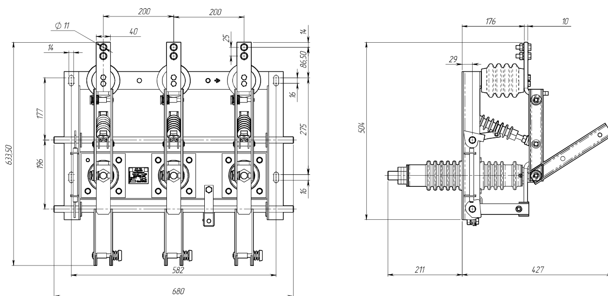
Рис. 8. Разъединитель внутренней установки типа РВФЗ-10/1000-II-II У2 с заземляющими ножами со стороны шарнирных контактов, масса не более 39 кг
