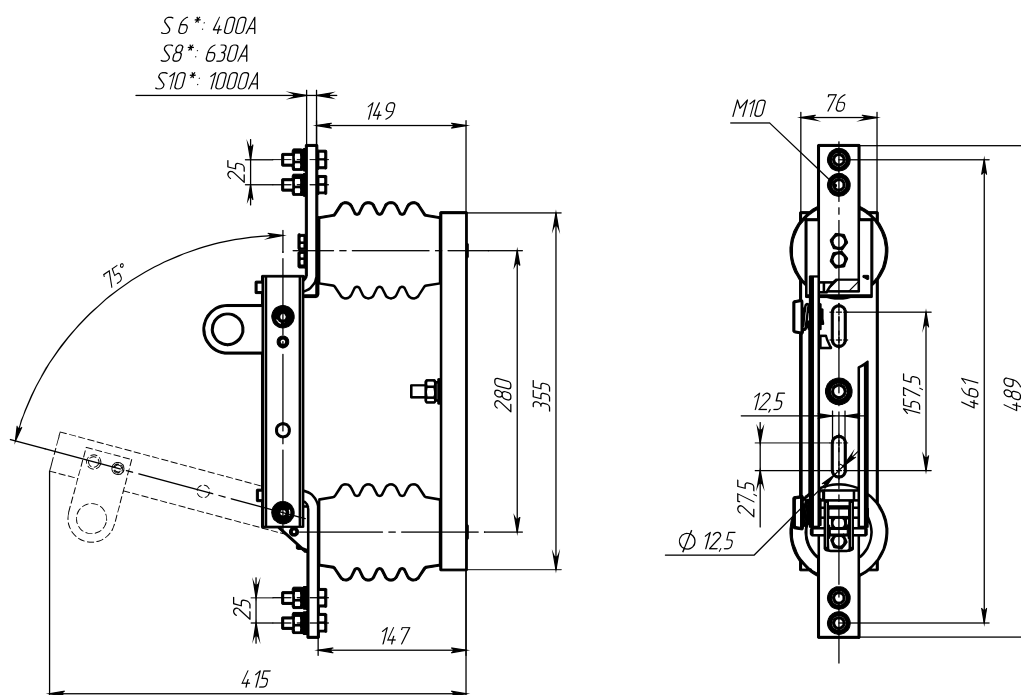
Рис. 9. Разъединитель внутренней установки типа РВЗ-10/630-III У2 с микропереключателем с заземляющими ножами с двух сторон, масса не более 30,5 кг
