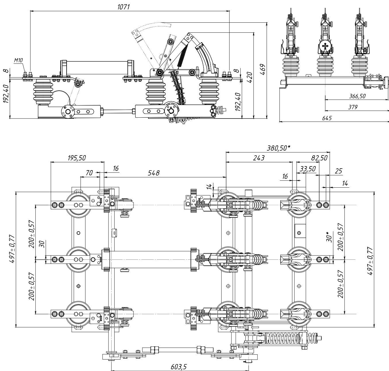
Рис. 3. Выключатель нагрузки автогазовый типа ВНАП-10/630-20-ІІз ПТ 1.2 У2, масса не более 46,5 кг
