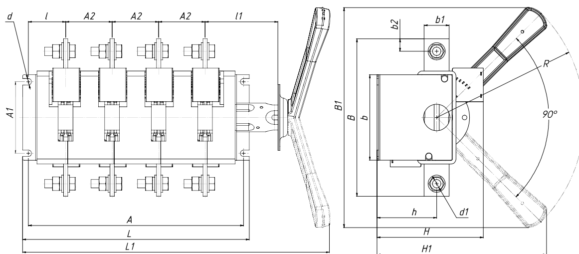
Рис. 19. Выключатель-разъединитель на одно направление 4-полюсный с боковой смещенной рукояткой
