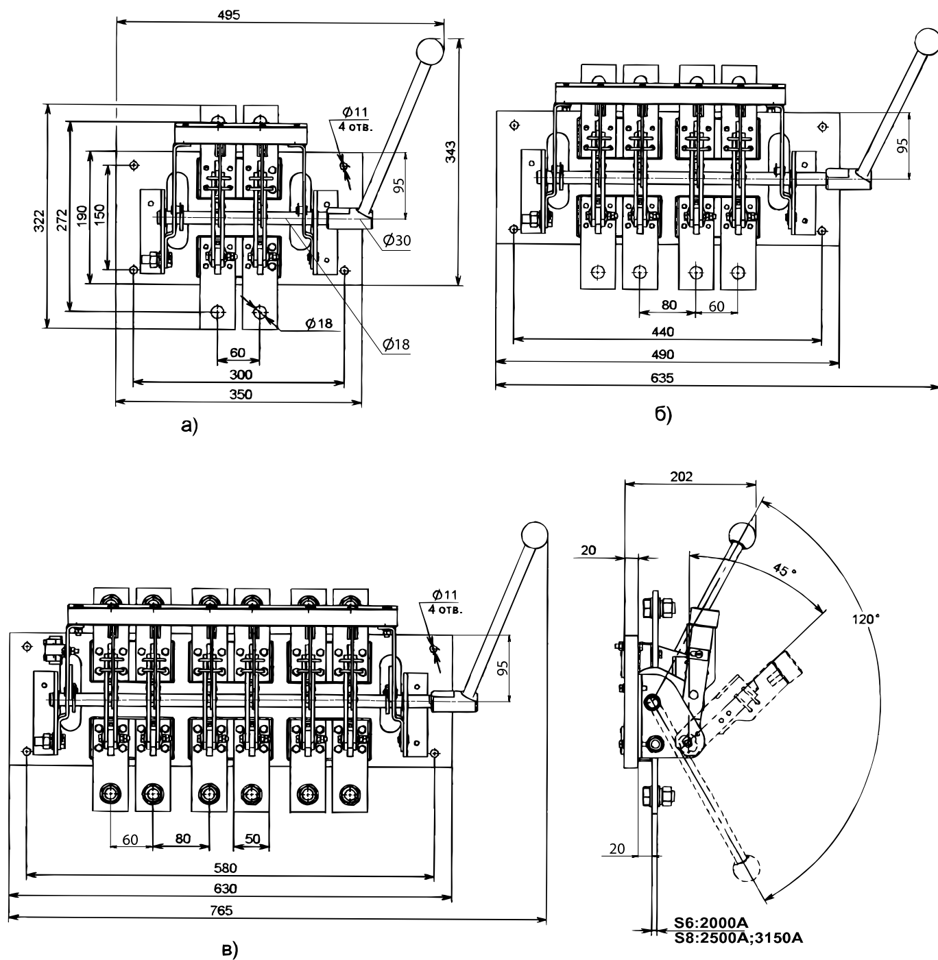
Рис. 51. Разъединитель PE19 с боковой рукояткой, на изоляционной плите а) PE19-44(45, 46)-11120-00 УХЛЗ, и/п; б) PE19-44(45, 46)-21120-00 УХЛЗ, и/п; в) PE19-44(45, 46)-31120-00 УХЛЗ, и/п
