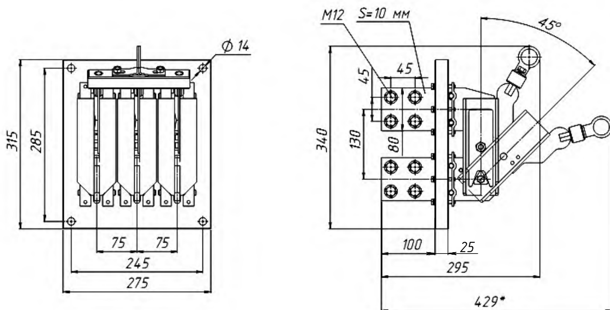
Рис. 56. Разъединитель PE19 с центральным рычагом для управления штангой, на изоляционной плите PE19-49-12290-00 УХЛЗ, и/п
