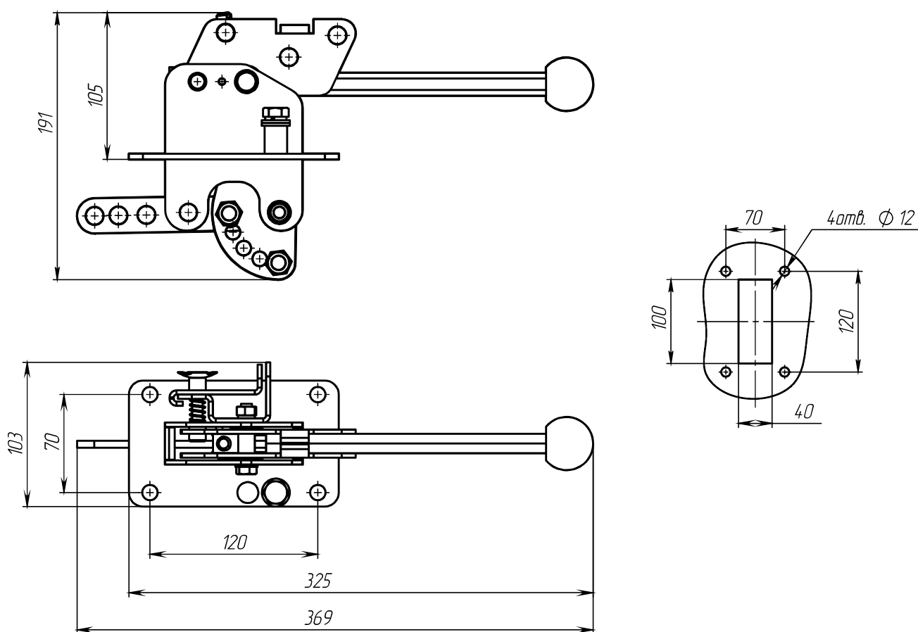
Рис.12. Привод ПР-10, масса не более 2,5 кг
