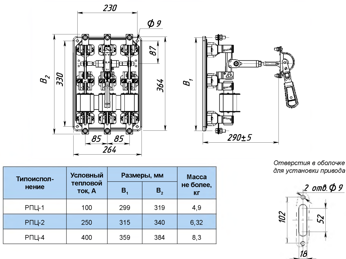
Рис. 5. Разъединители-предохранители с центральным приводом на токи 100 А, 250 А и 400 А
