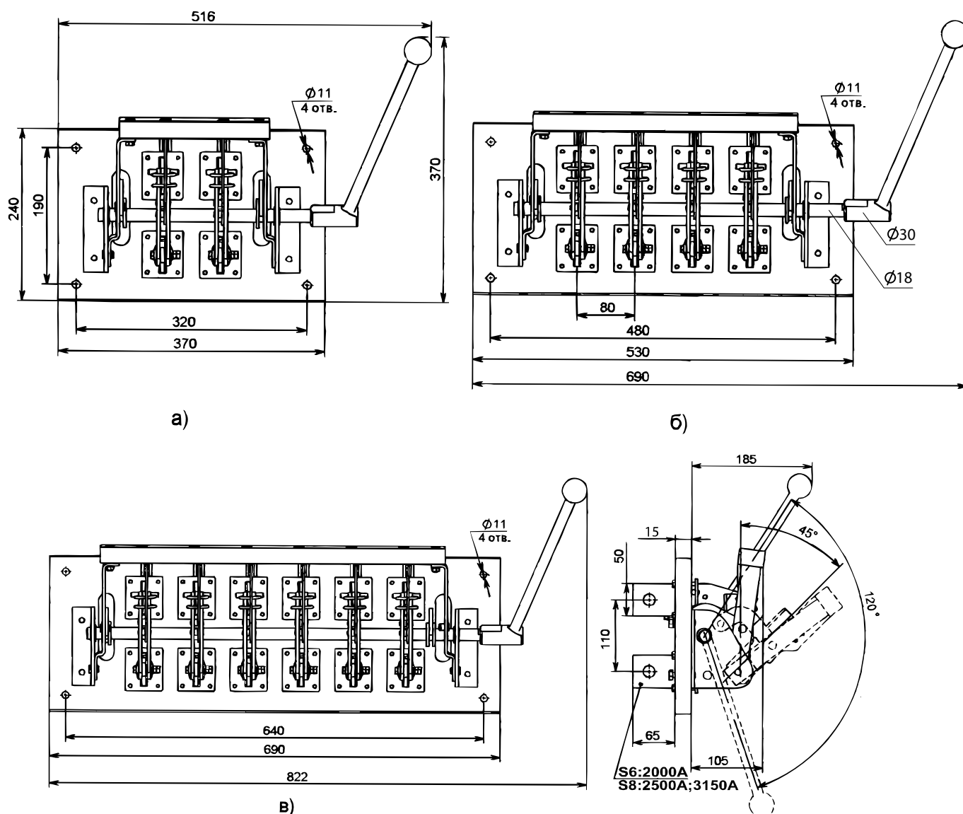
Рис. 52. Разъединитель PE19 с боковой рукояткой, заднего присоединения шин, на изоляционной плите а) PE19-44(45, 46)-12220-00 УХЛЗ, и/п; б) PE19-44(45, 46)-22220-00 УХЛЗ, и/п; в) PE19-44(45, 46)-32220-00 УХЛЗ, и/п
