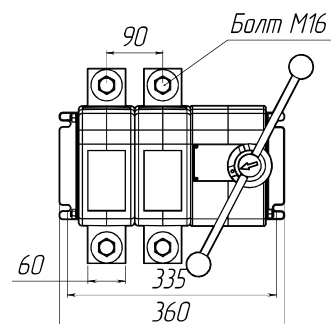
Рис. 12. ВНК-41-21130-32 УХЛЗ, масса не более 13,2 кг
