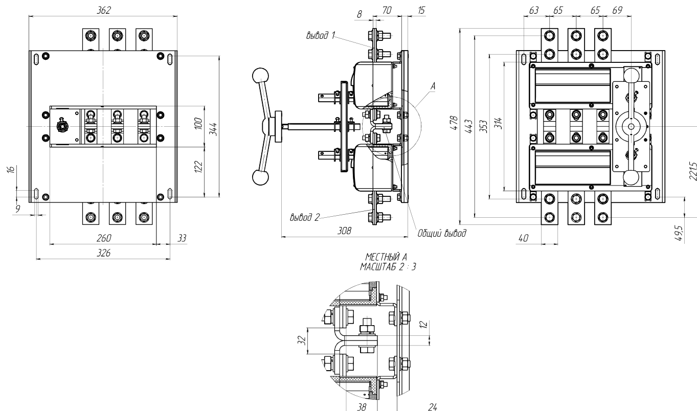
Рис. 6. Выключатель-разъединитель ВНК-39-71130-32 УХЛ3 на два направления, масса не более 14,5 кг
