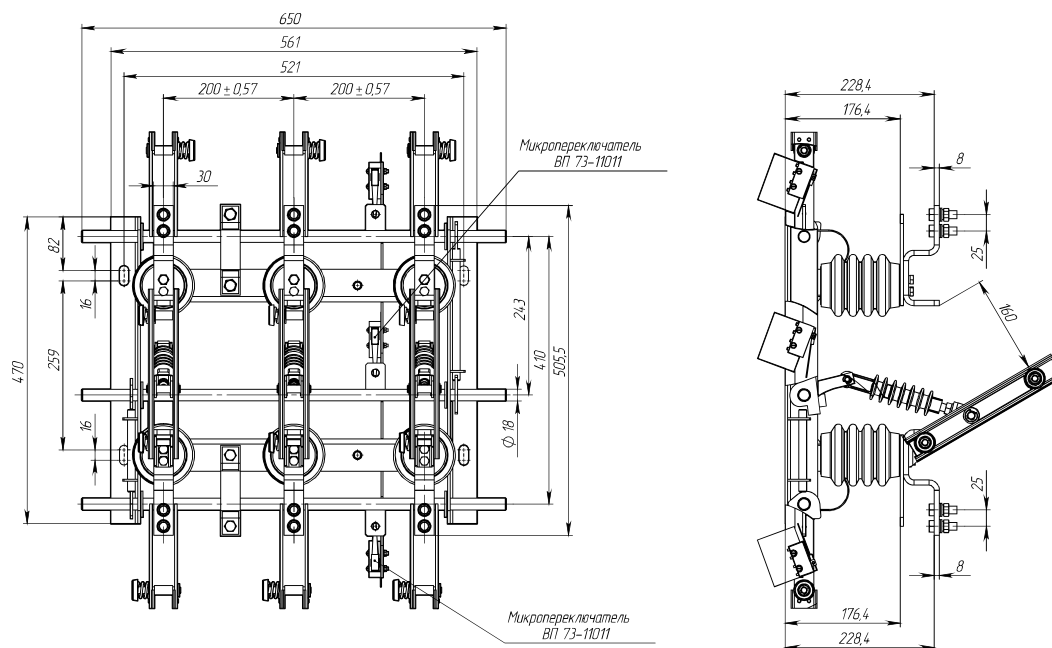
Рис. 9. Разъединитель внутренней установки типа РВЗ-10/630-III У2 с микропереключателем с заземляющими ножами с двух сторон, масса не более 30,5 кг
