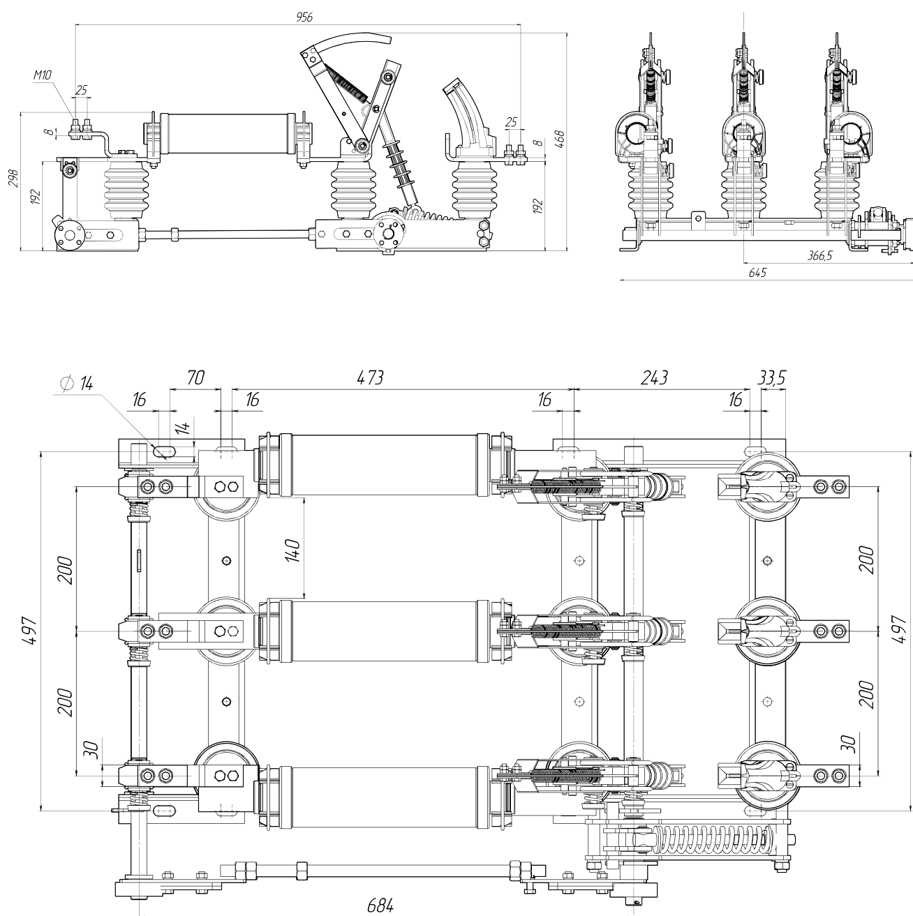
Рис. 11. Выключатель нагрузки автогазовый типа ВНАП-10/630-20-ІІз ПКТ-ВК У2, масса не более 49 кг
