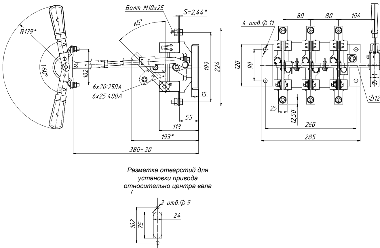
Рис. 9. Разъединитель РЕ19-35(37)-31140-00 УХЛ3 с передней смещенной рукояткой
