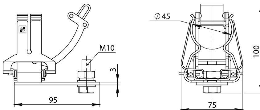
Рис. 2 исполнение-02 остальное см. рис. 1
