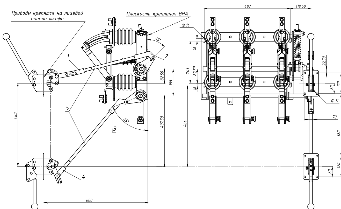
Рис. 27. Возможный монтаж выключателя нагрузки с приводом ПРБД-10.
