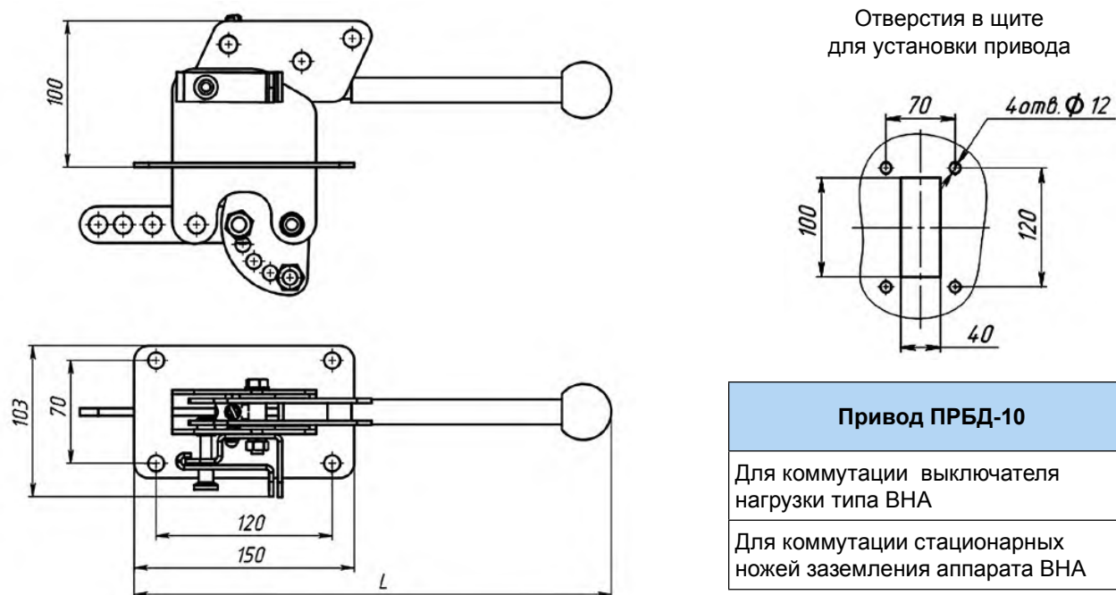
Рис. 26. Привод ПРБД-10
