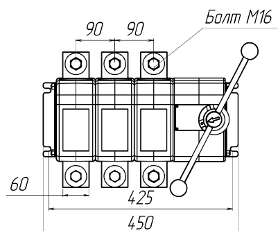
Рис. 10. ВНК-41-31130-32 УХЛЗ, масса не более 17,5 кг
