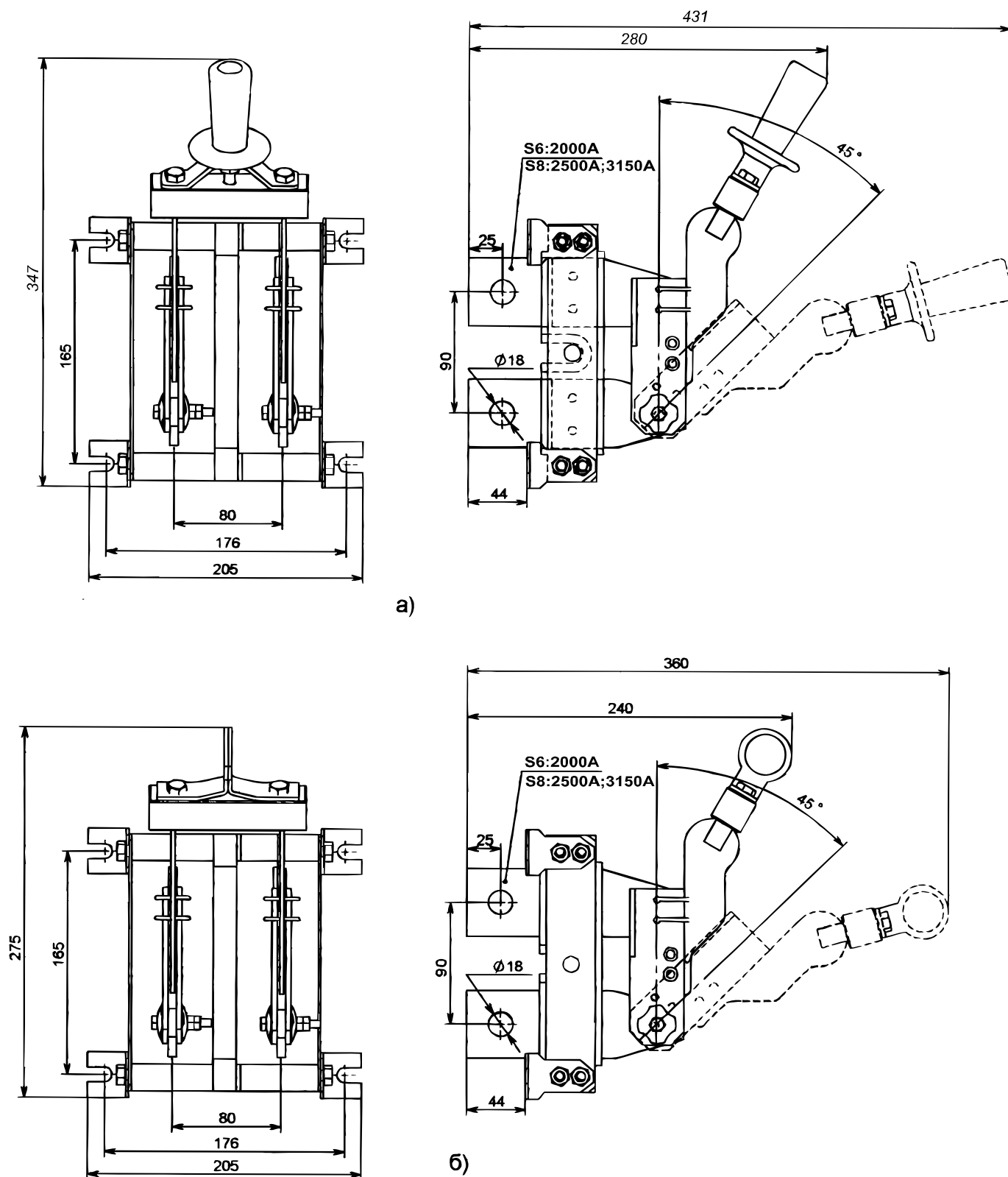
Рис. 46. Разъединитель PE19 однополюсный, заднего присоединения шин
