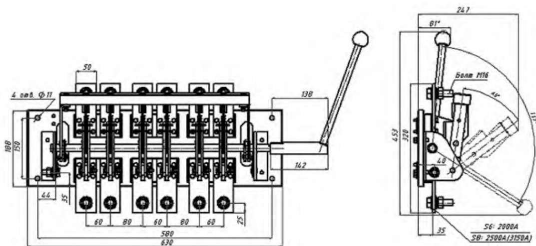
Рис. 53. Разъединитель PE19 с боковой смещенной рукояткой, на изоляционной плите PE19-44(45, 46)-31150-00 УХЛЗ, и/п
