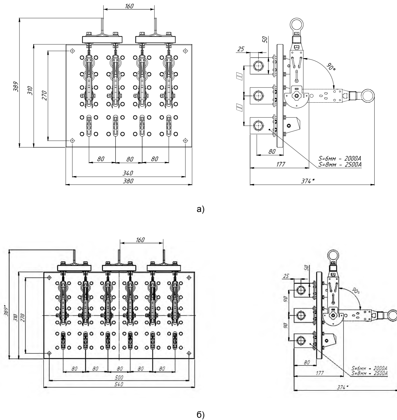
Рис. 54. Разъединитель РЕ19 на два направления с рычагом для пополюсного оперирования штангой, на изоляционной плите а) РЕ19-44(45, 46)-62260-00 УХЛЗ, и/п; б) РЕ19-44(45, 46)-72260-00 УХЛЗ, и/п
