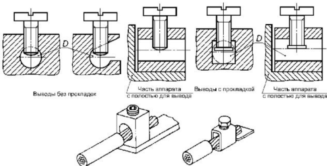
Выводы с прямой передачей давления
