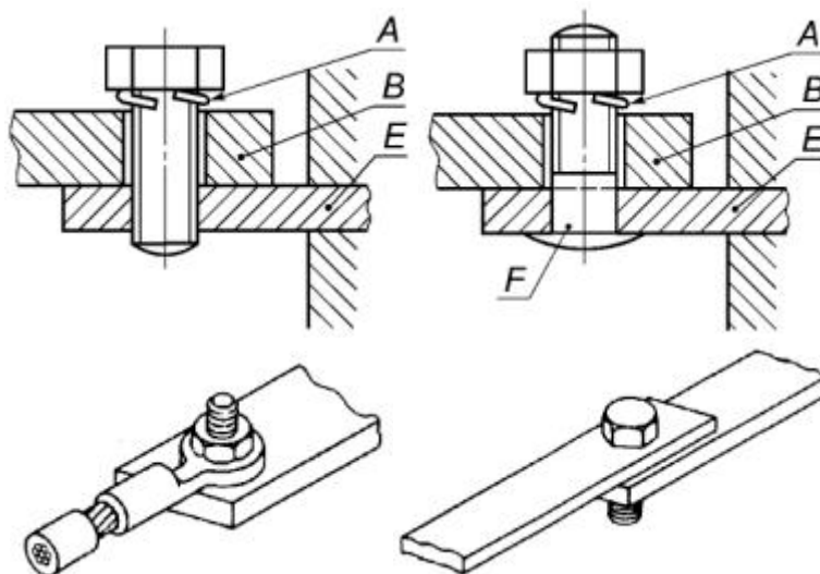
Рисунок D.4 - Выводы с прокладками
