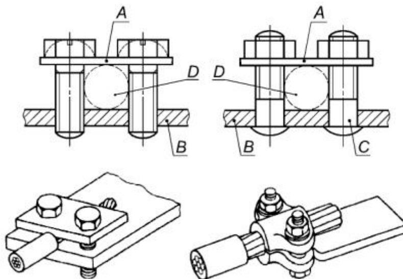
Рисунок D.3 - Штифтовой вывод
