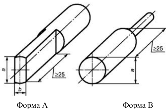
Рисунок 2 - Щупы формы А и В (см. 8.2.4.5.2 и таблицу 7 )
