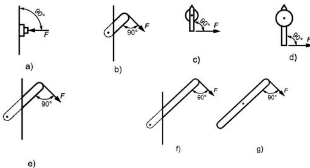
Рисунок 16 - Испытательное усилие, прикладываемое к органу управления (см. 8.2.5.2.1 и таблицу 17 )
