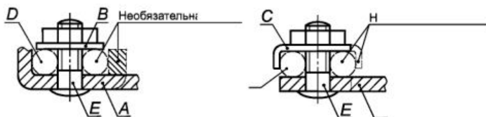
Рисунок D.2 - Выводы с отверстиями
