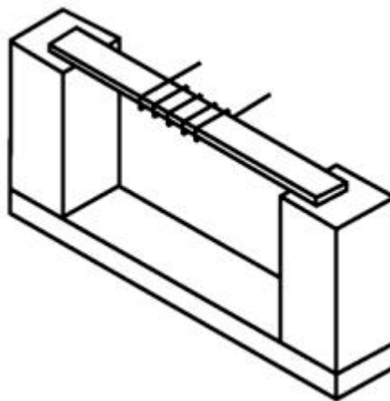
Рисунок М.1 - Приспособление для испытания материала нагретой проволокой
