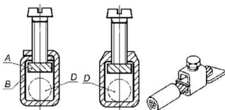
Выводы с непрямой передачей давления
