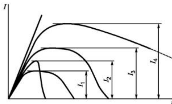
Рисунок 15 - Определение ожидаемого тока отключения после проведения первой калибровки при токе, меньшем номинальной отключающей способности (см. 8.3.4.1.8 , перечисление б)
