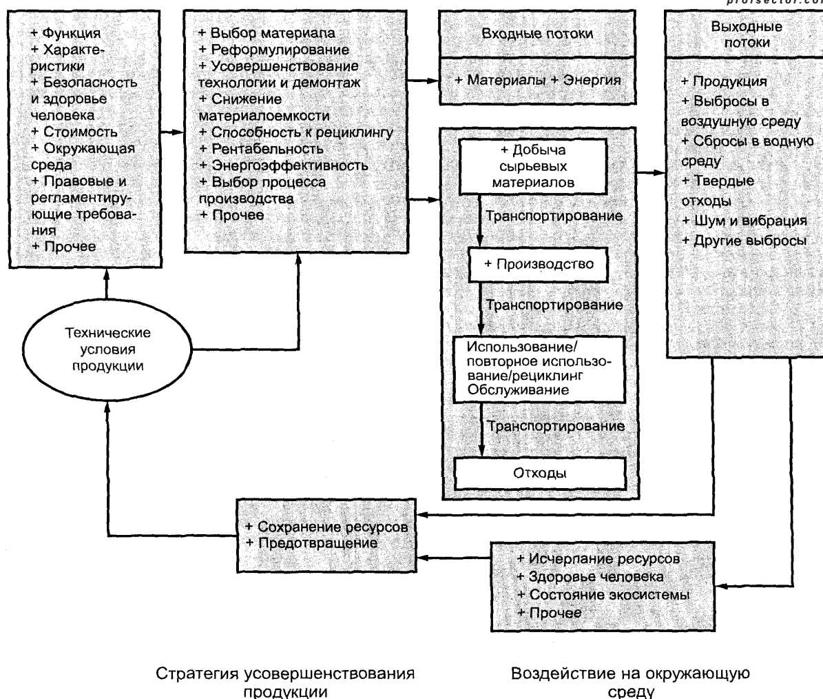
Рисунок О.1 - Экологические аспекты продукции на протяжении ее жизненного цикла
