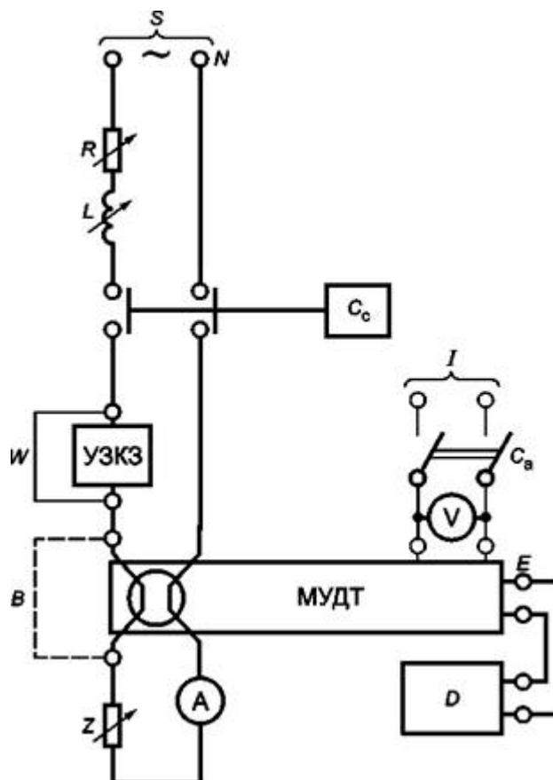
Рисунок М.17 - Испытательная цепь для проверки поведения МУДТ с отдельным датчиком в условиях короткого замыкания
