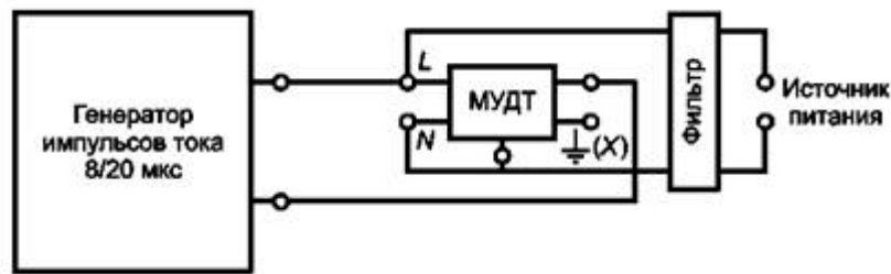
с) МУДТ выводного типа
