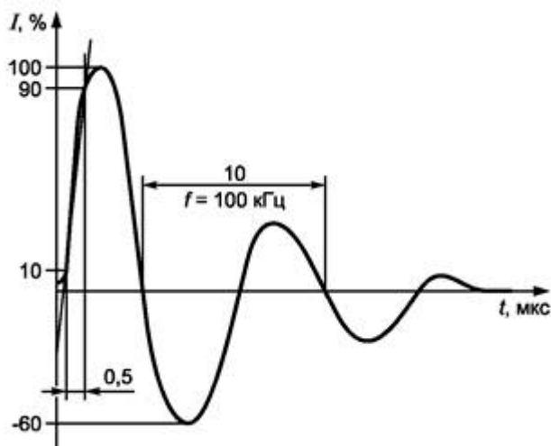
Рисунок В.4 - Волна тока 0,5 мкс/100 кГц
