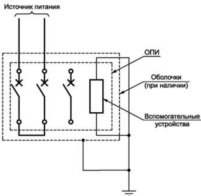
Рисунок F.2 - Испытательная цепь для проверки устойчивости к низкочастотным электромагнитным помехам и испытаний на помехоэмиссию по F.4.1.3 , F.4.2 , F.4.3 , F.4.6 , F.4.7.1 , F.5.4 и F.6.2 для двух фазных полюсов, соединенных последовательно
