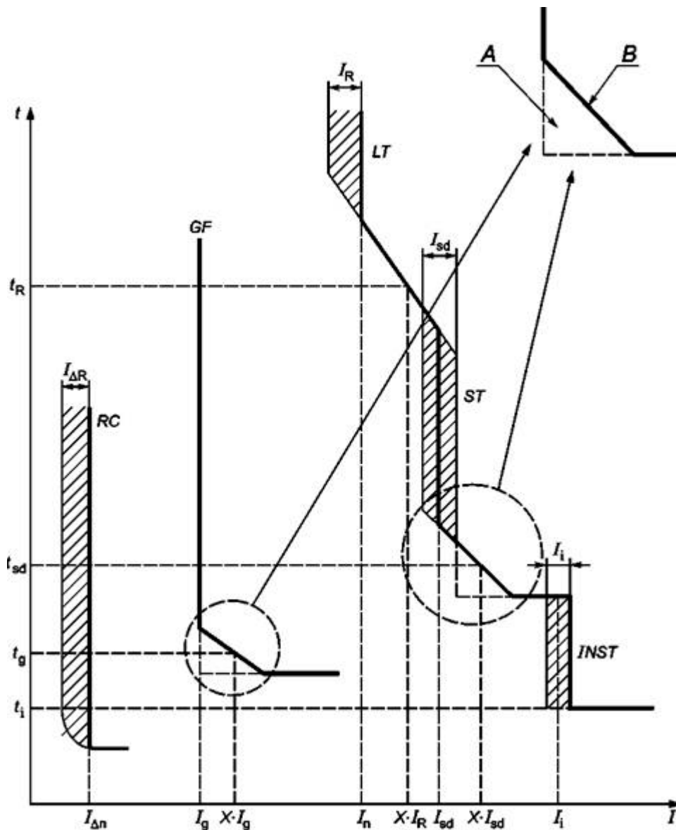
Рисунок К.1 - Соответствие символов характеристикам расцепления
