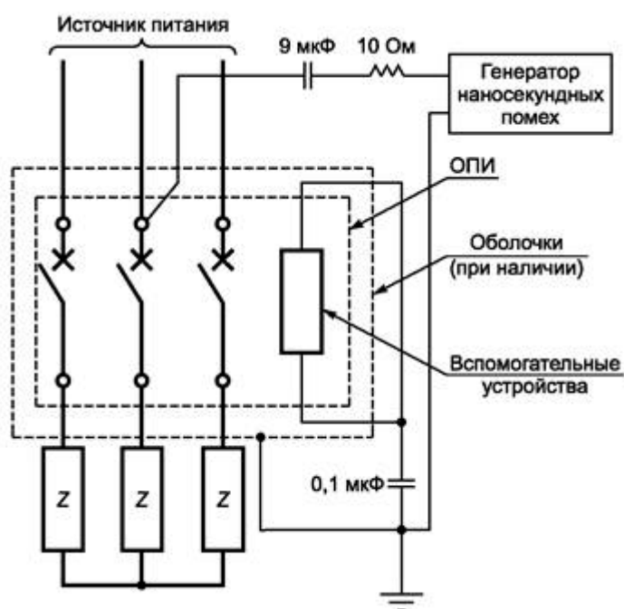
Рисунок F.10 - Испытательная цепь для проверки влияния скачков напряжения/тока в главной цепи (между фазой и землей) по F.4.5 для трех фазных полюсов, соединенных последовательно
