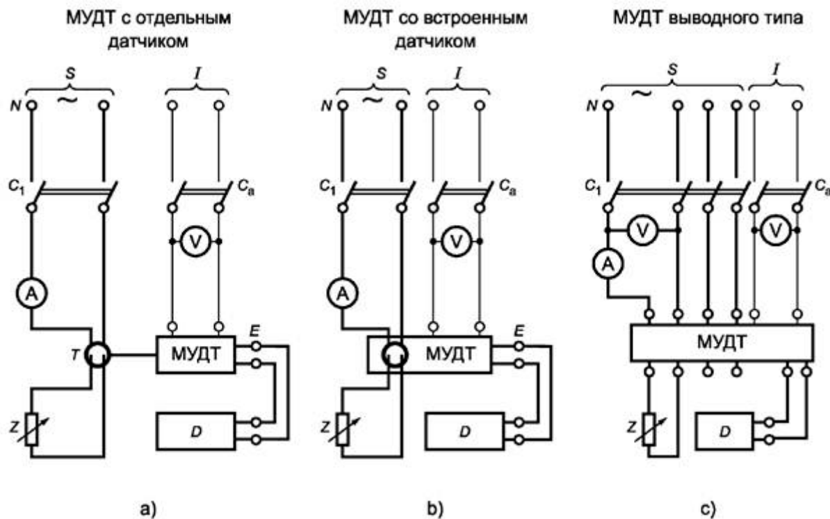
Рисунок М.3 - Испытательные цепи для проверки срабатывания в случае неожиданно возникающего дифференциального тока (без отключающего устройства)
