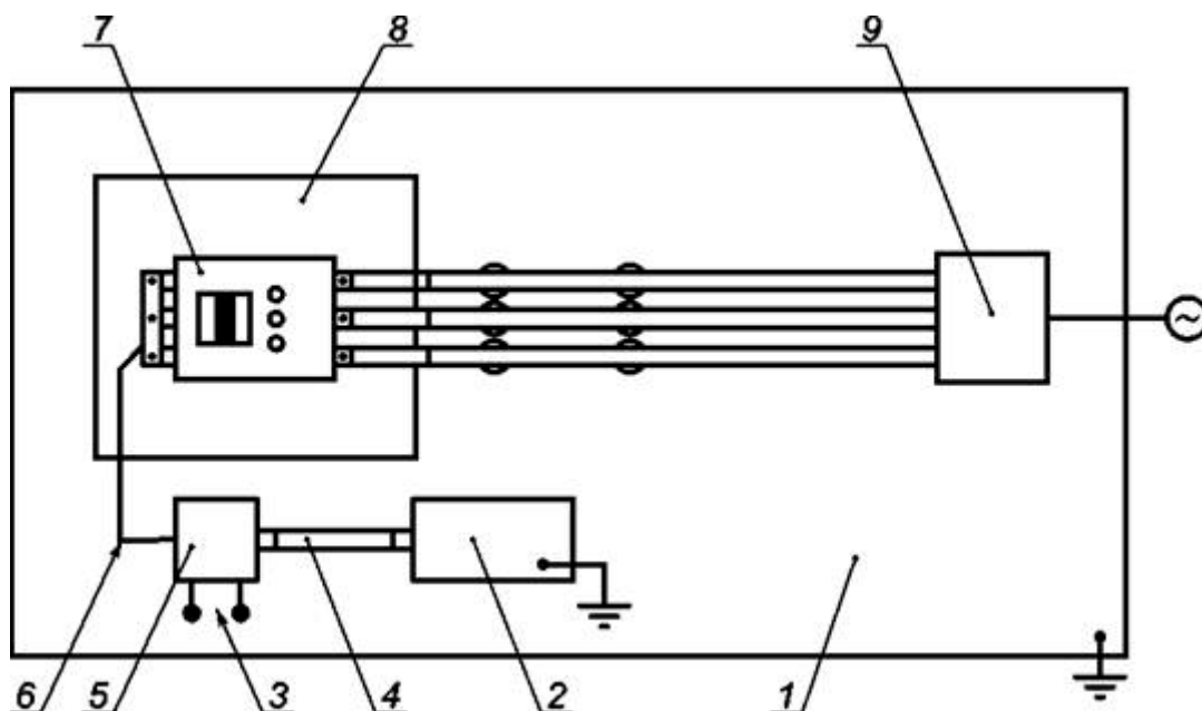
Рисунок F.22 - Схема соединений для проверки устойчивости к кондуктивным низкочастотным помехам, наведенным радиочастотными полями, для трех фазных полюсов, соединенных последовательно
