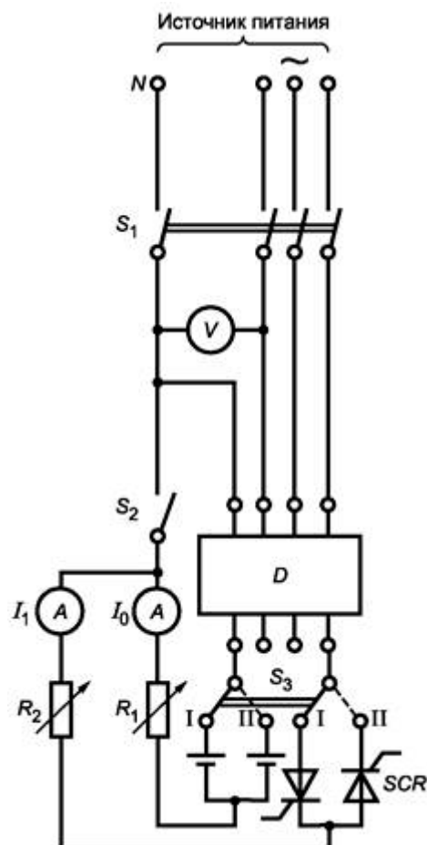
S_1 - многополюсный выключатель; S_2 - однополюсный выключатель; S_3 - переключатель на два направления; V - вольтметр; A - амперметр измерения действующего значения; R_1 , R_2 - регулировочные резисторы; D - испытуемый АВДТ; SCR - тиристоры; N - нейтраль
