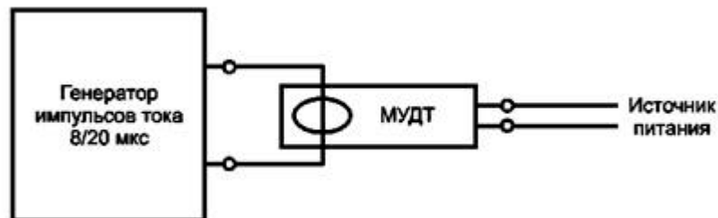
b) МУДТ со встроенным датчиком
