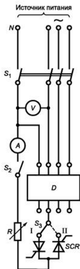
S_1 - многополюсный выключатель; S_2 - однополюсный выключатель; S_3 - переключатель на два направления; V - вольтметр; A - амперметр измерения действующего значения; R - регулировочный резистор; D - испытуемый АВДТ; SCR - тиристоры; N - нейтраль
