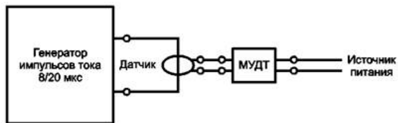
a) МУДТ с отдельным датчиком
