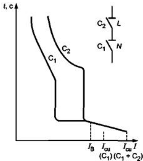
Рисунок D.2 - Полная селективность между двумя выключателями
