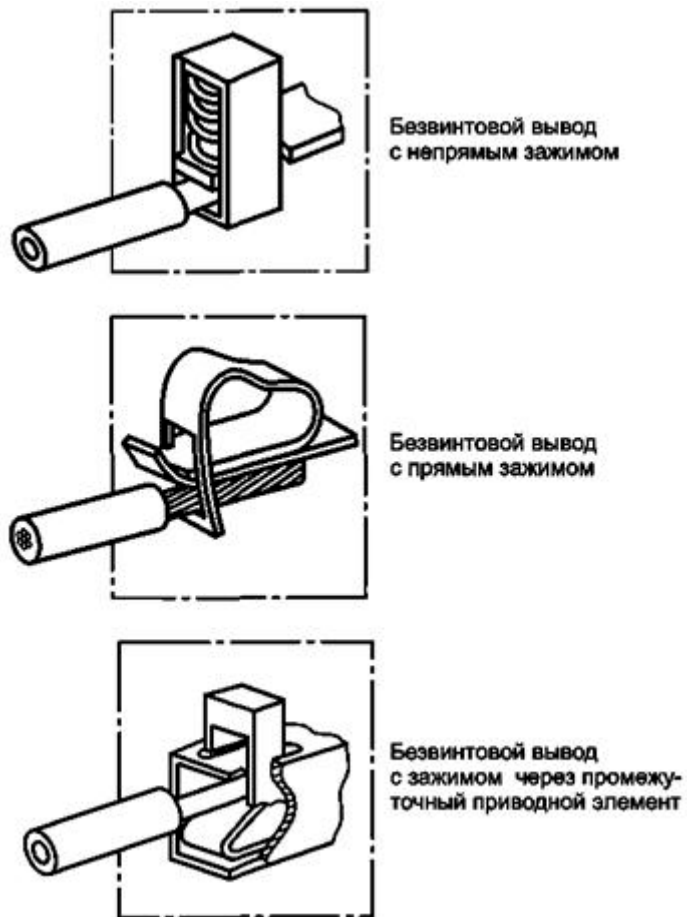
Рисунок J.2 - Примеры безвинтовых выводов
