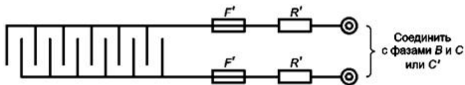
Рисунок Н.3 - Цепь решетки
