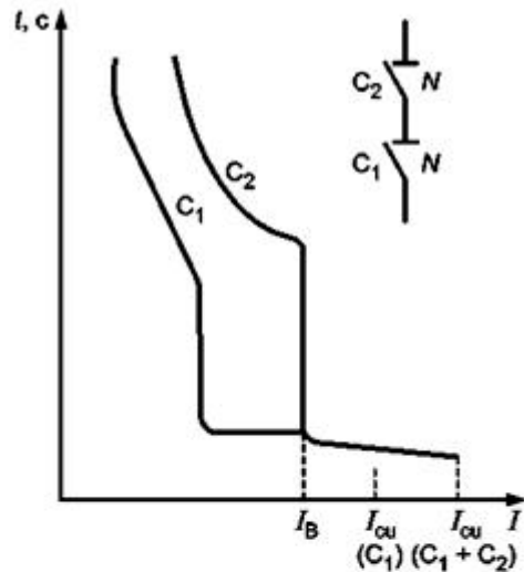
Рисунок D.2 - Полная селективность между двумя выключателями
