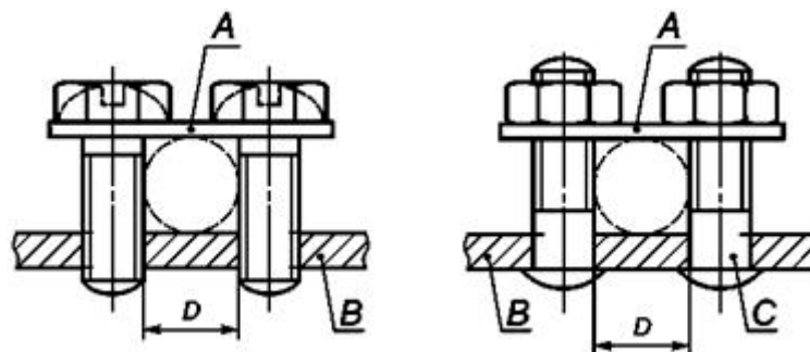
Рисунок F.2 - Пример винтовых и штыревых выводов
