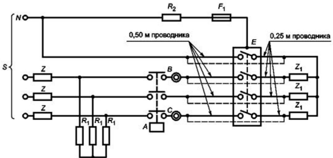
Рисунок 6 - Четырехполюсный автоматический выключатель
