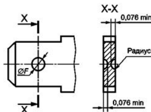
Рисунок К.2 - Размеры штыревых контактов (штекеров)
