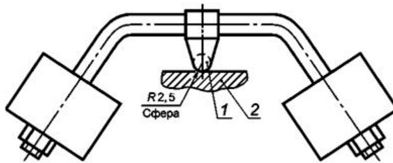
Рисунок 16 - Установка для испытаний давлением шарика
