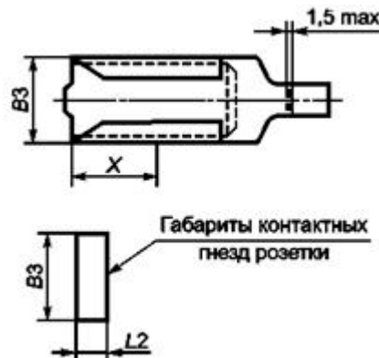
Рисунок К.5 - Размеры отверстий для фиксации
