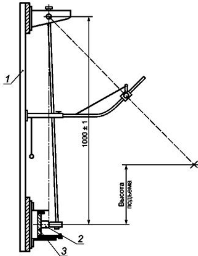
Рисунок 10 - Устройство для испытания на механический удар (см. 9.13.2 )
