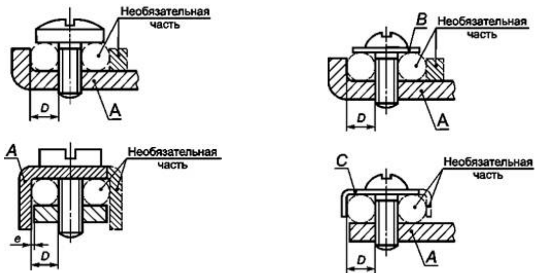
Рисунок ИС.1 - Примеры столбчатых выводов
