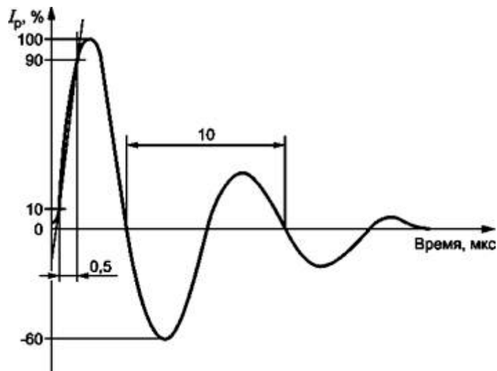
Рисунок 23 - Ток звенящей волны 0,5 мкс/100 кГц
