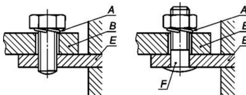
A - запорное устройство; B - кабельный наконечник или шина; E - неподвижная часть; F - штырь
