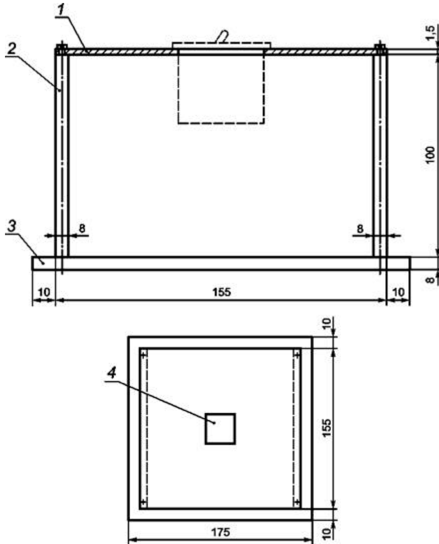
Рисунок 15 - Пример монтажа АДТ открытого исполнения для испытания на механический удар (9.13.2.1)
