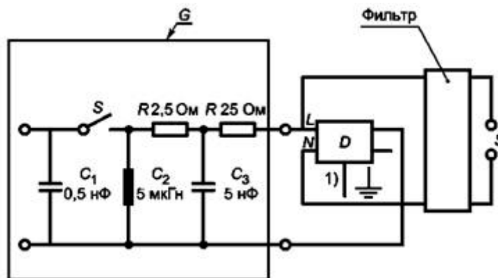
Рисунок 23 - Ток звенящей волны 0,5 мкс/100 кГц
