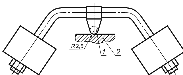
Установка для испытаний на твердость по Бринеллю
