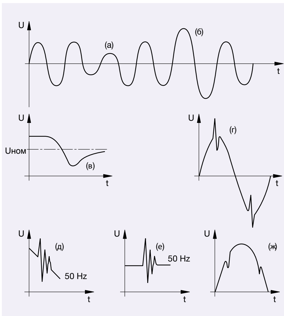
Рис. 1.2: Типы изменения амплитуды напряжения
