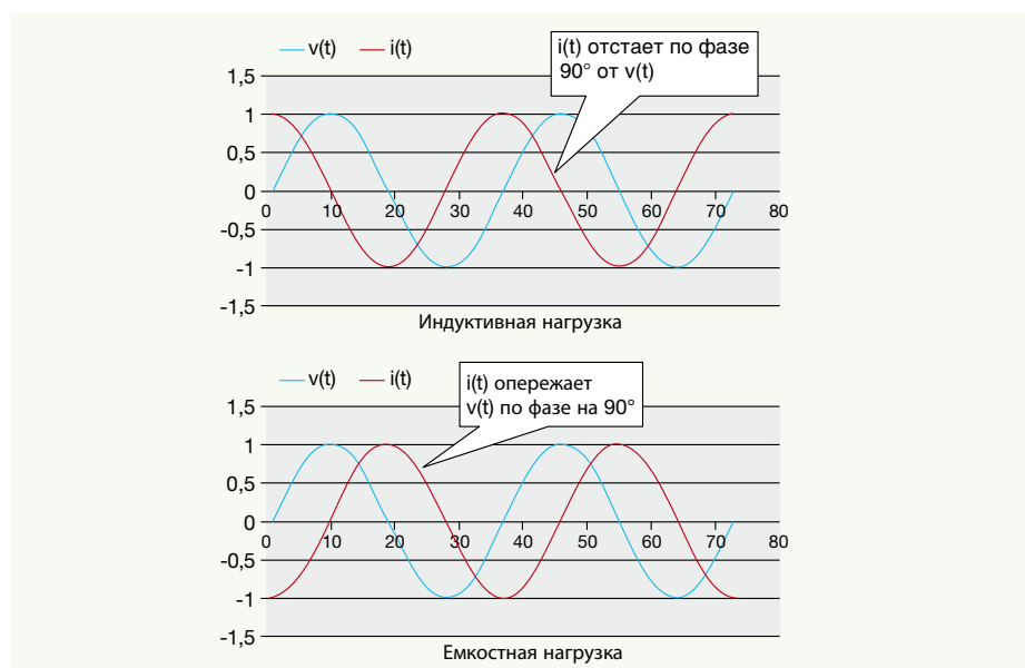
Рис. 1. Линейная зависимость между синусоидальным током I(t) и напряжением V(t)
