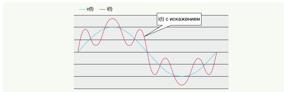
Рис. 2. Несинусоидальная зависимость i(t) от U(t) в нелинейной нагрузке
