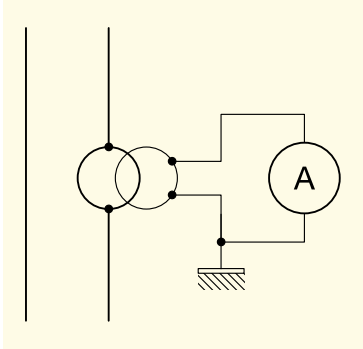
Рис. 4.1. Электрическая схема токового трансформатора
