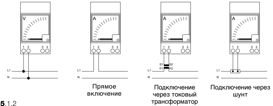
Рис. 5.1. Подключение аналоговых приборов различными способами (прямое, через токовый трансформатор и через шунт)
