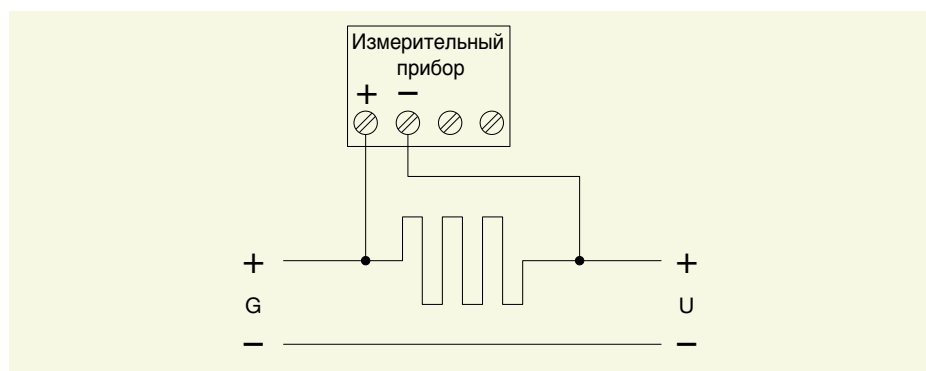
Рис. 5.14. Способ установки шунта в измерительную цепь
