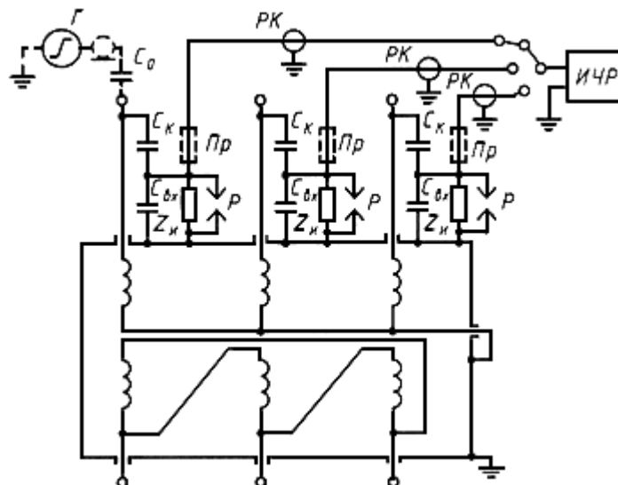
Принципиальная схема установки для измерений характеристик частичных разрядов
