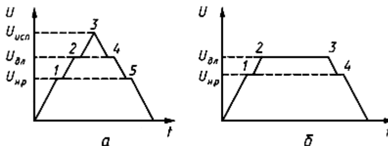
Графики изменения напряжения во времени при испытании нормированными испытательными одноминутным (а) и длительным (б) напряжениями
