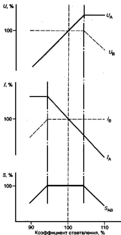
Рисунок 3 - Комбинированное регулирование напряжения (режим в)
