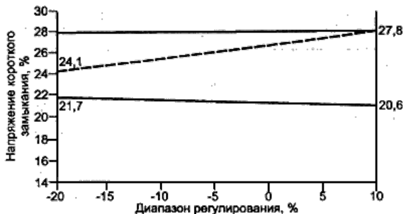
Рисунок В.1 - Диапазон изменения напряжения короткого замыкания
