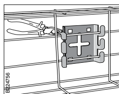
Для повышения прочности крепления достаточно загнуть выступы консоли вокруг прутьев лотка.
