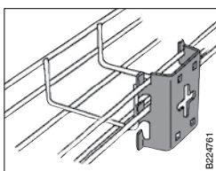
Для крепления лотка просто заведите его прутья за выступы консоли.
