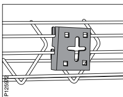
Крепление лотка под углом 45°.
