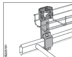
Крепление лотка к лестнице посредством B21 и консоли B4/B4 mini.
