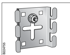
Консоль крепится к стене анкерным болтом через центральное отверстие или шурупами через угловые квадратные отверстия.
