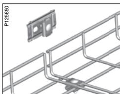
Комплект B52 до установки на лоток.
