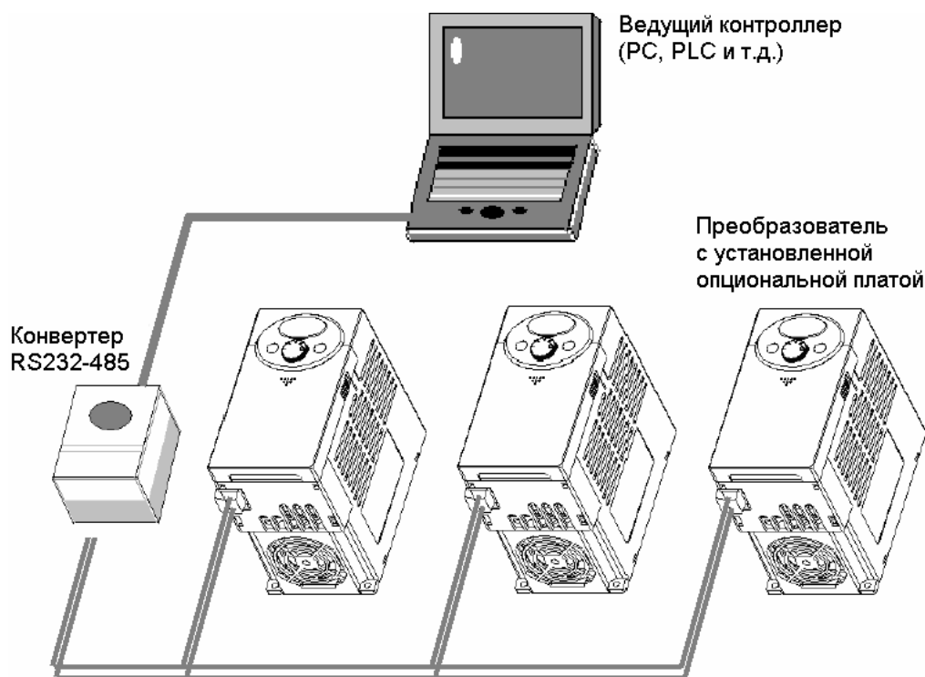
Рис. 2. Конфигурация системы
