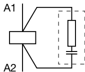
RC-цепь
