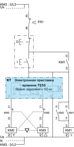
Схема цепи управления: дистанционный режим
