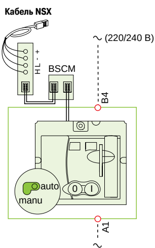
Коммуникационный мотор-редуктор (MTc) (1)
