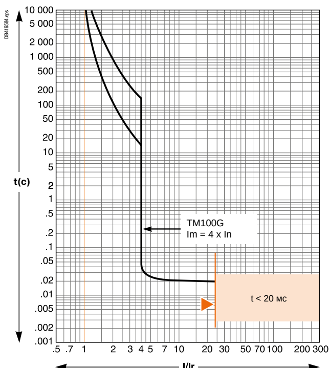
TMG100
