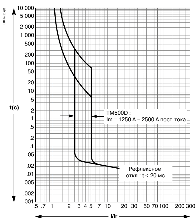
TM-DC 500
