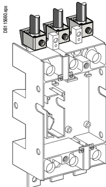
Одиная клемма
