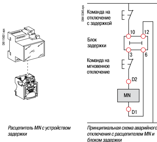
Расцепитель напряжения MN
