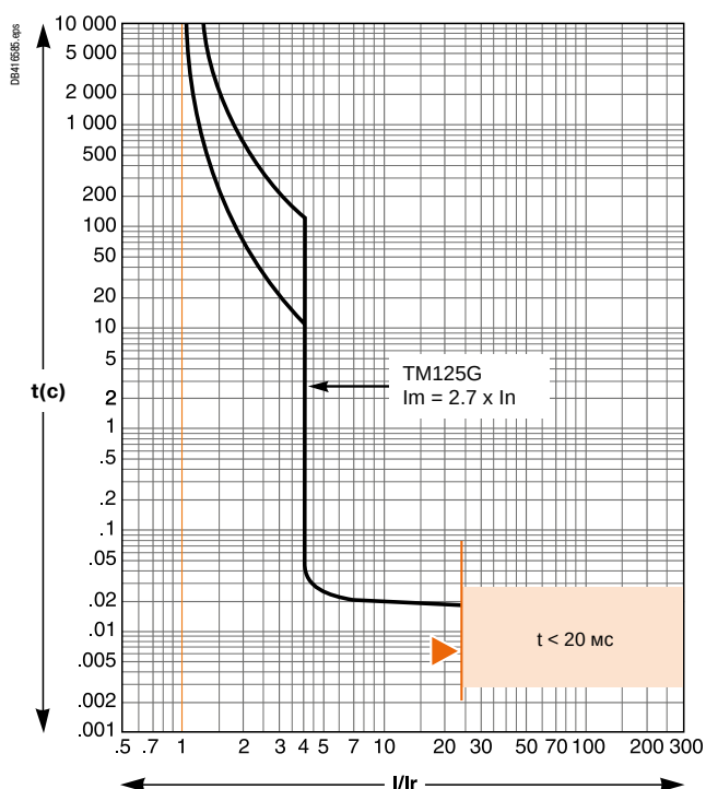
TMG125
