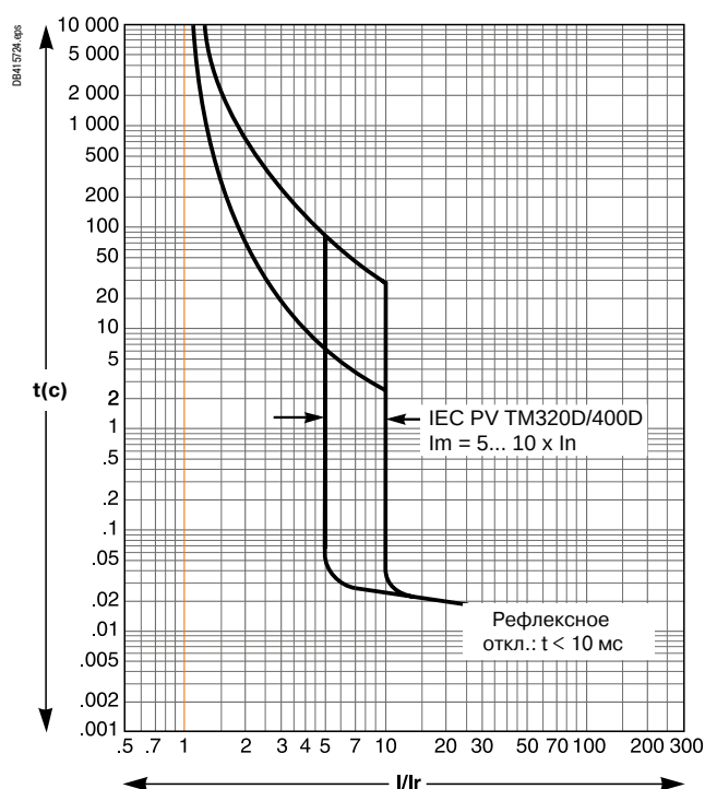
TM-DC 320 PV/ TM-DC 400 PV
