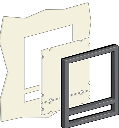
Рамка передней панели (CDP) с заглушкой
