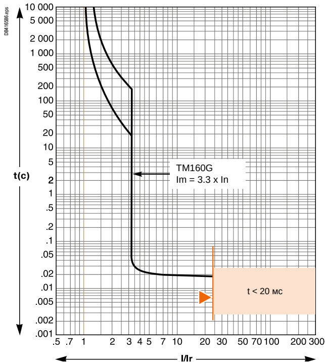
TMG160
