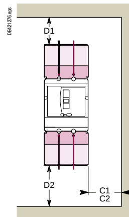
Устройства с длинными или короткими клеммными заглушками
