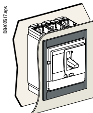
Рамка передней панели для рычага управления без доступа и с доступом к расцепителю
