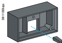
Тамбур и удлинитель для рычага управления, обеспечивающие степень защиты IP4 в положениях «вклено» и «выкачено»
