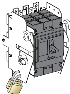
Блокировка шасси в положении «выкачено»
