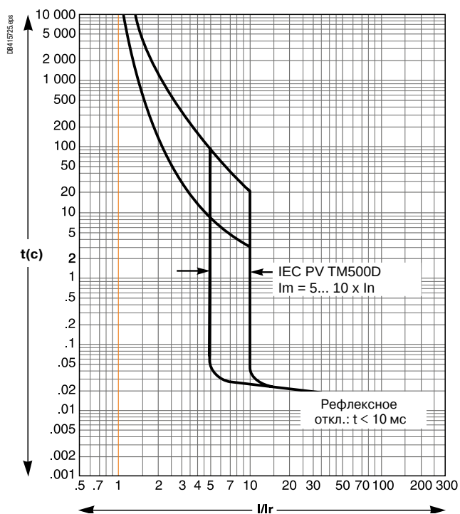
TM-DC 500 PV
