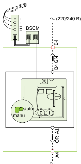
Коммуникационный мотор-редуктор (МТс) (1)
