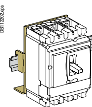
Монтаж на DIN-рейке (с адаптером)
