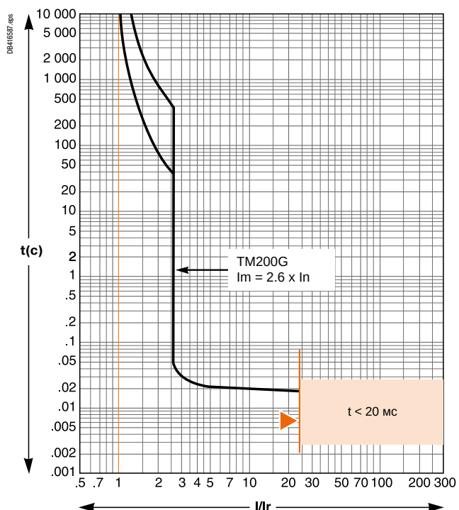
TMG200
