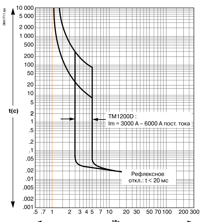
TM-DC 1200
