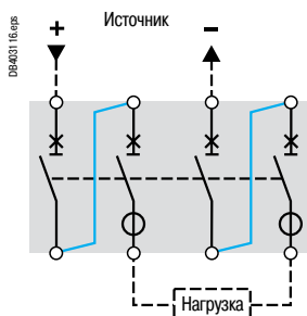
Masterpact NW20H DC, исполнение Е
