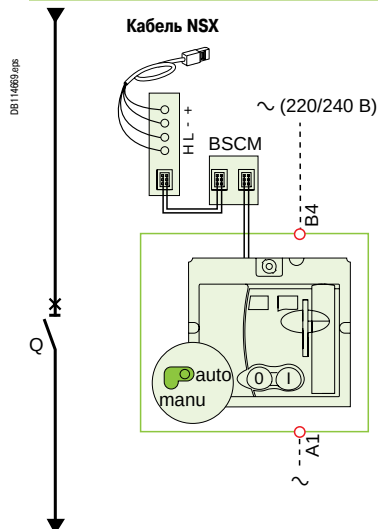
Принципиальная схема коммуникационного мотор-редуктора (МТ)
