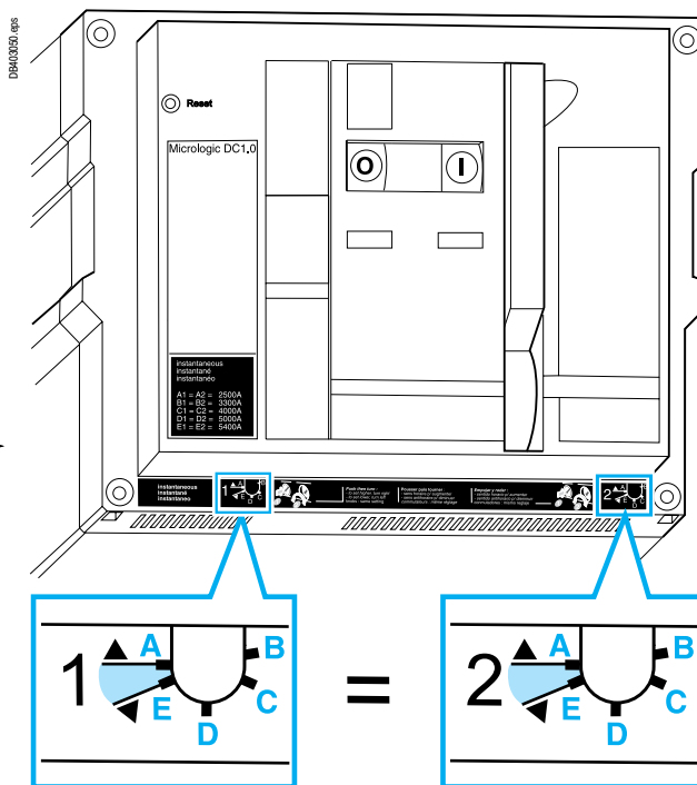
Две одинаковые настройки
