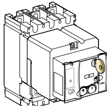
Блокировка мотор-редуктора с помощью встроенного или навесного замка
