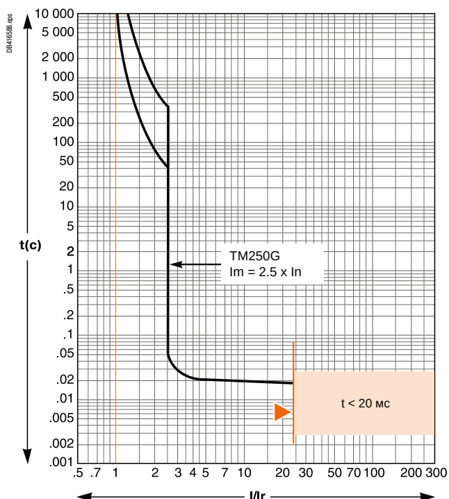
TMG250
