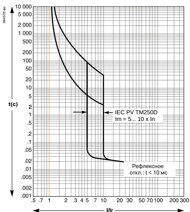
TM-DC 250 PV
