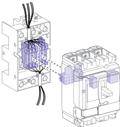
Втычной /выдвижной автоматический выключатель Compact NSX DC
