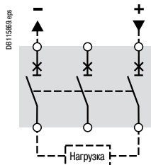
Выбор 3: Compact NSX250 DC3P с 2 подключенными полюсами
