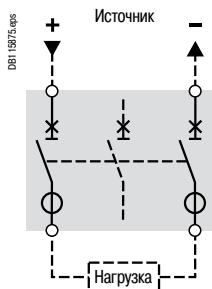
Masterpact NW1 0N DC, исполнение С
