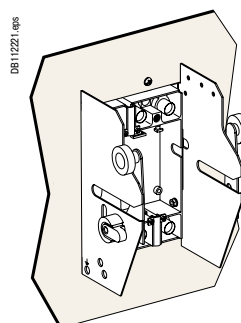
Монтаж в вырез передней панели
