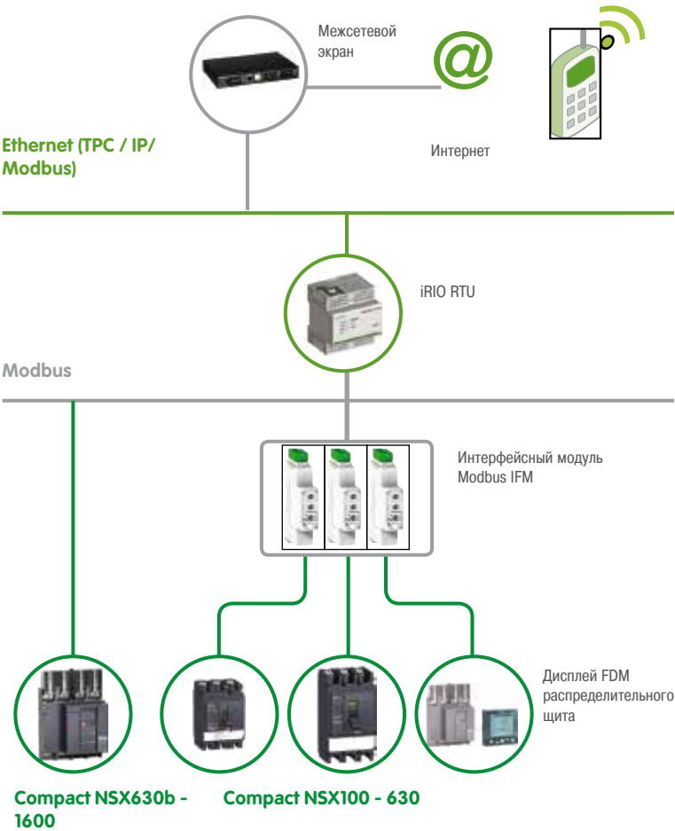
iRIO RTU
