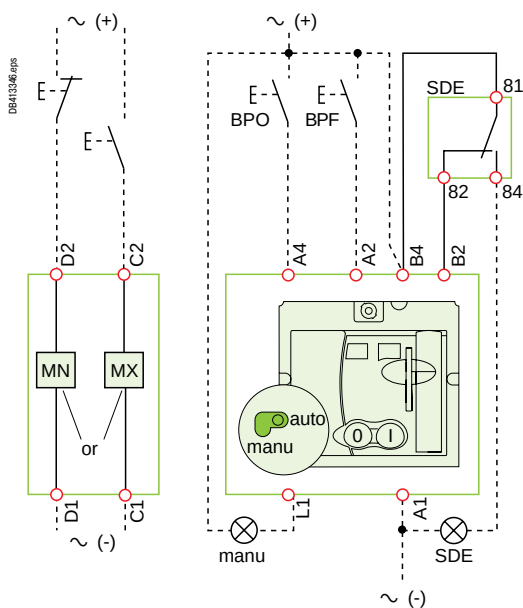
Мотор-редуктор (MT)
