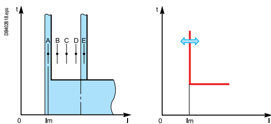
Значение уставки мгновенного срабатывания
