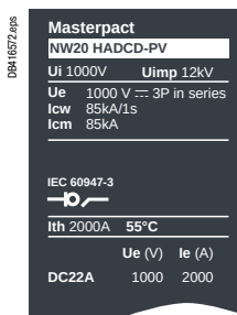
Заводская табличка аппарата NW20 HADCD-PV
