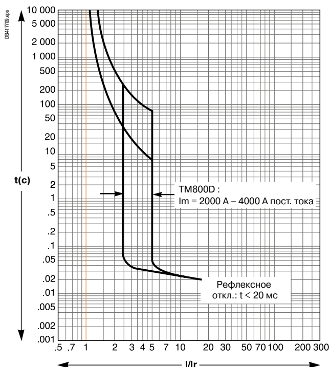
TM-DC 800
