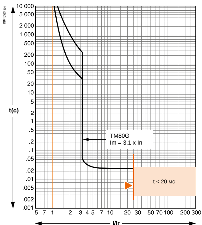
TMG80
