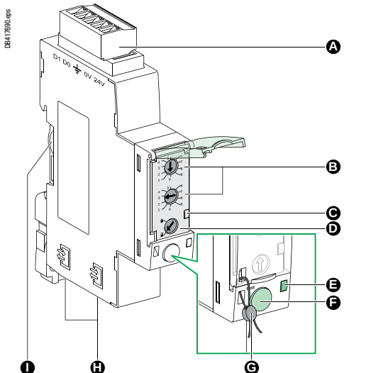
Модуль коммуникационного интерфейса Modbus. № по каталогу: TRV00210
