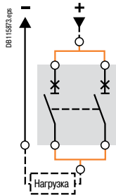
Выбор 3: Compact NSX100N 2P DC параллельно
