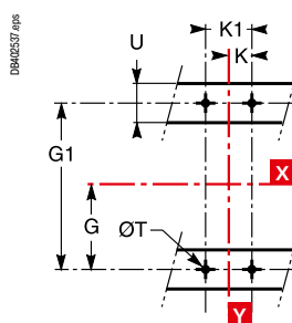
1 полюс
