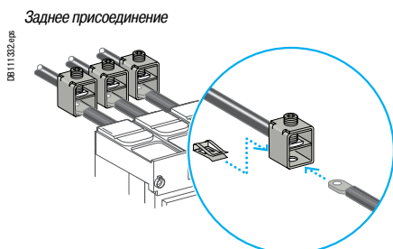
Подключение неизолированных кабелей к автоматическим выключателям NSX100 – 250 DC с помощью скобов
