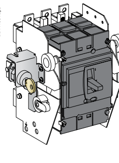
Блокировка мотор-редуктора с помощью встроенного или навесного замка
