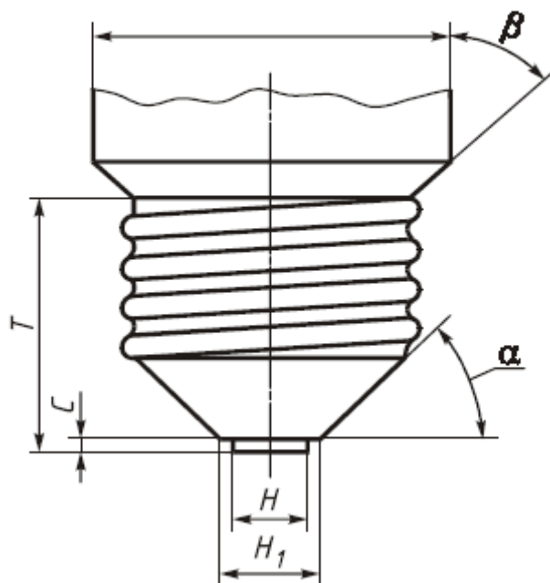
Испытательный цоколь E40
