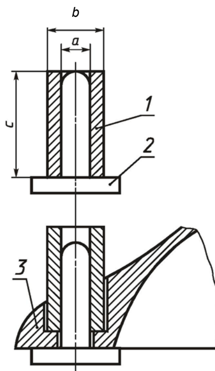
1 — втулка; 2 — штырь; 3 — фланец
