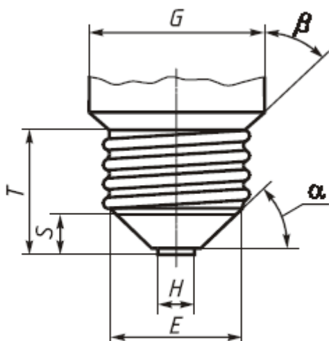
Испытательные цоколи E14 и E27
