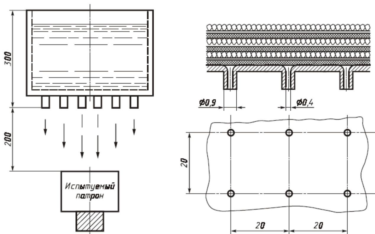
Рисунок 17 — Установка для проверки защиты от капель воды
